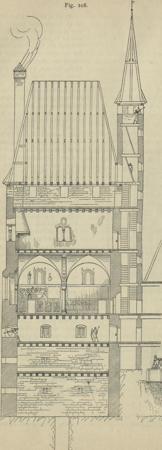
Thurm des Schlosses zu Friesach. — \frac{1}{250} n. Gr.
