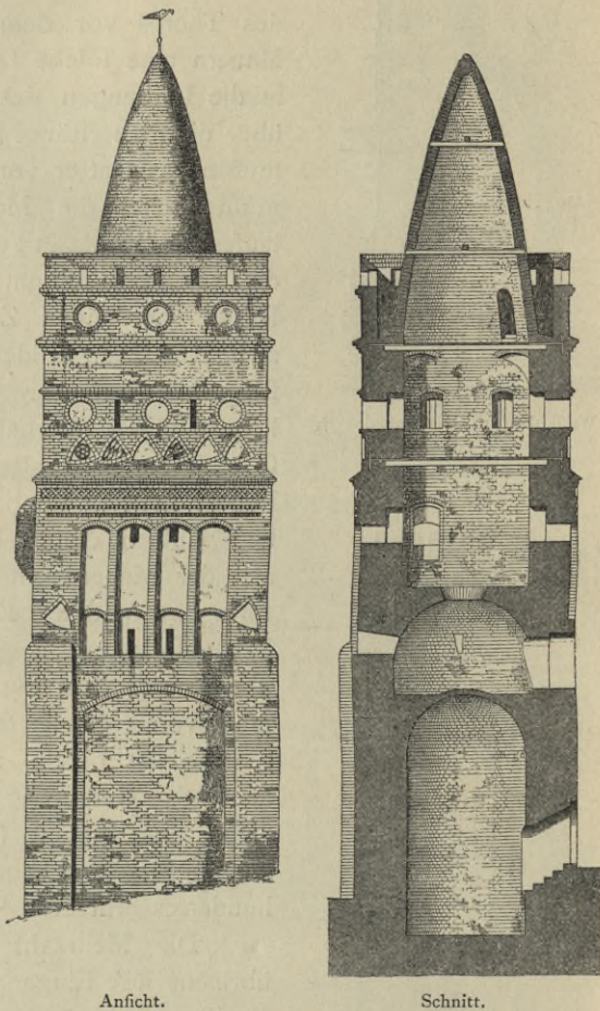
Ansicht.
