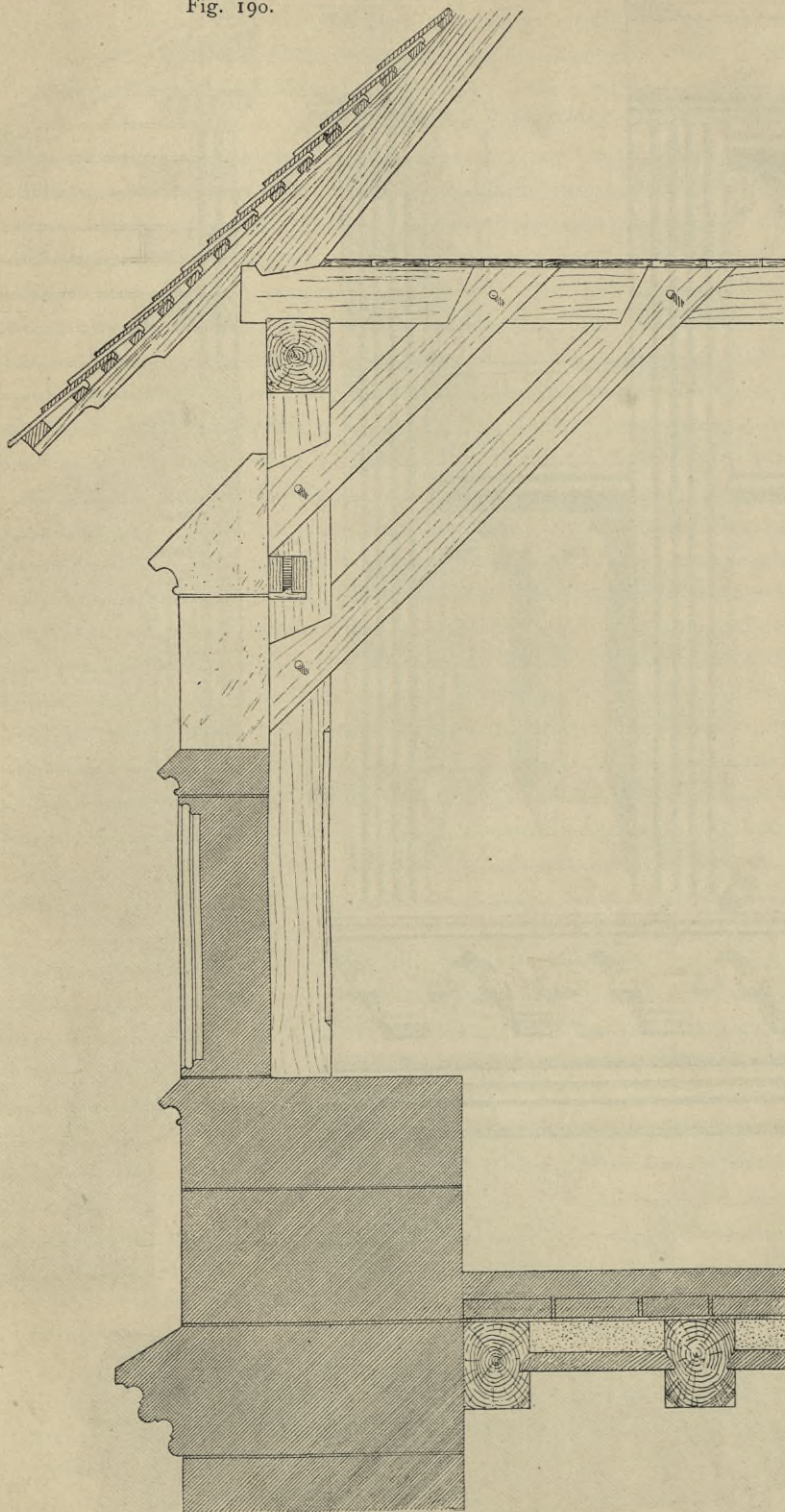
Zinnen des Schlüsselfelder'schen Stiftungshauses zu Nürnberg. — \frac{1}{25} n. Gr. (Zugleich Querschnitt zu neben stehender Tafel.)
