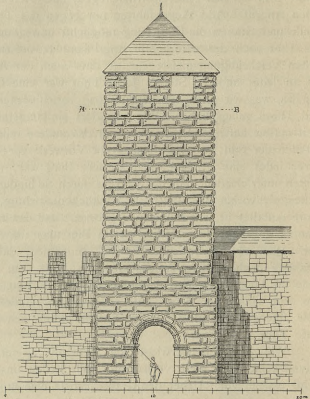
Thorthurm der Salzburg.
