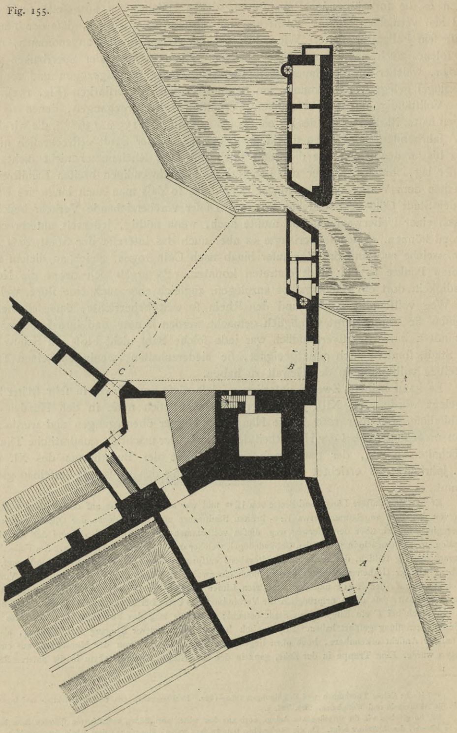
Bayen-Thor zu Cöln mit Vorwerken 200 ).
