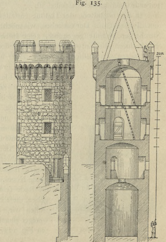
Cuniberts -Thürmchen zu Cöln 185 ).
