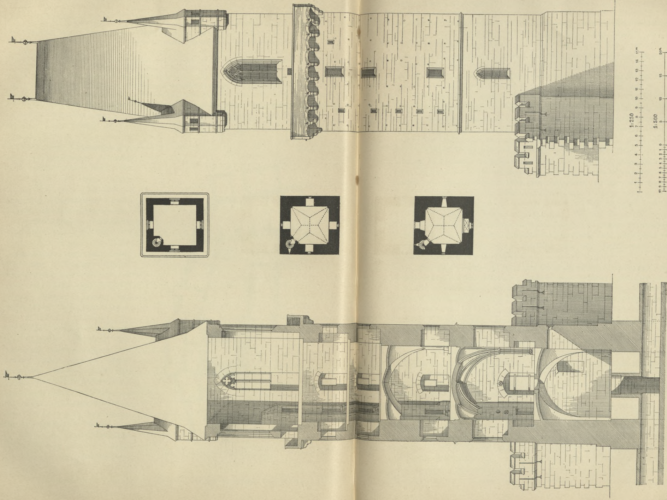
Thurm zu Perchtoldsdorf bei Wien.
