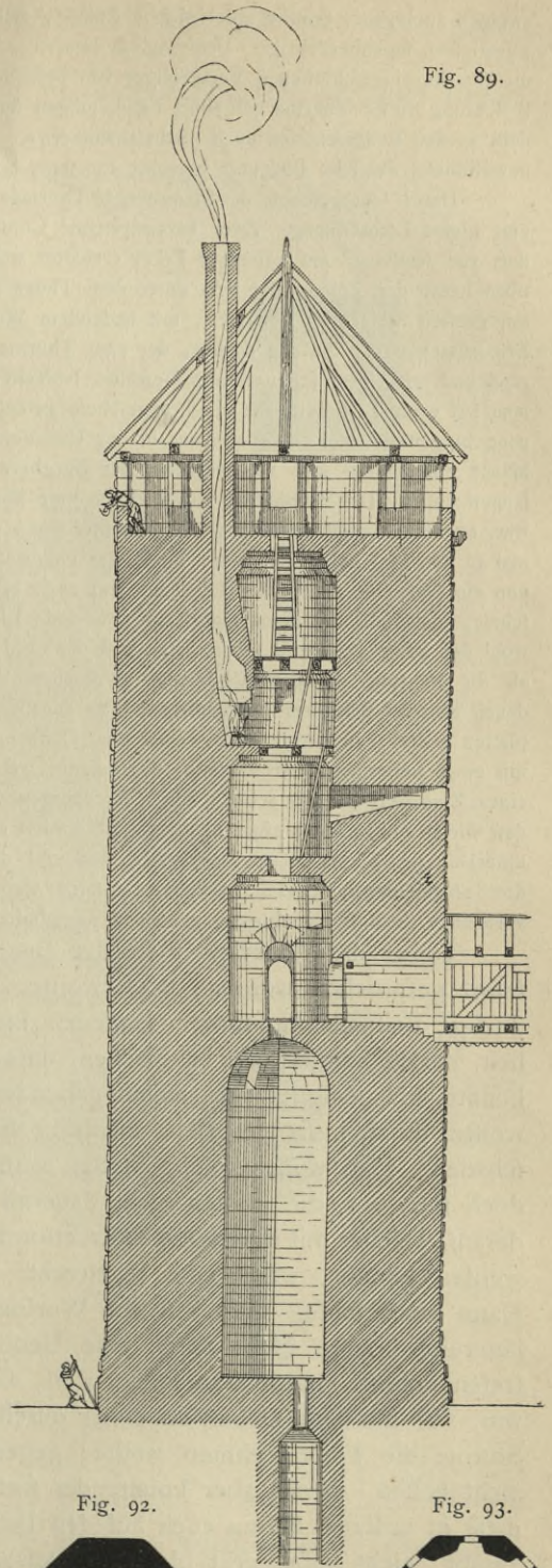
Querschnitt.
