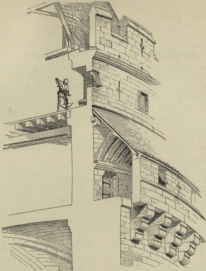
Thurmkrönung des Schloßes zu Pierrefonds 117) .
