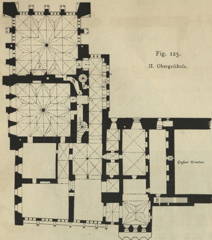
Grundriffe des Hauptgebäudes des neuen Schloßes der Marienburg 174 ).
