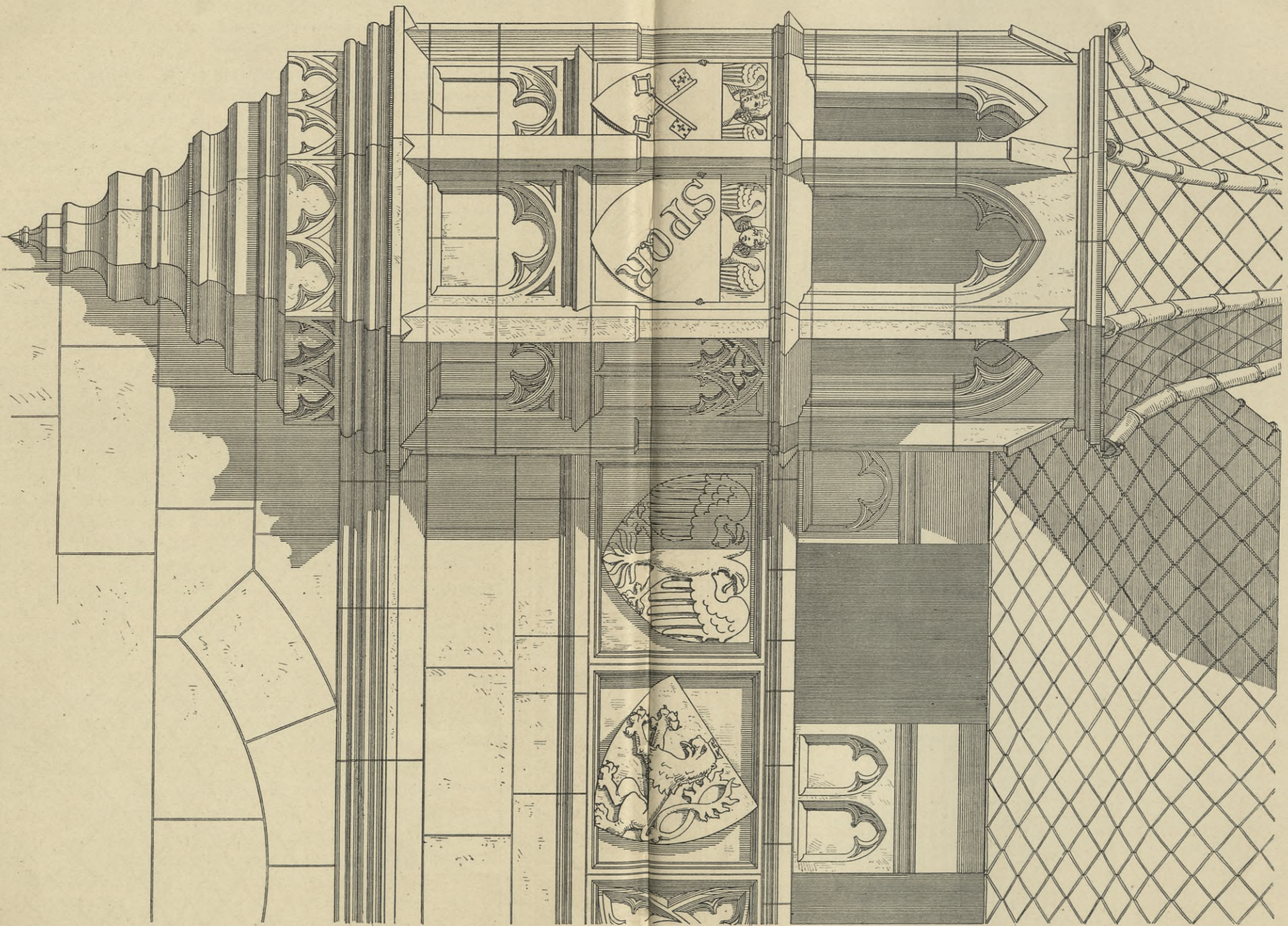
Vom Schlüßfeldern'schen Stiftungshaus zu Nürnberg.
