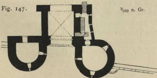
Grundriß.
