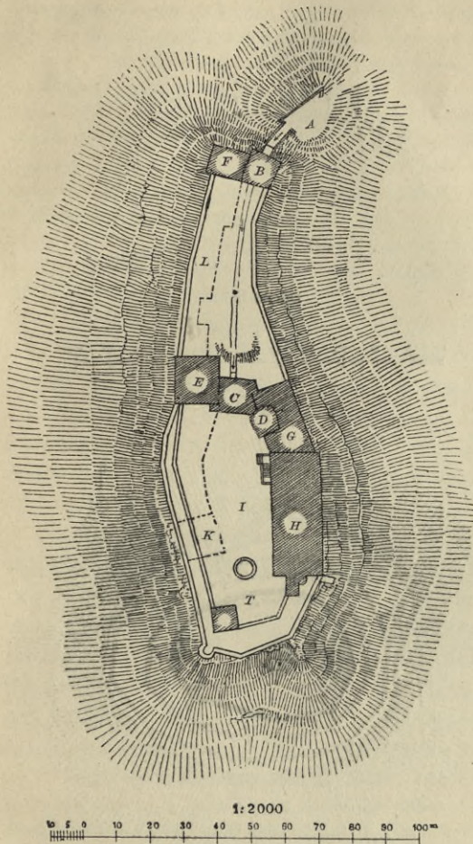
Grundriss der Wartburg 64) .
