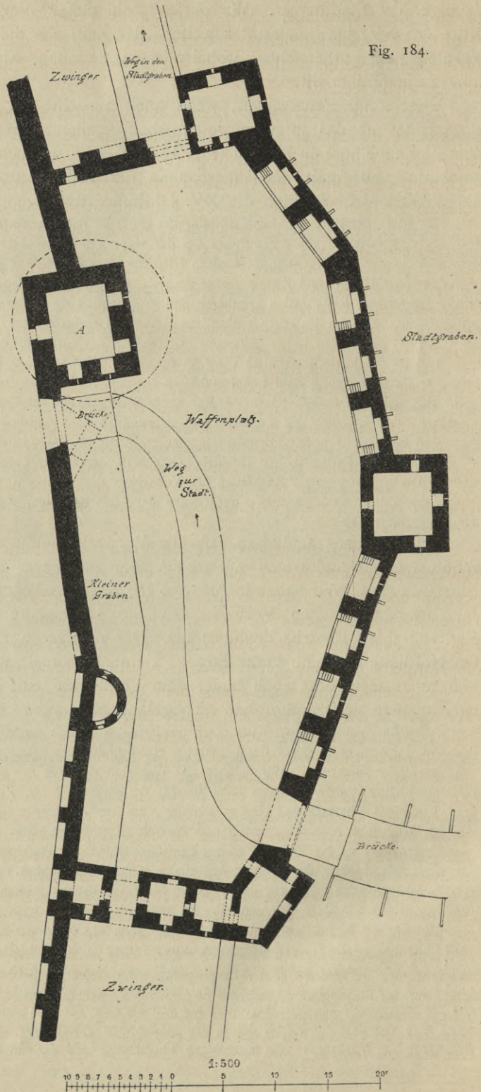
Vorwerk des Laufertthores zu Nürnberg.
