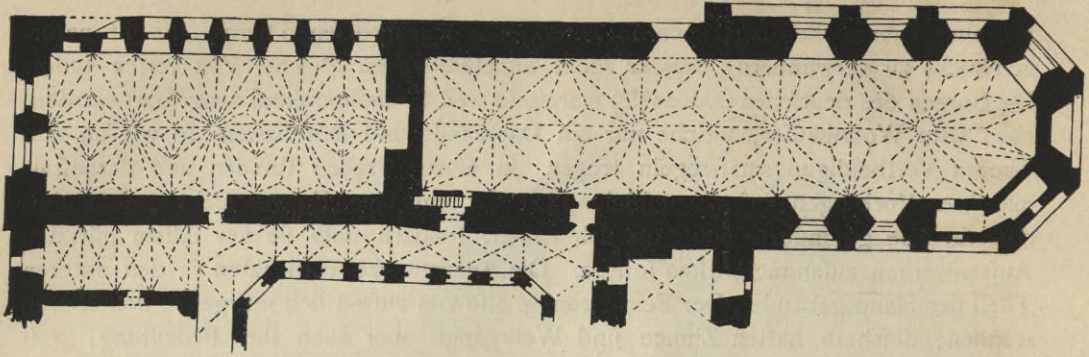
I. Obergefchofs.
