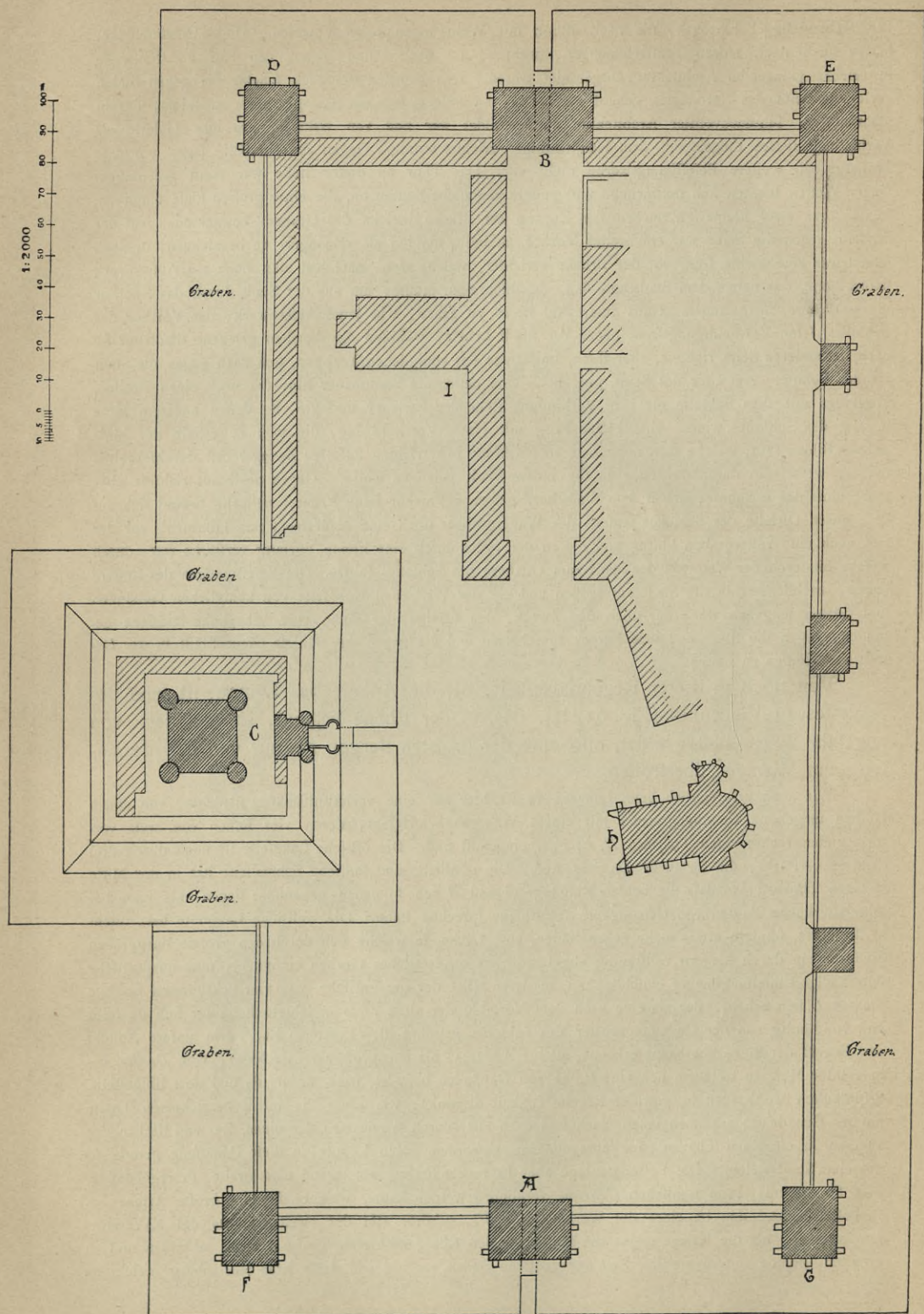
Grundriß des Schlosses zu Vincennes 113) .
