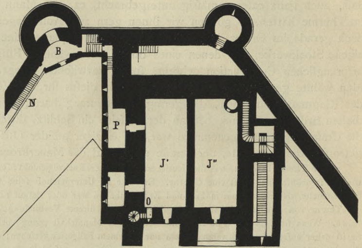
I. Obergeschoss.
