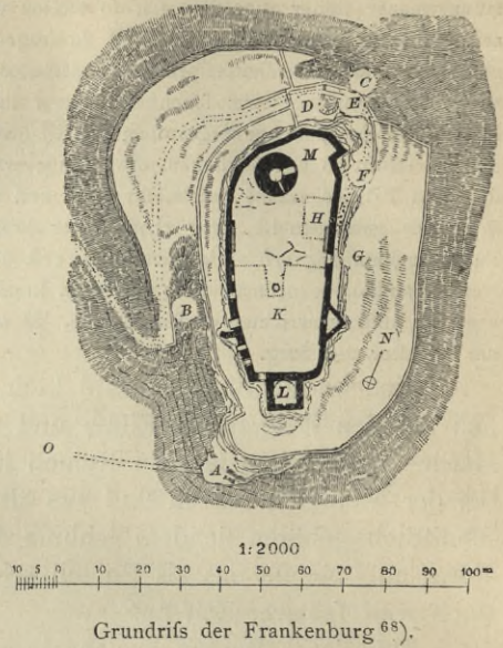
Grundriß der Frankenburg 65) .
