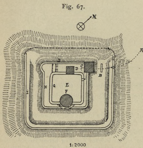
Grundriß der Burg Hugstein 118 ).
