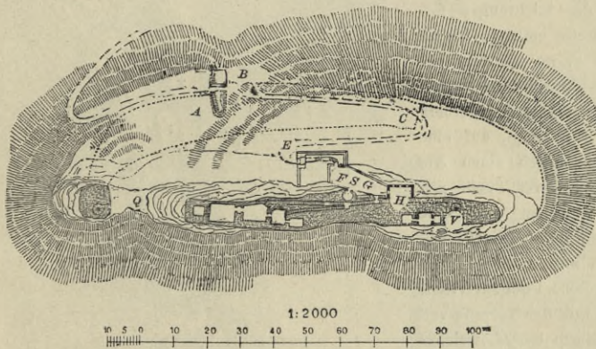
Grundriß der Burg Fleckenstein. — Ursprüngliche Anlage 76) .
