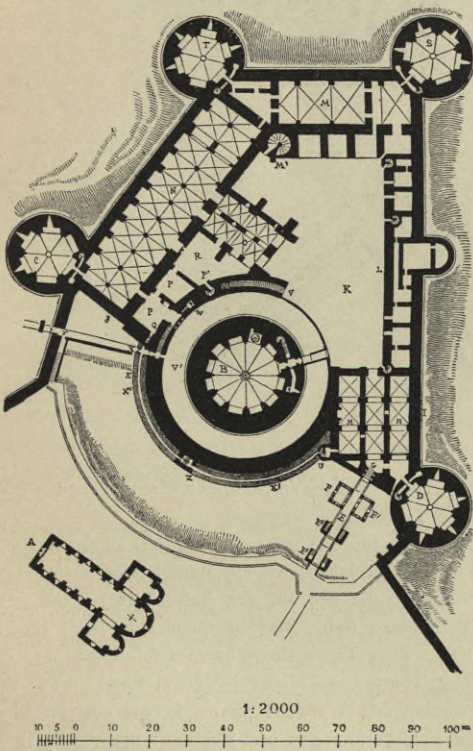
Grundriß des Schloßes zu Coucy 109) .
