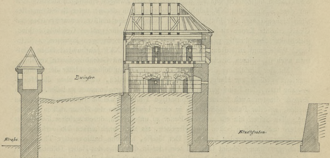
Durchschnitt
