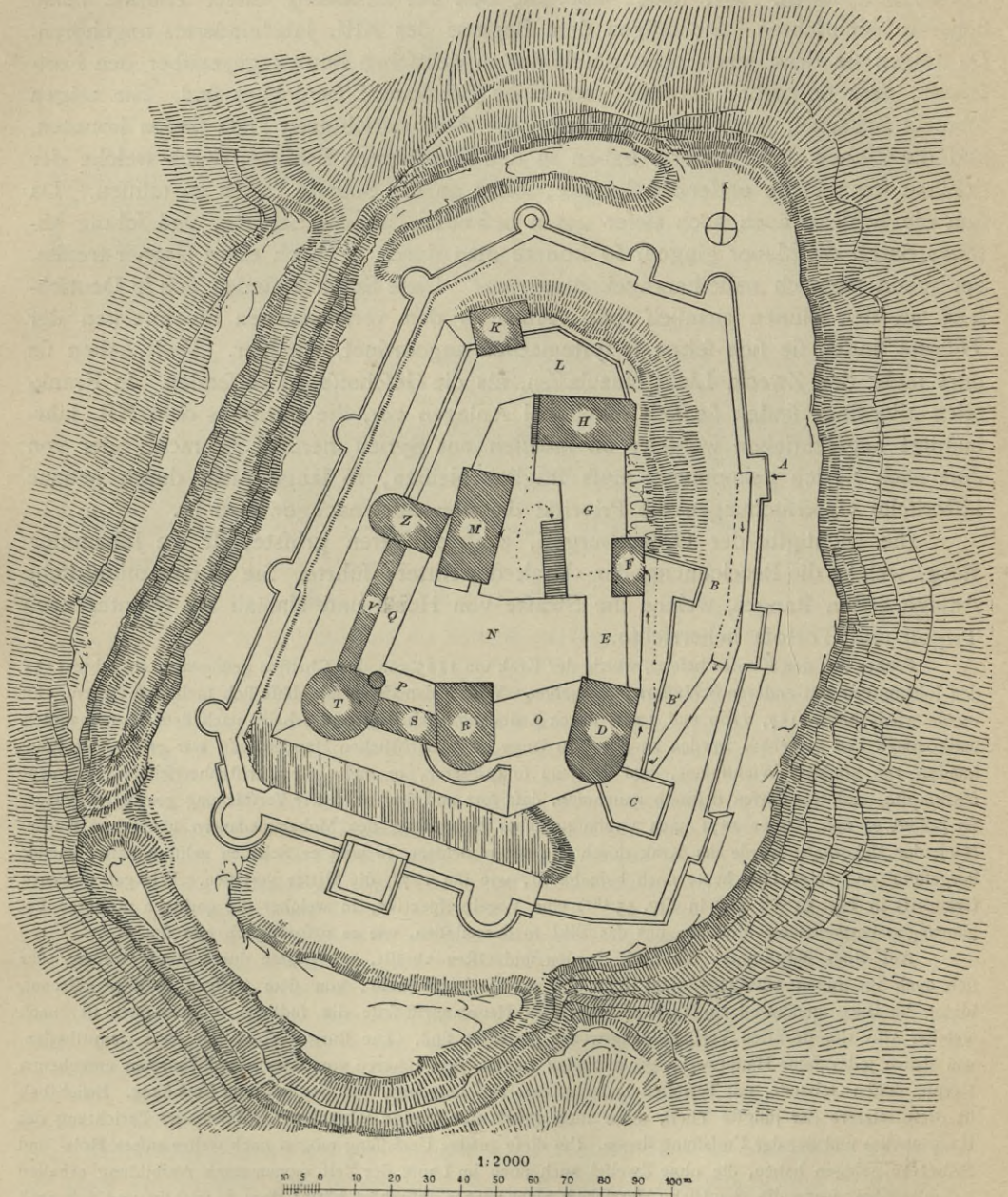
Grundriß des Johanniter-Schlosses »Krak der Ritter« 106) .
