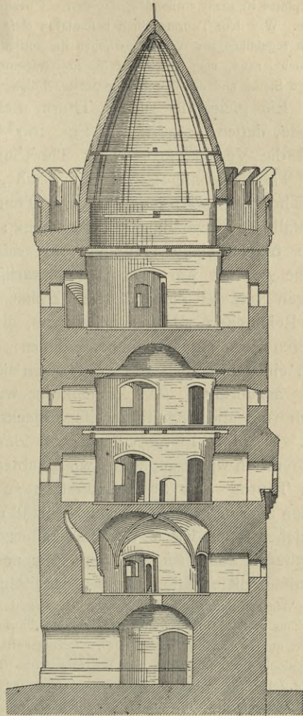
Schnitt.
