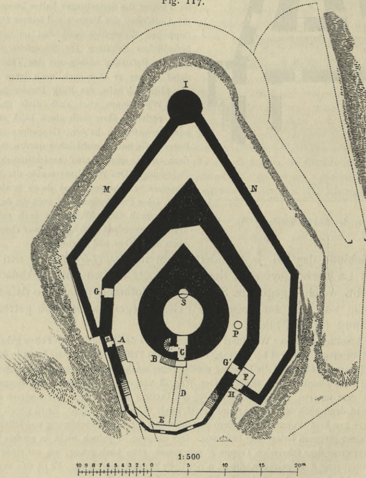
Thurm des Schlosses La Roche-Guyon 162 ).
