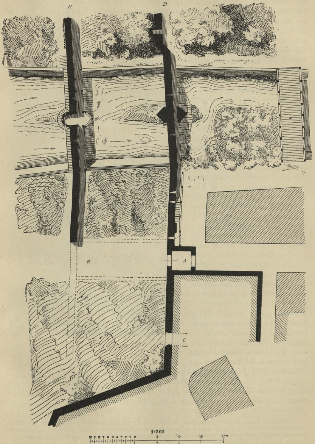
Grundriss des Steinthores zu Basel 202) .
