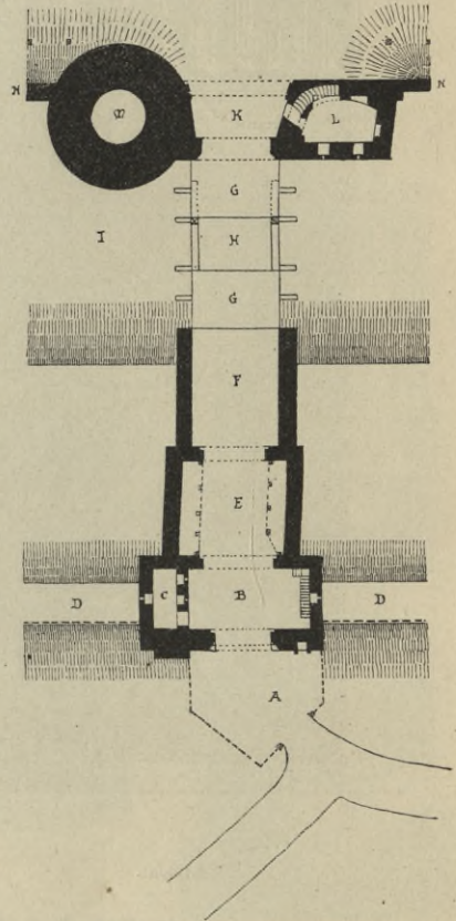
Grundrifs des Neustädter Thores zu Tangermünde 207) . — 1/500 n. Gr.
