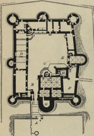
Grundriß des Schloßes zu Pierrefonds 114) .
