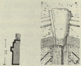
Fig. 332. Rosenthal, Turmtor, Profil und Fig. 333. Rosenthal, Turmtor, Profil und Schlußstein.
