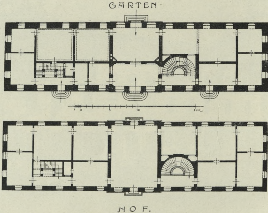
Fig. 266 und 267. Oberlichtenau, Schloß, Grundrisse des Erdgeschosses und des Obergeschosses.
