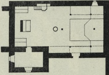
Fig. 297. Prietitz, alte Kirche, Grundriß.
