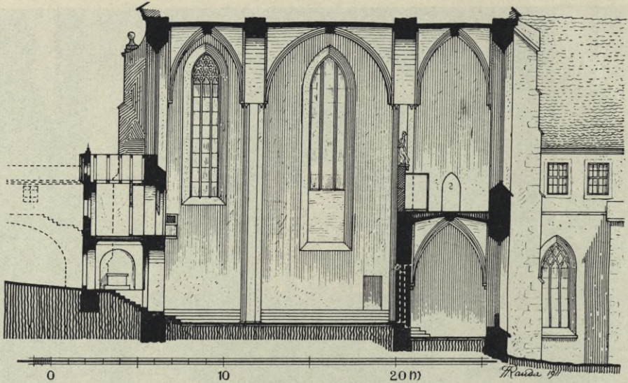
Fig. 144. Marienstein, Klosterkirche, Querschnitt.
