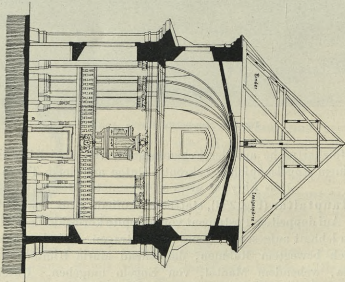
Fig. 252. Nebelschitz, Kirche, Querschnitt.
