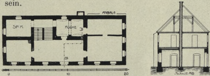
Fig. 33a und 33b. Elstra, Pfarre, Grundriß und Querschnitt.
