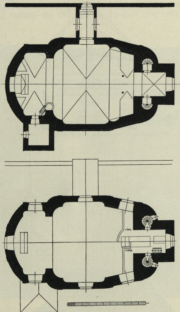
Fig. 287 u. 288. Ostro, Kirche, Grundrisse.
