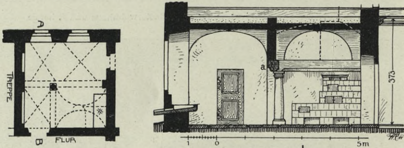
Fig. 323 u. 324. Röhrsdorf, Herrenhaus, alte Küche, Grundriß und Schnitt A-B.
