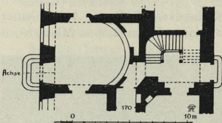
Fig. 302. Prietitz, Herrenhaus, Grundriß des Mittelteiles.
