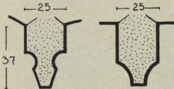
Fig. 152. Marienstern, Klosterkirche, Kreuz- und Scheiderippenprofil.
