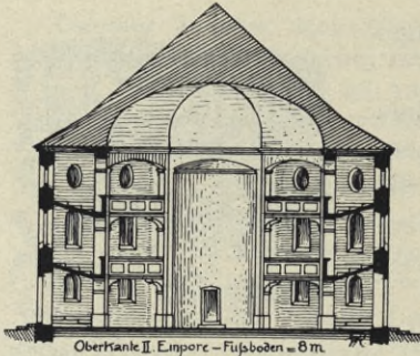
Fig. 140. Lichtenberg, Kirche, Querschnitt.
