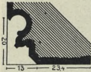
Fig. 160. Mariensterne, Klosterkirche, Profil des Nordtors.
