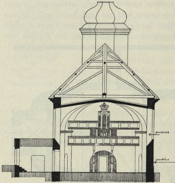
Fig. 289. Ostro, Kirche, Querschnitt.
