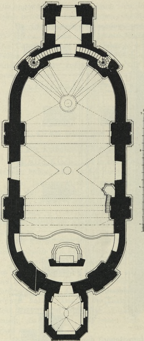
Fig. 248. Nebelschitz, Kirche, Grundriß.
