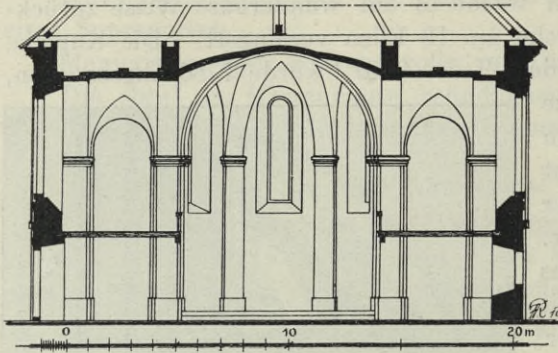
Fig. 331. Rosenthal, Kirche, Querschnitt.
