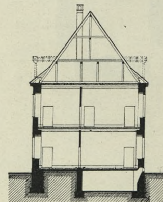
Fig. 272. Oberlichtenau, Schloß. Querschnitt.
