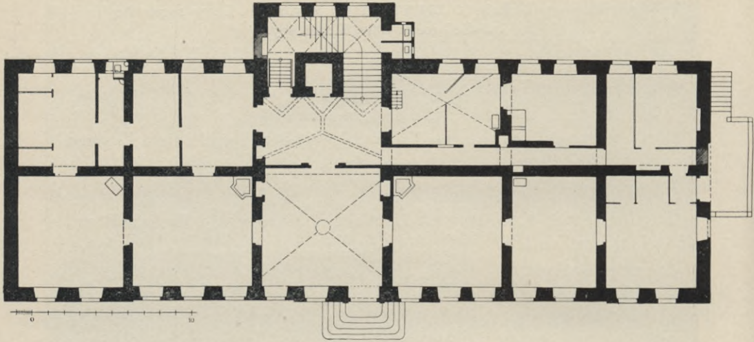
Fig. 225. Naunhof, Schloß, Grundriß.
