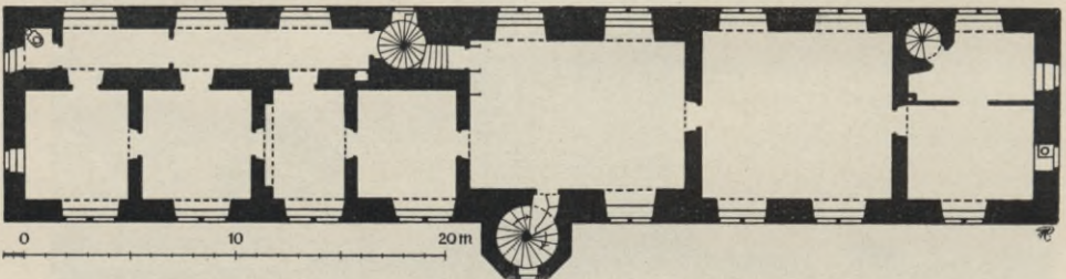
Fig. 579 Zottewitz, Schloß, Grundriß des 1. Obergeschosses.
