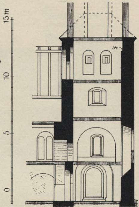
Fig. 242. Oberebersbach, Schnitt durch den Turm.
