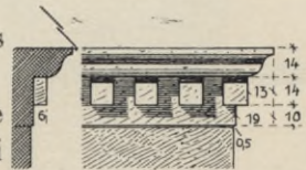
Fig. 371. Schönfeld, Schloß, Hauptgesims.
