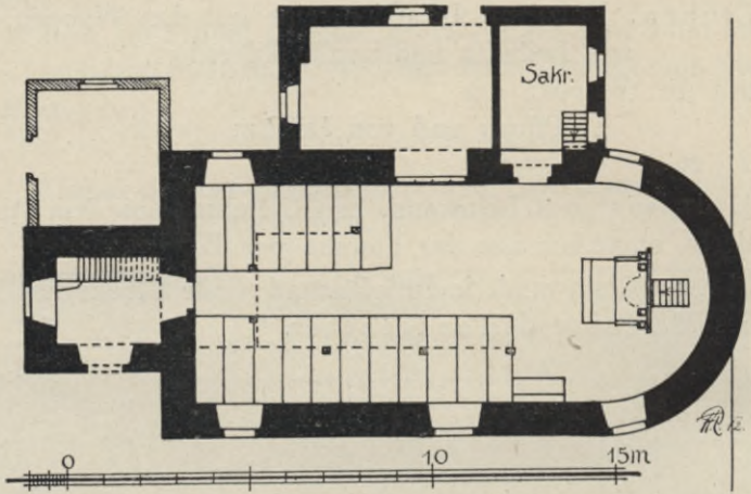
Fig. 589. Zschaiten, Kirche, Grundriß.
