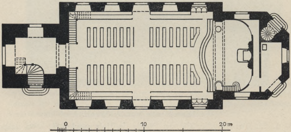
Fig. 259. Pausitz, Entwurf zur Kirche, Grundriß des Erdgeschosses.
