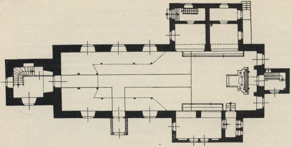
Fig. 106. Gröba, Kirche. Grundriß.
