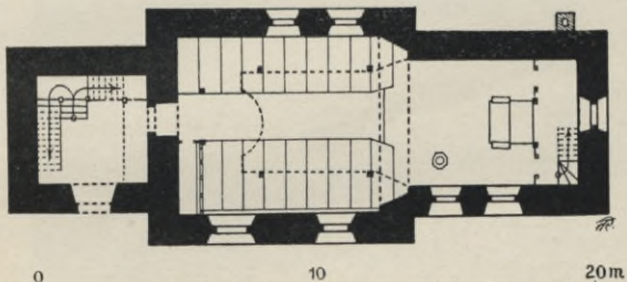
Fig. 100. Görzig, Kirche, Grundriß.
