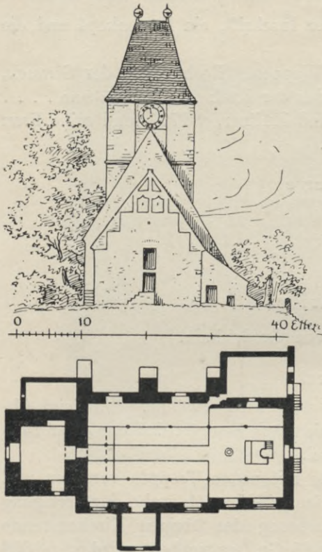
Fig. 514 und 515. Wantewitz, alte Kirche, Grundriß und Ansicht.
