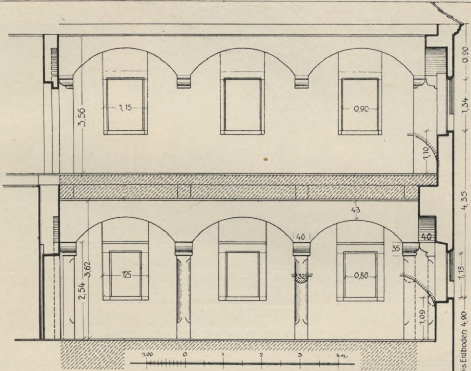
Fig. 381. Schönfeld, kleines Schloß, Teilschnitt.
