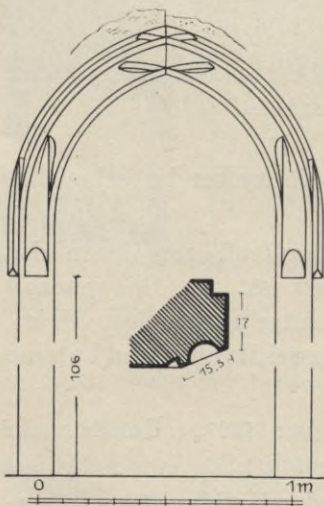
Fig. 442. Spansberg, Kirche, Sakristeithür.
