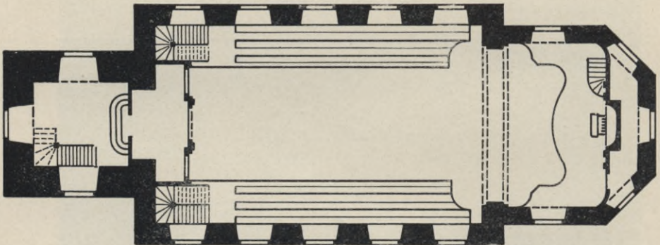
Fig. 258. Pausitz, Entwurf zur Kirche, Grundriß der Empore.
