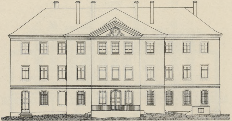
Fig. 556. Zabeltitz, Palais, Ansicht vom Garten, jetziger Zustand.
