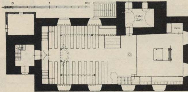
Fig. 55. Dobra-Kirche, Grundriß.
