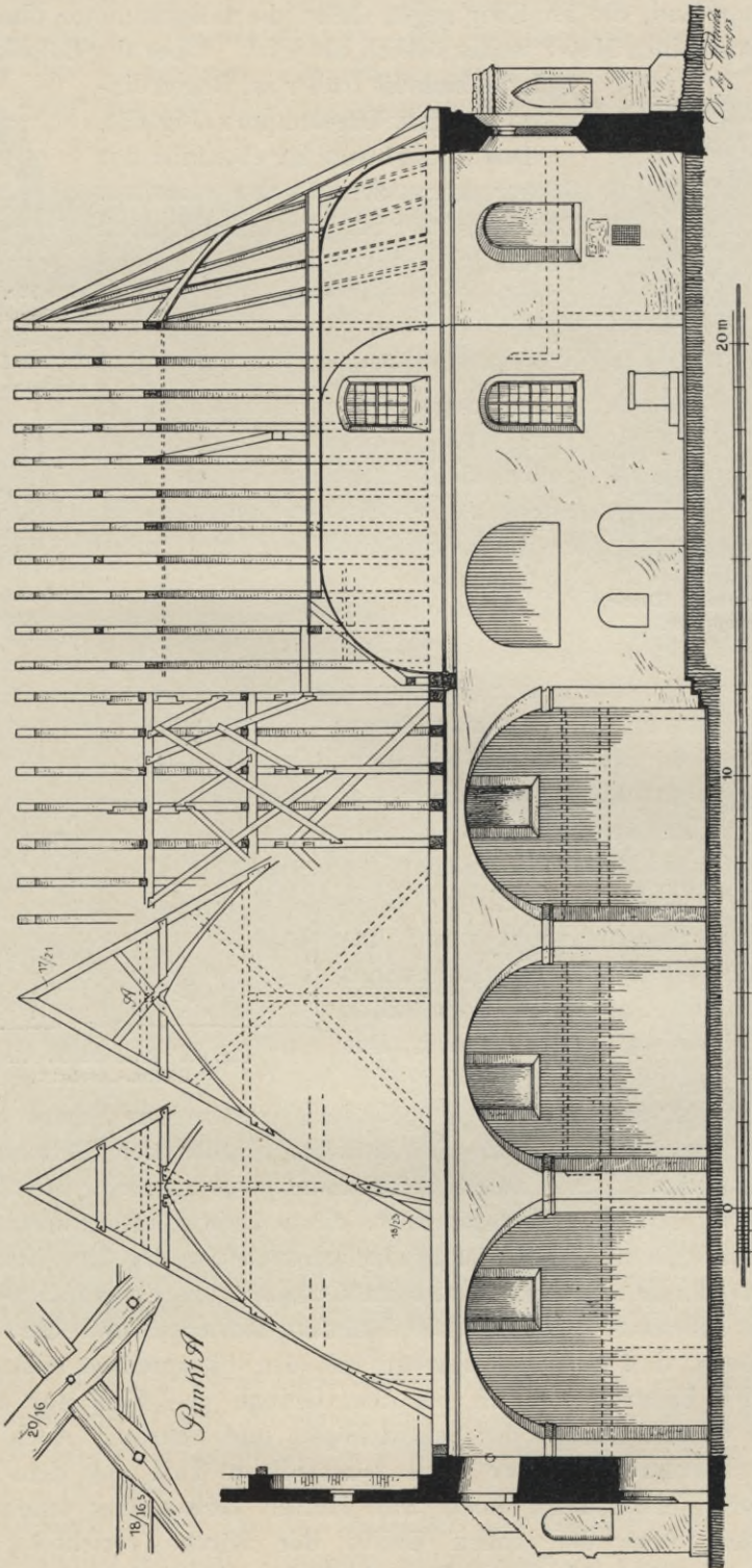
Fig. 61. Frauenhain, Kirche, Längsschnitt mit Chorddach.
