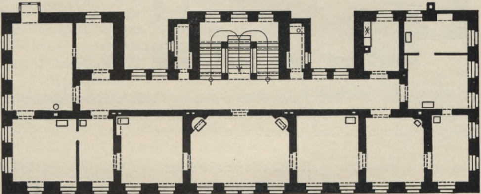
Fig. 54. Dallwitz, Herrenhaus, Grundriß des Obergeschosses.]
