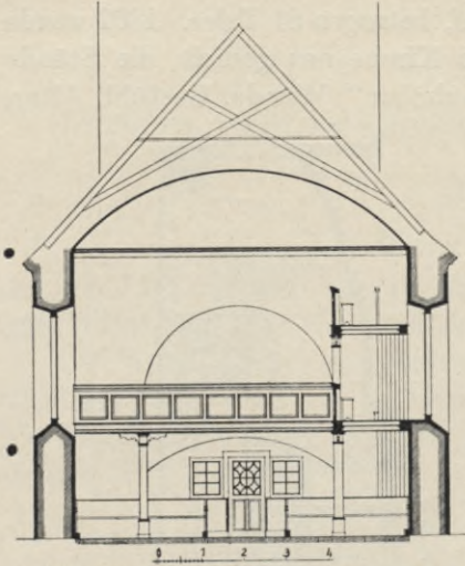
Fig. 340. Sacka, Kirche, Querschnitt.
