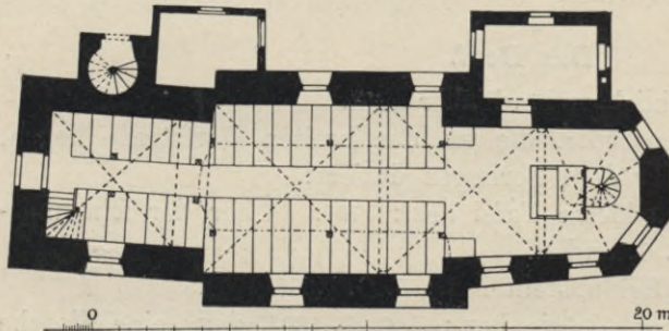
Fig. 182. Lichtensee, alte Kirche, Grundriß.
