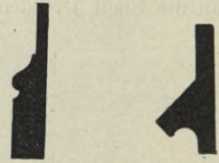
Fig. 46. Sockelprofil. Fig. 47. Gurtgesims.
