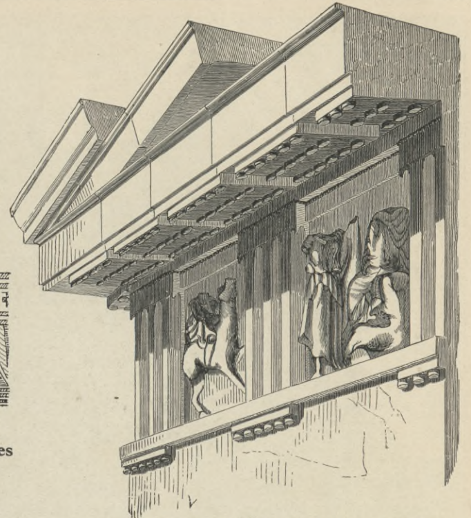
9. Dorischer Fries und Kranzgesims.
