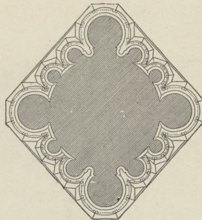
5. Grundriß eines Bündelpfeilers.
