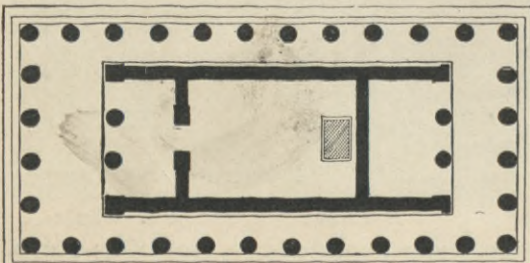
4. Tempel in Rhamnus. Grundriß.
