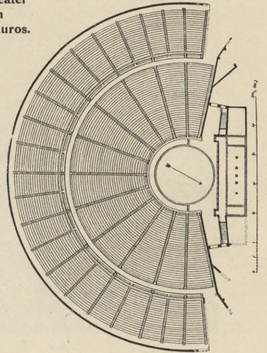
2. Grundriß des Theaters in Epidauros.
