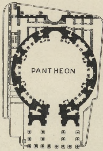
2. Pantheon in Rom. Grundriß.
