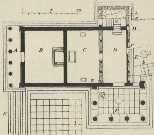
2. Erechtheion. Grundriß.
