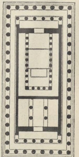
3. Parthenon. Grundriß.
