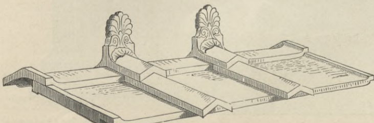
3. Firstziegel von Rhamnus.
