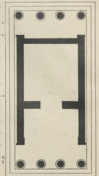
6. Tempel am Ilissos. Grundriß.
