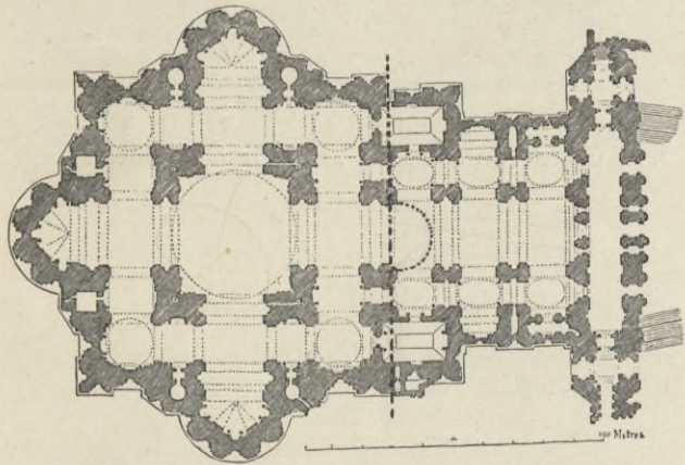
2. St. Peter in Rom. Grundriß.
