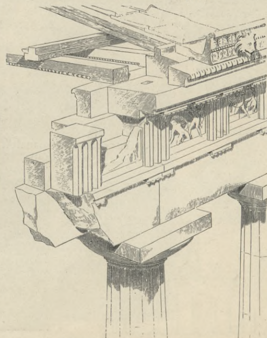
8. Dorische Deckenbildung.
