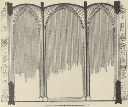
1. S. Maria zur Wiese in Soest. Querschnitt einer Hallenkirche.
