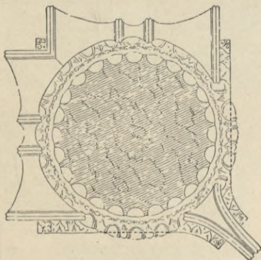
7. Grundriß des ionischen Eckkapitells.
