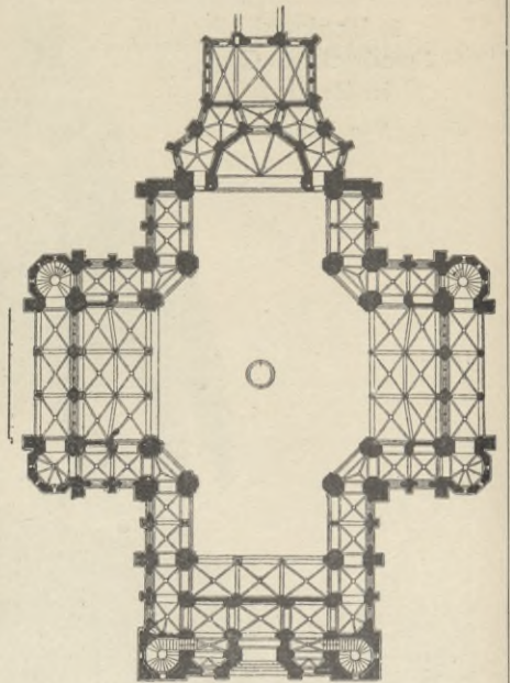
3. Die Kreuzkirche in Berlin. Von Otzen. Grundriß.
