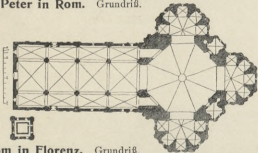
4. Der Dom in Florenz. Grundriß.
