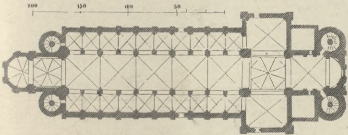
2. Dom zu Worms. Grundriß.
