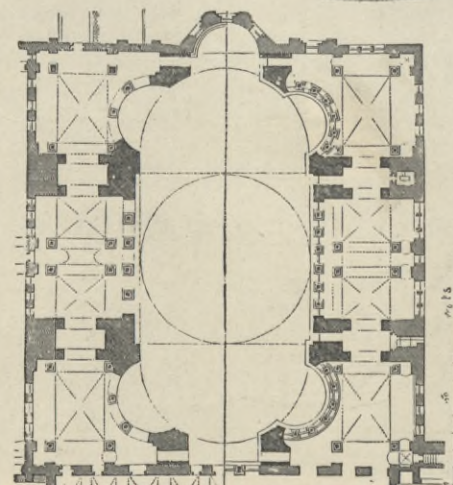
7. Sophienkirche in Konstantinopel. Grundriß.
