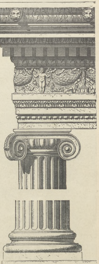
8. Römisch-ionische Ordnung. Eckkapitell vom sogen. Tempel der Fortuna virilis in Rom.
