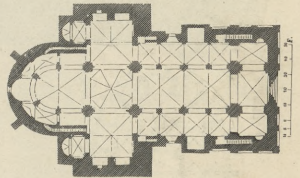
4. Dom zu Limburg a. d. Lahn. Grundriß.
