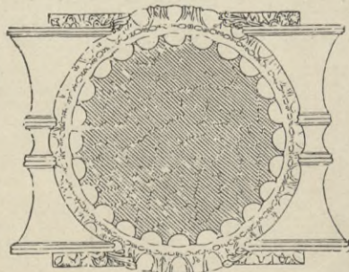
5. Grundriß des normalen ionischen Kapitells.
