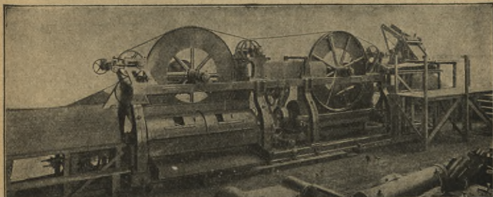
Entspinnungsmaschine „Victor“. Aus Clafey, Rohstoffe der Textilindustrie.
