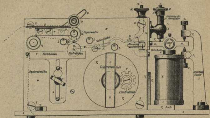
Morjsepparat. Aus Hamacher, Telegraphie und Telephonie.
