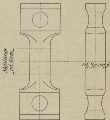
Versuchskörper nach Bauschinger
