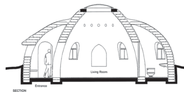
Il. 3. Przekrój przez konstrukcję struktury Sandbag Shelter, źródło: http://www.earthbagbuilding.com/projects/sandbagshelters.htm , dostęp: 22.11.2017 Ill. 3. Section of Sandbag Shelter construction, source: http://www.earthbagbuilding.com/projects/sandbagshelters.htm , access: 22.11.2017
