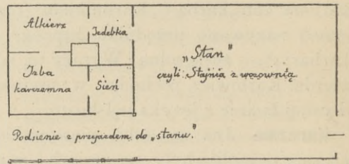
Fig. 2. Plan karczmy polskiej typu drugiego.
