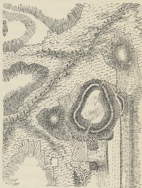
Plan topograficzny grodziska z epoki piastowskiej pod Tykocinem.
