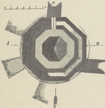
Przekrój poziomy baszty zamkowej w Rawie.
