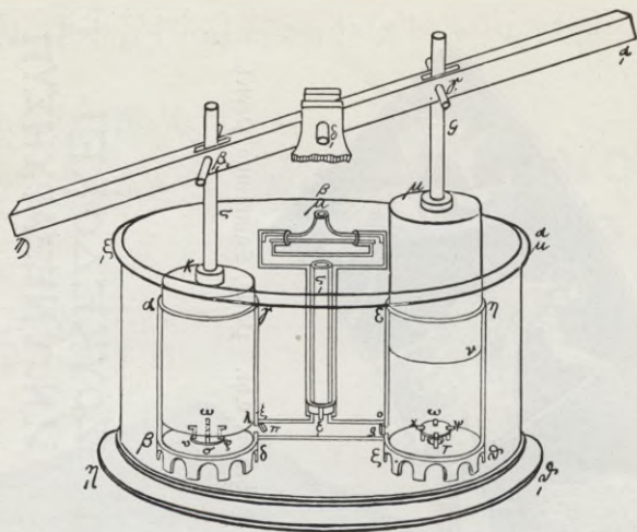
125. Feuerspritze. Nach Heron.
