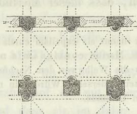
Dom zu Mainz.
