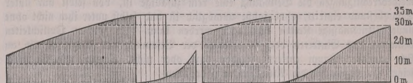
Vertikalschnitt in der Richtung A B.
