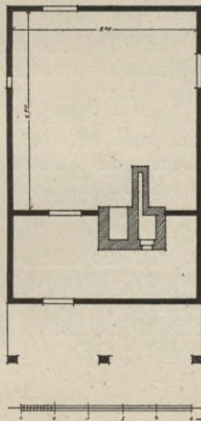
Abb. 4. Haus in Lesno, Kreis Konitz
