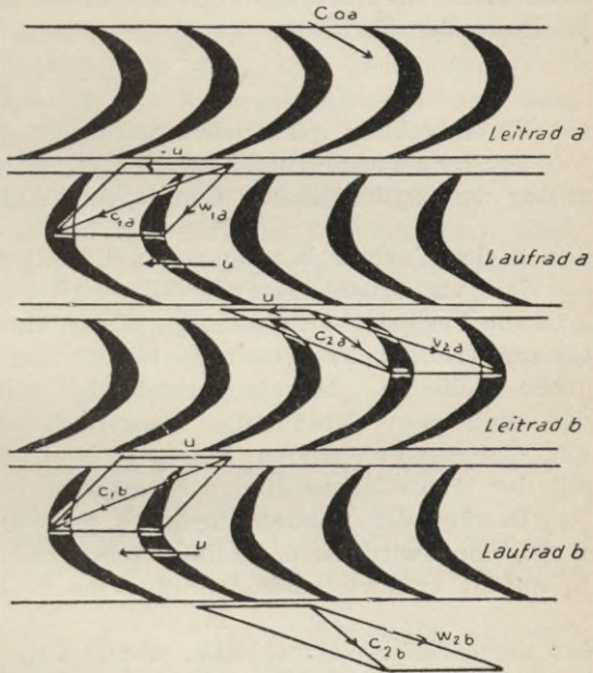
Fig. 28. Schaufelanordnung der Parsons-Turbine.
