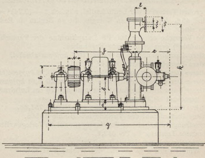
Konstruktionszeichnung (Aufriß) zur Tabelle 6.
