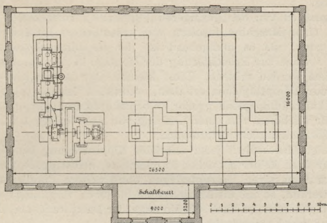
Fig. 41a. Abmessungen für den Platzbedarf von drei Kolbendampfmaschinen von je 600 PS.
