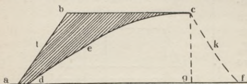
Fig. 20. Entropie-Temperaturdiagramm einer Maschine ohne Expansion.
