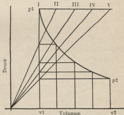
Fig. 4. Isothermische Expansionskurve.
