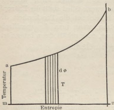
Fig. 14. Entropie-Temperaturdiagramm.
