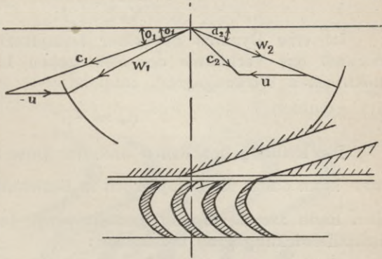
Fig. 27. Graphische Berechnung der Ein- und Austrittsgeschwindigkeit strömenden Dampfes.
