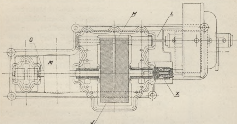
Fig. 32. Ansicht von oben und teilweiser Horizontalschnitt durch die Lagerung der Übersetzung einer 30 pferdigen de Laval-Turbine.
