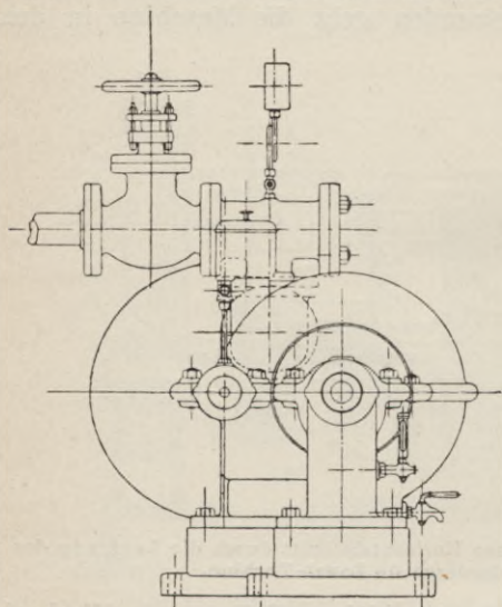
Fig. 33. Seitenansicht einer 30 pferdigen de Laval-Turbine.
