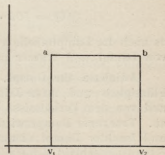
Fig. 13. Diagramm einer isothermischen Expansion.
