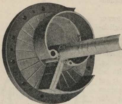
Fig. 79. Ansicht der Kraftwelle mit den Steuerungsteilen, der linken Expansionszylinderwand, dem Dichtungs- und Anlaufkammringe, sowie der Dichtungszunge mit ihrem verdeckten Führungsringe einer Patschke-Rotationsdampfmaschine.
