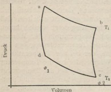
Fig. 11. Diagramm eines Kreisprozesses mit zwei isothermischen und zwei adiabatischen Vorgängen.
