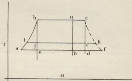
Fig. 19. Entropie-Temperaturdiagramm einer Idealmaschine ohne Kompression, jedoch mit völliger Expansion.
