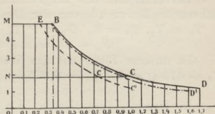
Fig. 17. Druck-Volumenkurve für gesättigten Dampf.
