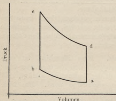
Fig. 7. Indikatordiagramm nach Stirlings Kreisprozeß.
