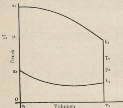
Fig. 9. Indikatordiagramm einer nicht umkehrbaren Zustandsänderung.
