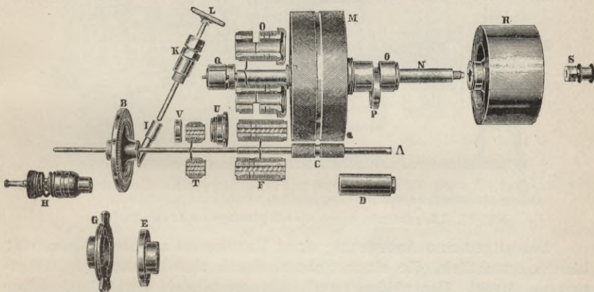
Fig. 30. Bestandteile einer de Laval-Maschine.
