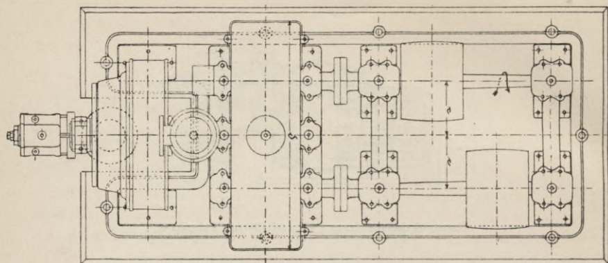
Konstruktionszeichnung (Grundriß) zur Tabelle 7.
