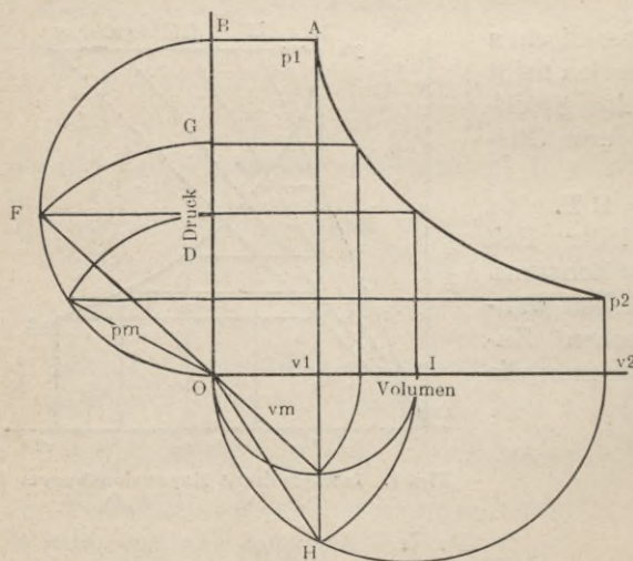
Fig. 5. Polytropische Expansionskurve.
