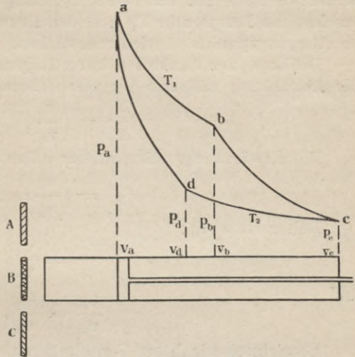
Fig. 6. Indikatordiagramm nach Carnots Kreisprozeß.
