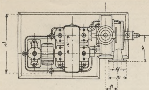
Konstruktionszeichnung (Grundriß) zur Tabelle 6.
