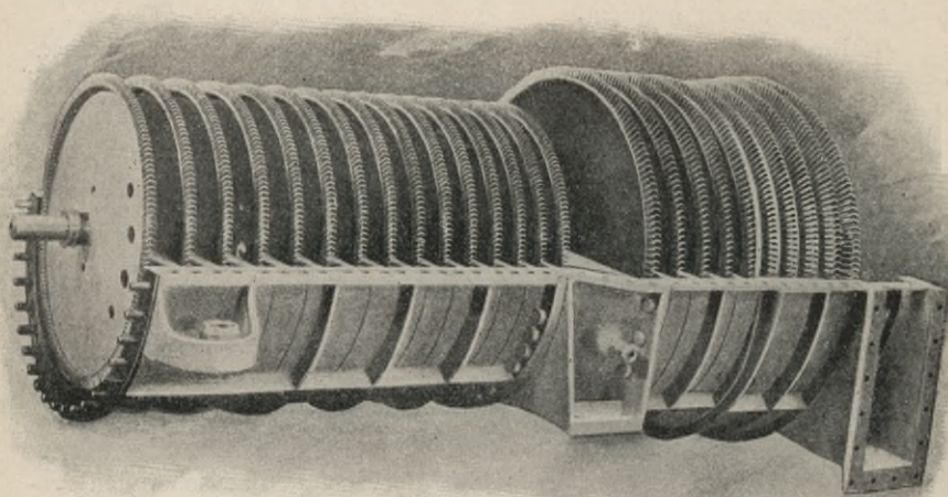
Fig. 56. Ansicht der Laufräder einer Rateau-Turbine, deren obere Gehäusehälfte entfernt ist.
