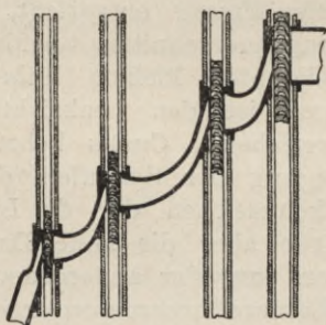
Fig. 46 und 47. Schnitte durch eine Curtis-Turbine.
