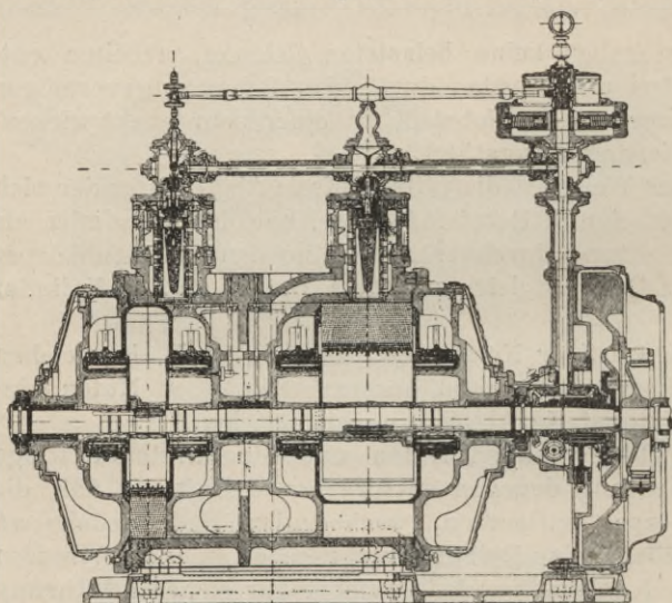
Fig. 77. Längsschnitt durch eine zweifache Expansions-Rotationsdampfmaschine von Patschke.
