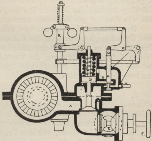
Fig. 40. Steuerungsschema einer Parsons-Turbine.
