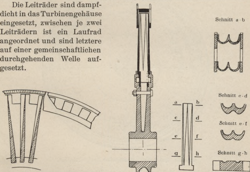
Fig. 62, 63, 64 und 65. Schnitte durch die Schaufel einer Zoelly-Turbine.
