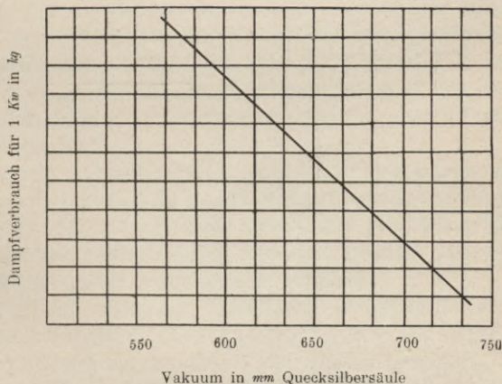
Fig. 55. Graphische Darstellung einer Untersuchung über die Abhängigkeit des Dampfverbrauches einer Curtis-Turbine vom Vakuum im Dampfraume.
