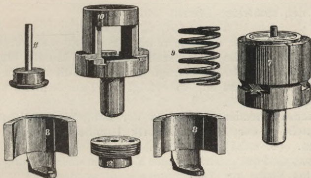
Fig. 38. Bestandteile des Reguliermechanismus der de Laval-Turbine.
