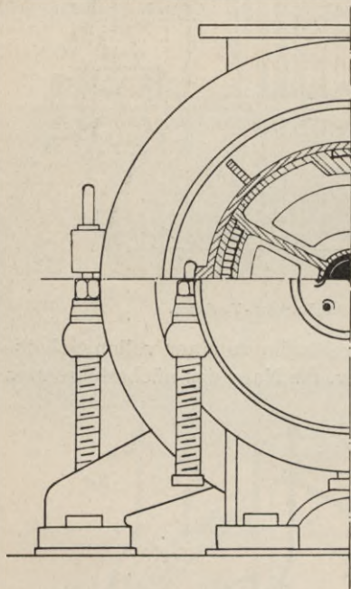
Fig. 60. Stirnansicht und teilweiser Querschnitt durch eine Rateau-Turbine.
