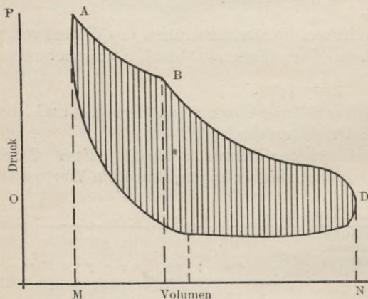
Fig. 1. Indikatordiagramm nach Watt.
