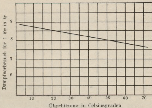
Fig. 54. Graphische Darstellung einer Untersuchung über die Abhängigkeit des Dampfverbrauches einer Curtis-Turbine von der Überhitzung des Dampfes.
