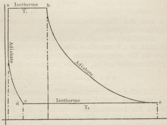
Fig. 22. Carnots Kreisprozeß mit Dampf durchgeführt.
