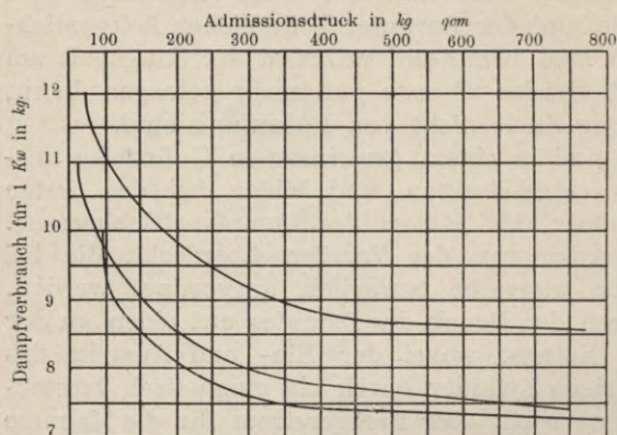
Fig. 52. Graphische Darstellung einer Untersuchung über den Dampfverbrauch einer Curtis-Turbine von 600 Kilowatt Leistung.
