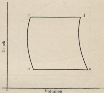
Fig. 8. Indikatordiagramm nach Ericsons Kreisprozeß.
