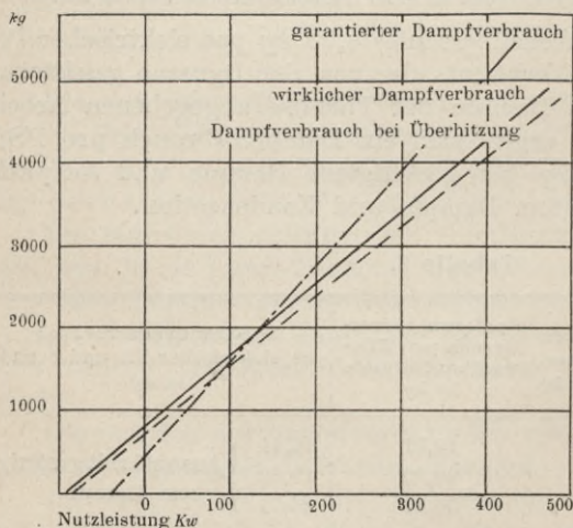
Fig. 43. Graphische Darstellung einer Untersuchung über den Dampfverbrauch an einer Parsons-Turbine von 600 P.S.
