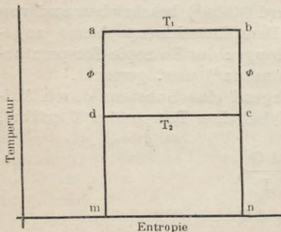
Fig. 15. Entropie-Temperaturdiagramm eines Kreisprozesses.
