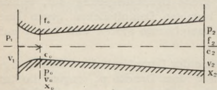
Fig. 26. Düsenenerweiterung.
