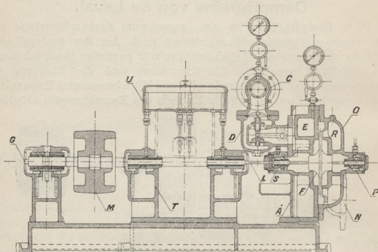
Fig. 31. Längsschnitt durch eine 30pferdige de Laval-Turbine.
