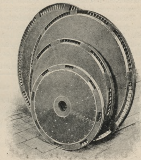
Fig. 61. Ansicht der Leiträder einer Rateau-Turbine.
