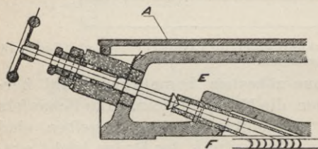
Fig. 36. Dampfdüsen-Querschnitt einer 30 pferdigen de Laval-Turbine.
