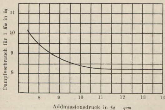
Fig. 53. Graphische Darstellung einer Untersuchung über die Abhängigkeit des Dampfverbrauches einer Curtis-Turbine von der Überhitzung des Dampfes.
