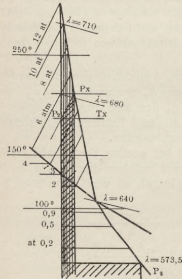
Fig. 29. Berechnung der Druckverteilung und Schaufelabmessung.
