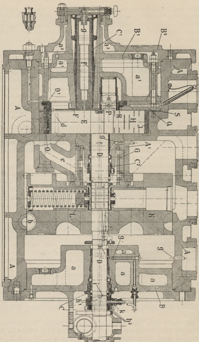
Fig. 76. Längsschnitt durch eine Versuchs-Rotationsdampfmaschine von Patschke.
