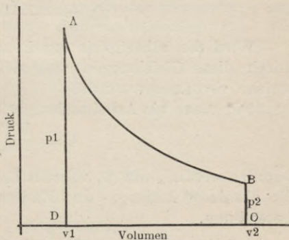
Fig. 2. Expansionskurve einer Arbeitsflüssigkeit.
