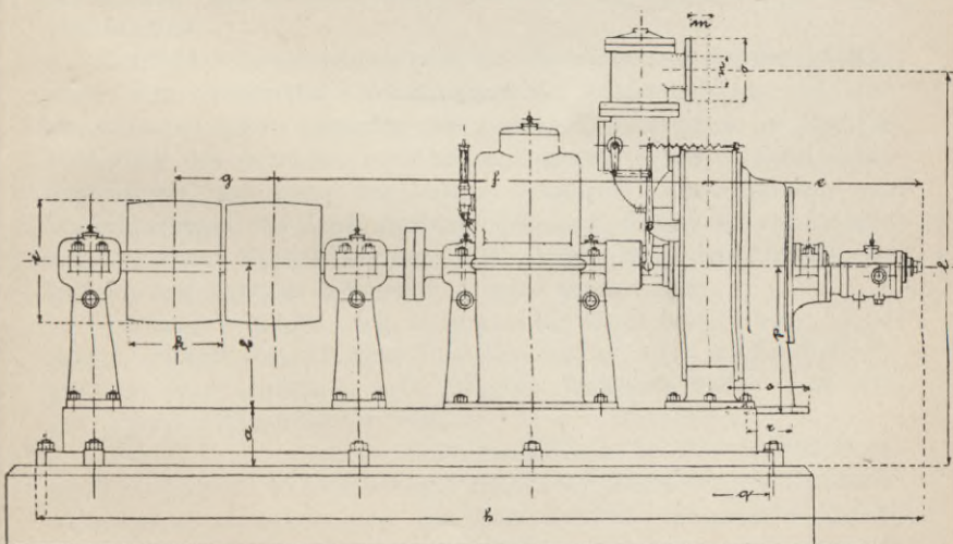
Konstruktionszeichnung (Aufriß) zur Tabelle 7.
