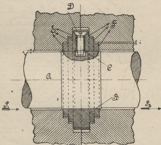
Fig. 80. Dichtungsring einer Patschke-Rotationsdampfmaschine.
