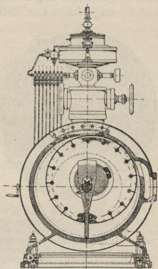
Fig. 78. Querschnitt durch eine zweifache Expansionsmaschine von Patschke.
