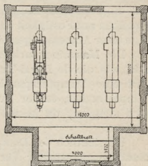
Fig. 41b. Abmessungen für den Platzbedarf von drei Parsonsturbinen von je 600 PS.
