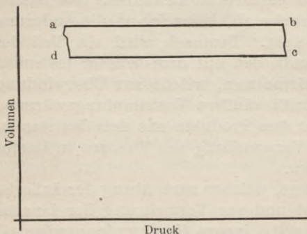
Fig. 12. Indikatordiagramm mit zwei Isothermen und zwei Adiabaten.
