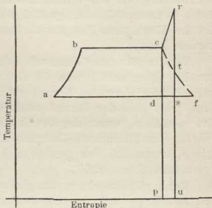
Fig. 21. Entropie-Temperaturdiagramm überhitzten Dampfes.
