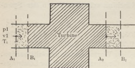
Fig. 23. Strömende Bewegung des Dampfes.
