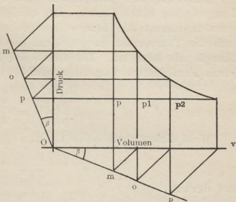
Fig 3. Adiabatische Expansionskurve.
