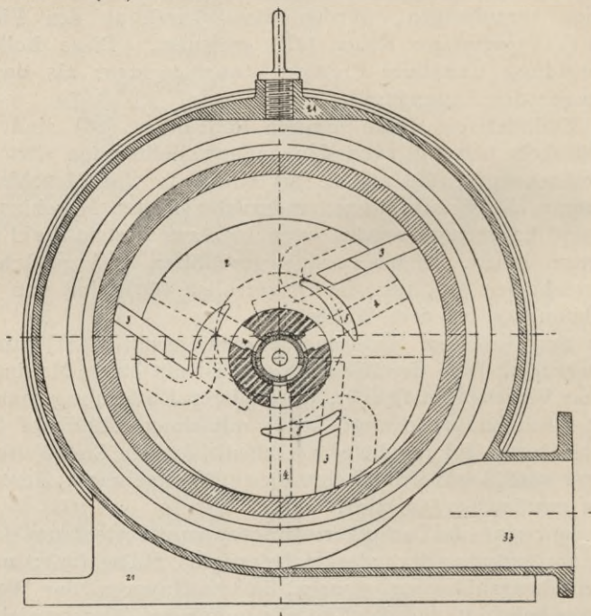
Fig. 73. Querschnitt durch eine Rotationsdampfmaschine von Hult.
