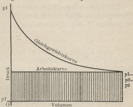
Fig. 10. Indikatordiagramm einer unvollkommenen Expansion.
