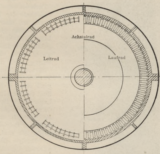
Fig. 67. Querschnitt durch eine Zoelly-Turbine.
