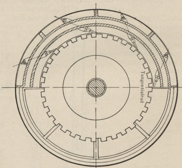
Fig. 66. Querschnitt durch eine Zoelly-Turbine.
