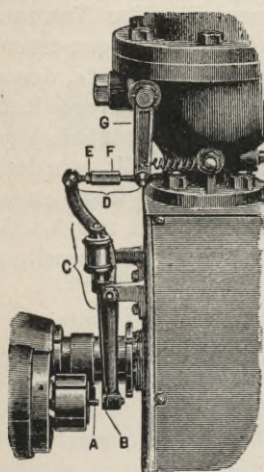
Fig. 37. Regulator der de Laval-Turbine.
