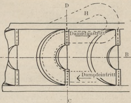
Fig. 69. Schaufelanordnung der Stumpf-Riedler-Turbine.
