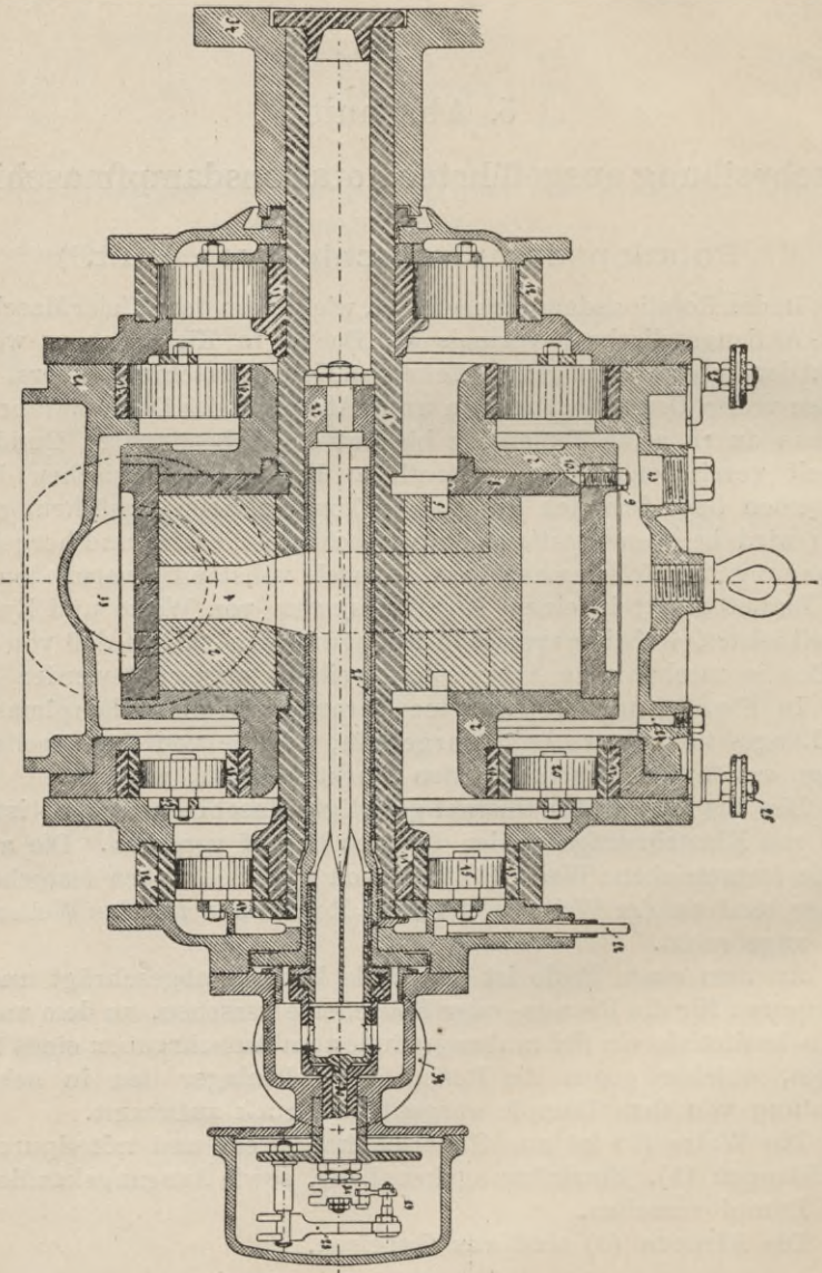
Fig. 72. Längsschnitt durch eine Rotationsdampfmaschine von Hult.
