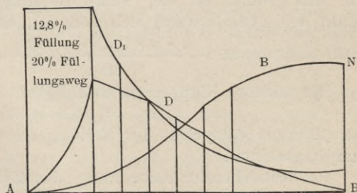
Fig. 74. Dampfdiagramm einer Rotationsdampfmaschine von Hult.
