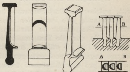
Fig. 35. Schaufeln in halber natürlicher Größe einer 300 pferdigen de Laval-Turbine und deren Befestigung.
