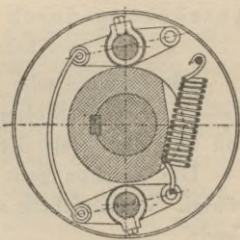
Fig. 151. Schnitt B-C.
