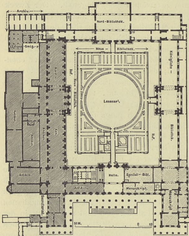
Grundriss des Britischen Museums zu London.
