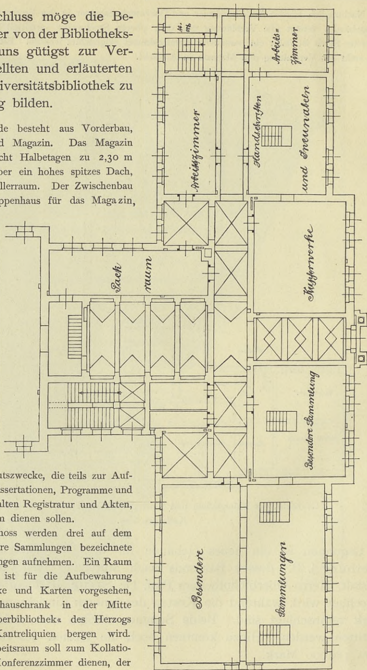
Grundriss der Könighchen und Universitätsbibliothek zu Königsberg. Erdgeschoss.
