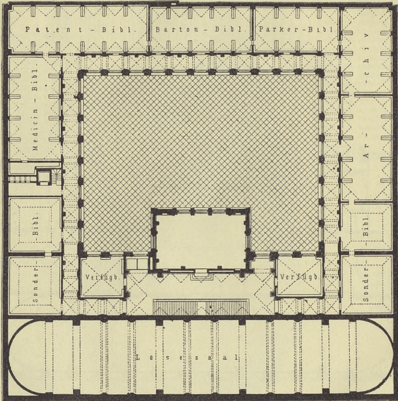
Zweites Obergeschoss der Oeffentlichen Bibliothek zu Boston.
