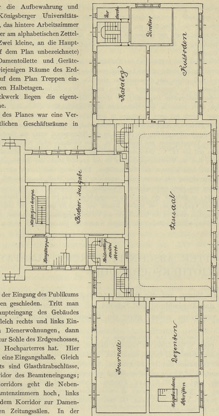
Grundriss der Königsberger und Universitätsbibliothek zu Königsberg. Erstes Stockwerk.
