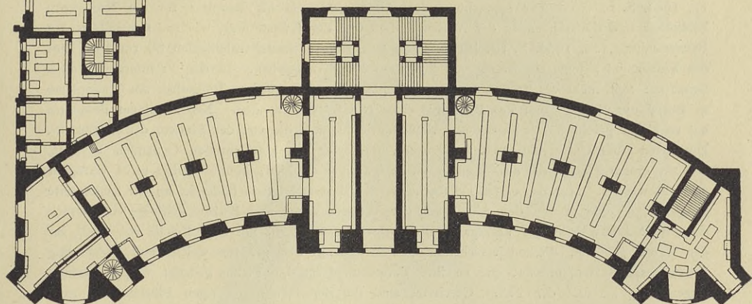
Grundriss der Königlichen Bibliothek zu Berlin. Obergeschoss.
