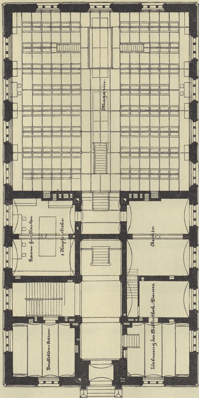
Grundriss der Königl. Universitätsbibliothek zu Kiel: Erdgeschoss.
