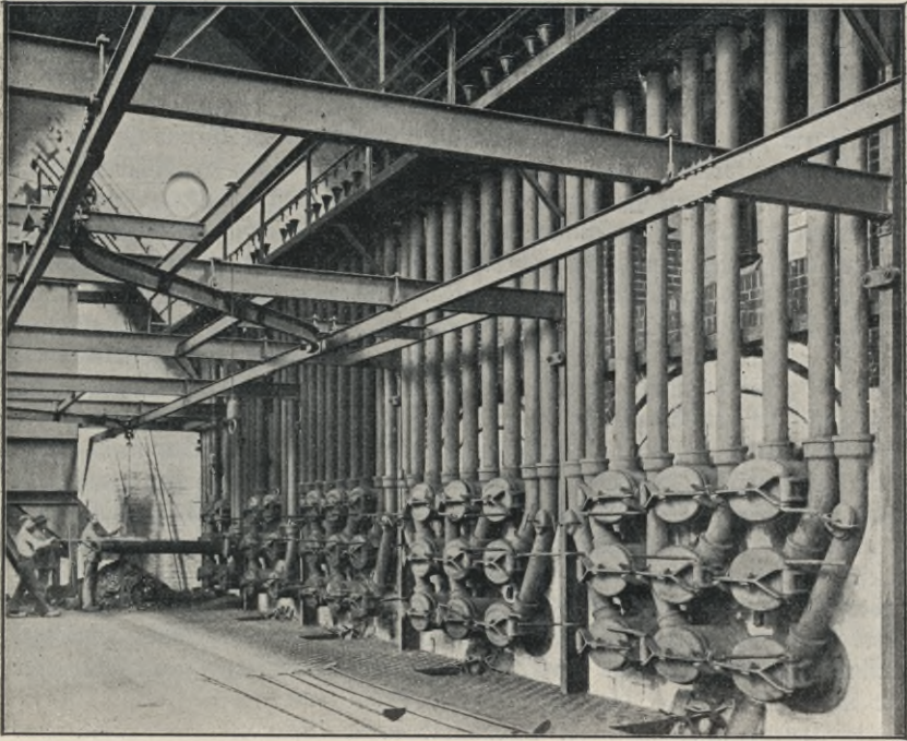
Abb. 112. Ofen-Anlage der städtischen Gasanstalt.
