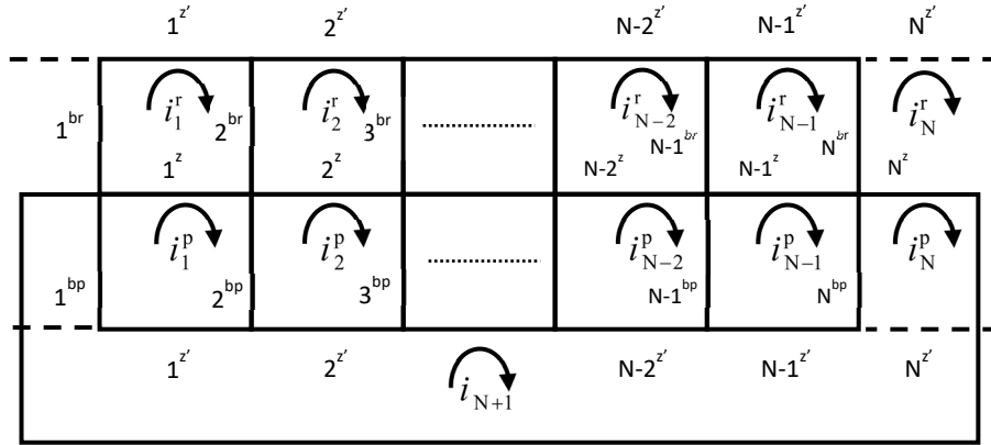
Rys. 2.2 Rozwinięty schemat obwodów wirnika zwartego wspólnym pierścieniem.
