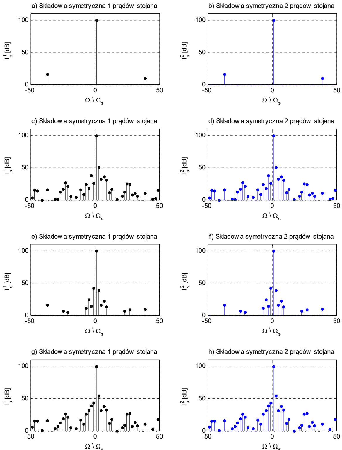
Rys. 2.16 Względne widmo amplitudowe składowych symetrycznych prądów stojana w funkcji pulsacji – silnik zwarty osobnymi pierścieniami, przerwa w fazie obwodu stojana, a-b) symetryczny wirnik, c-d) przerwa w pręcie klatki rozruchowej, e-f) przerwa w pręcie klatki pracy, g-h) przerwa w pręcie klatki rozruchowej i pręcie klatki pracy.
