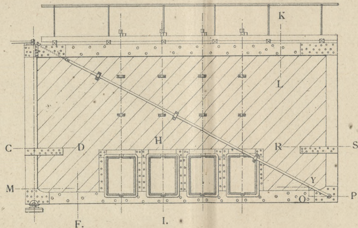
Разрѣзъ по HI.
