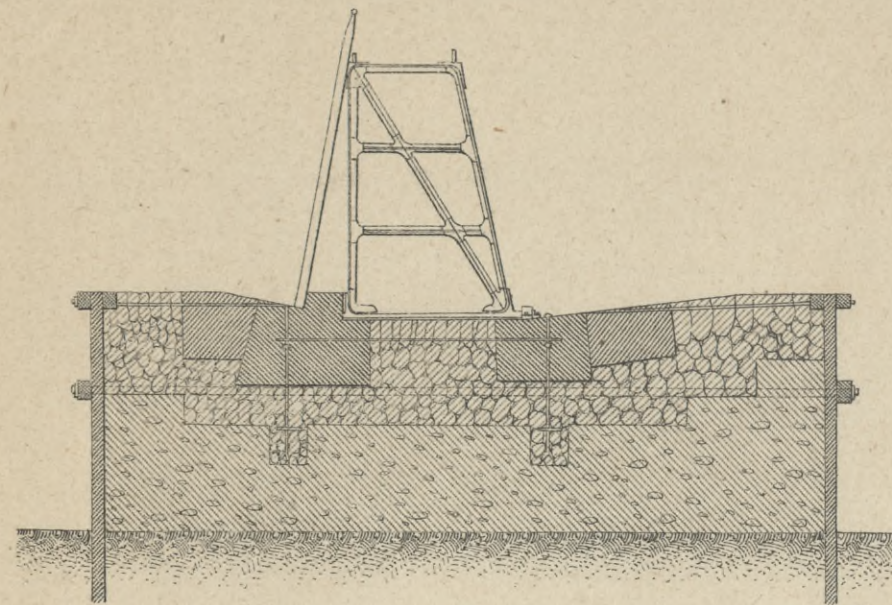
Разрѣзъ по АВ.
