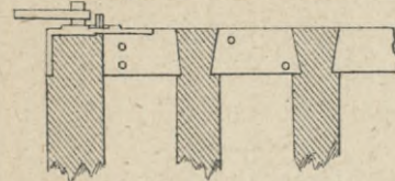
Разрѣзъ по АВ.
