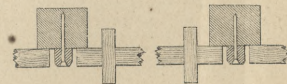
Разрѣзъ щитовъ и стоскъ.
