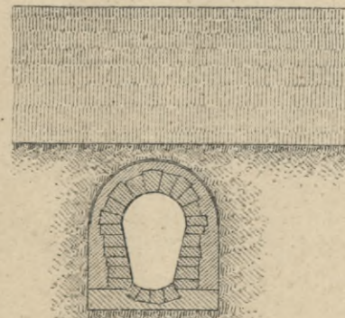
Поперечный разръзъ по оси канала.
