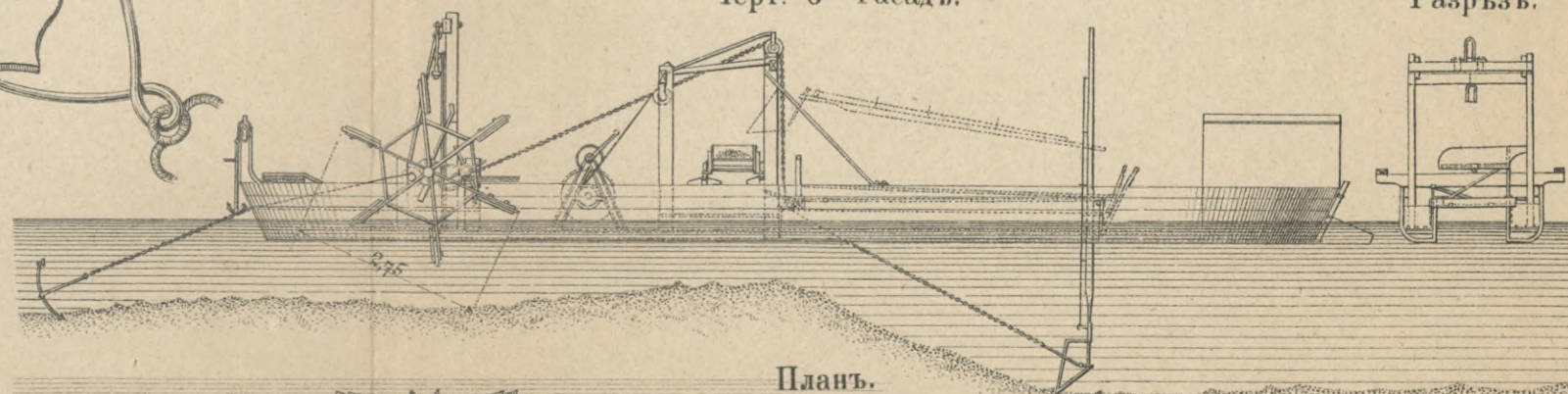
Черт. 6 Фасадъ.
