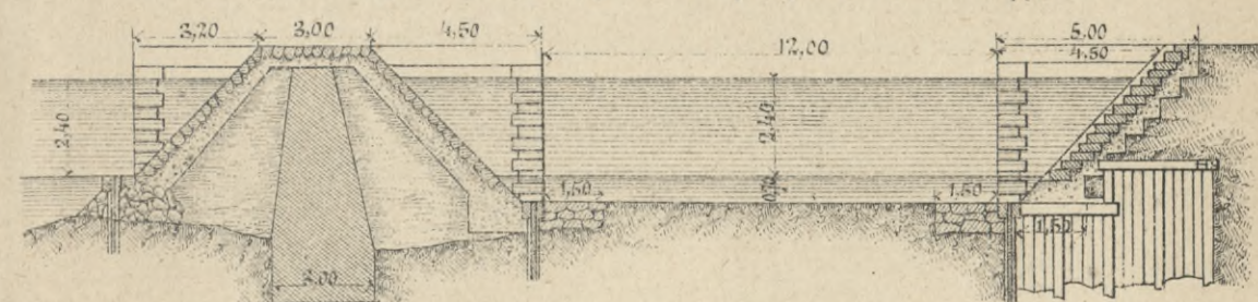
Черт. 6в. Прод. разръзъ верхней шлюзн. части
