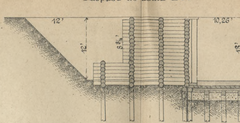
Разрѣзъ по линіи EF.
