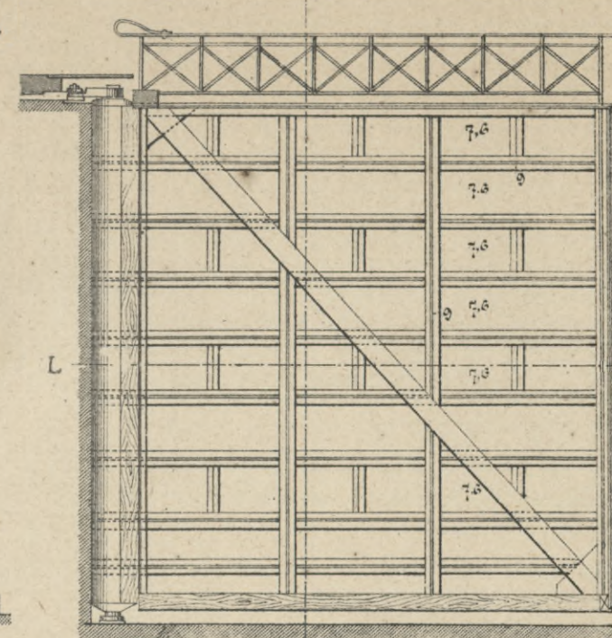
Черт. 3 б. Разрѣзъ по LM.
