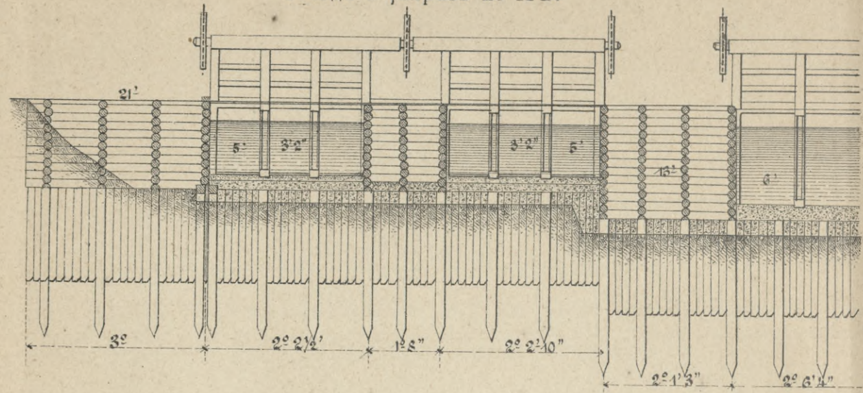
Фасадъ и разръзъ по А В.
