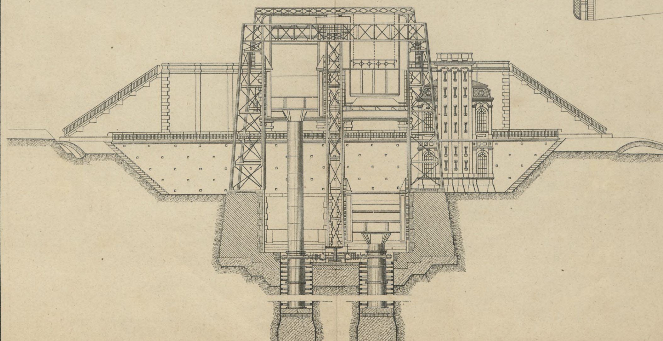
Поперечный разръзъ.
