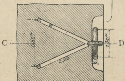
Планъ по шву.
