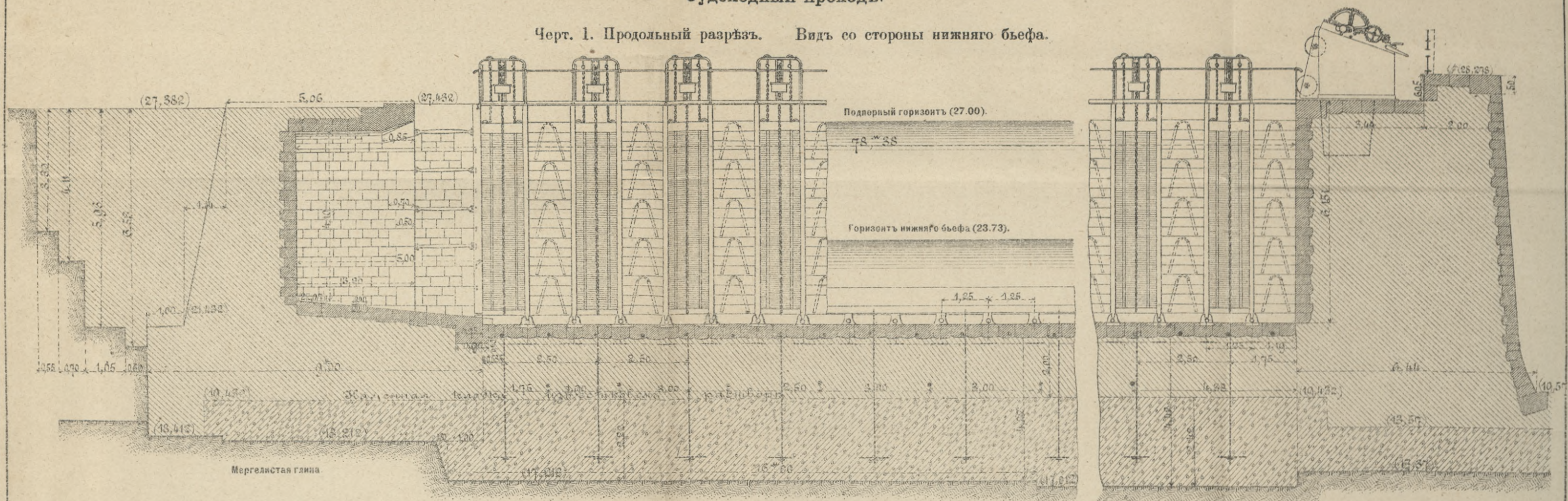
Черт. 2. Планъ.
