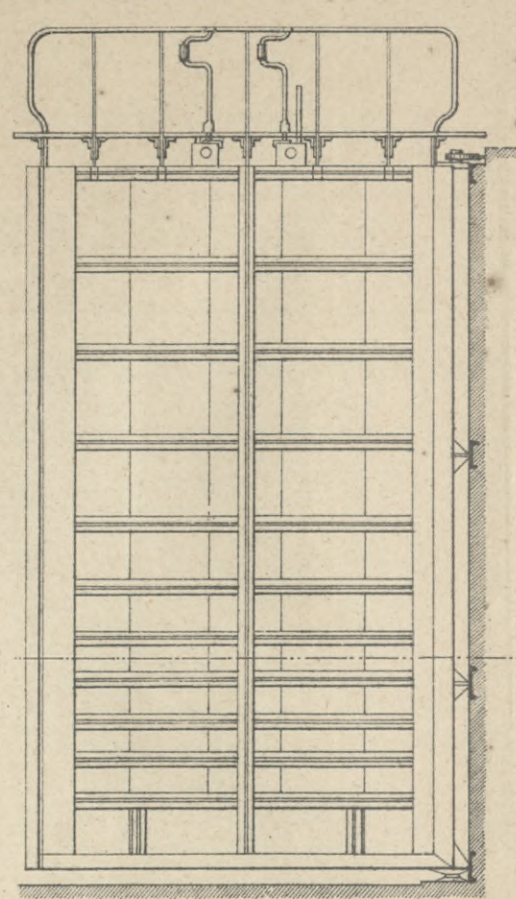
Черт. 2 д. Разрѣзъ по FF.
