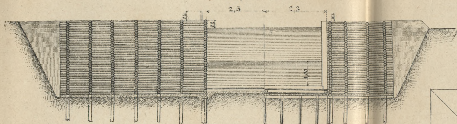
Разрѣзъ по С D.
