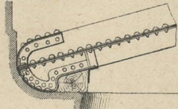
Черт. 3 з. Створный столбъ.
