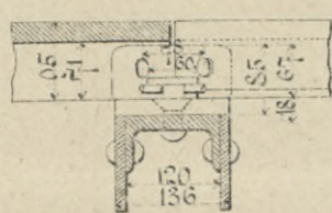
Черт. 7. Разръзъ ВВ.
