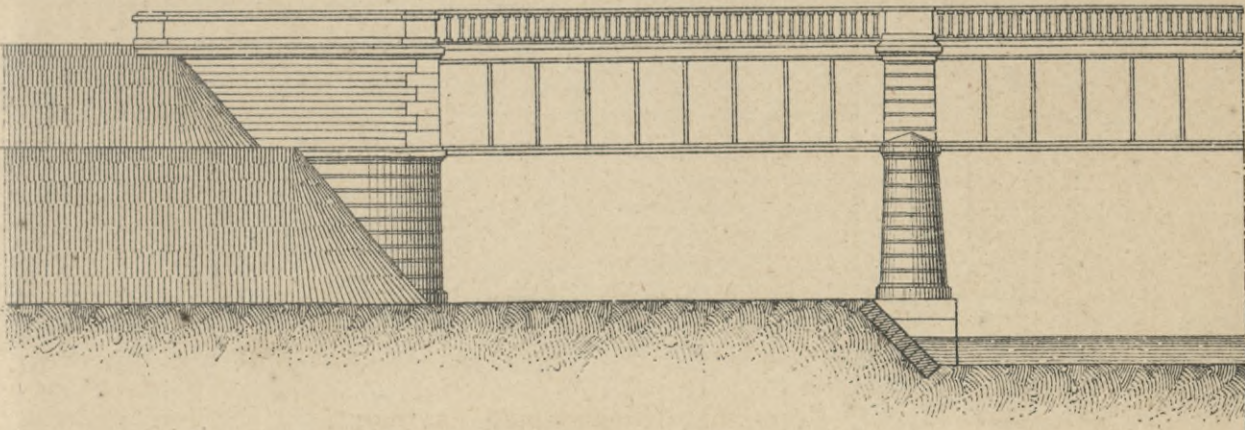
Черт. 3а. Фасадъ.
