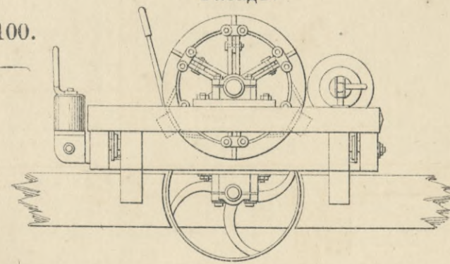
Черт. 103. Фасадъ.
