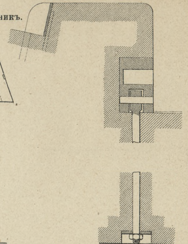
Разрѣзъ подферменнаго камня по оси верхняго подшипника АВ.
