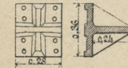
Черт. 2 з. Упорный уголокъ.
