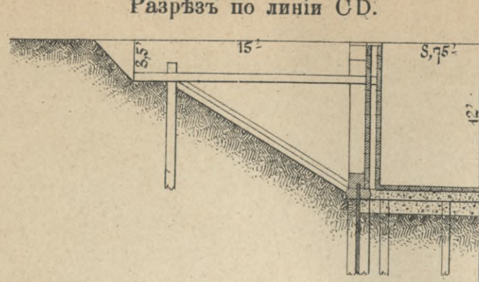
Разрѣзъ по линіи CD.
