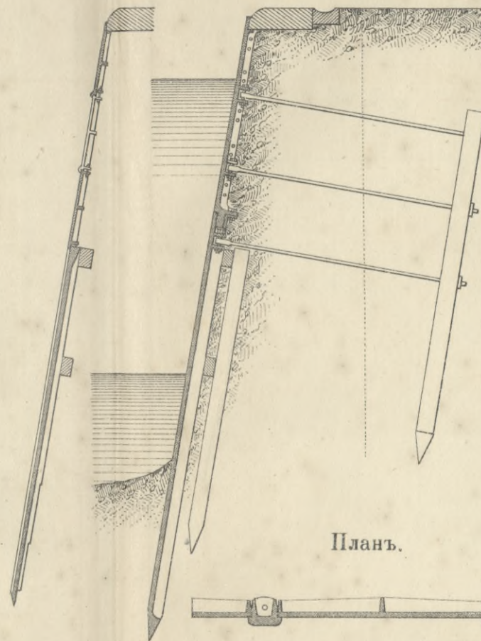
Разрѣзъ по С D.
