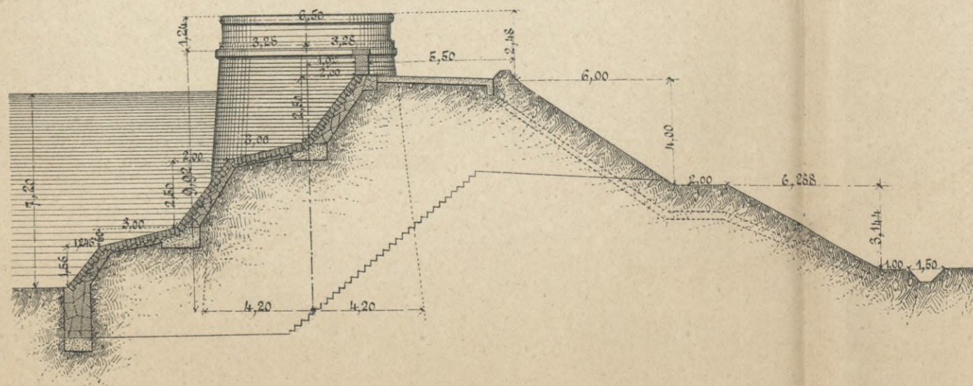
Черт. 2. Попер. разр. Плотины.
