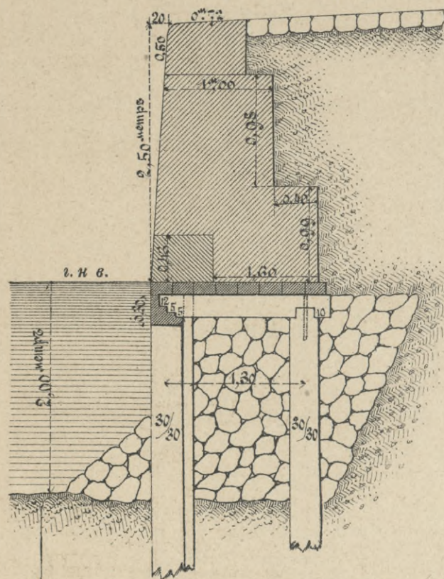
Черт. 8. Разрѣзъ по СД.
