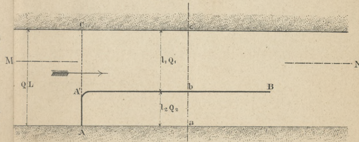
Черт. 8а. Планъ.
