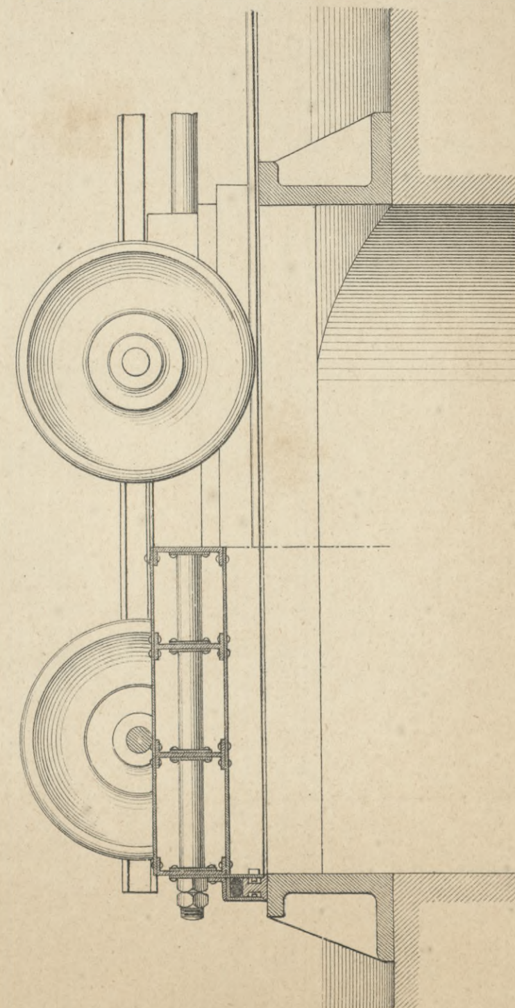
Черт. 3. Разрѣзъ и боковой видъ по абсд. (черт. 2).
