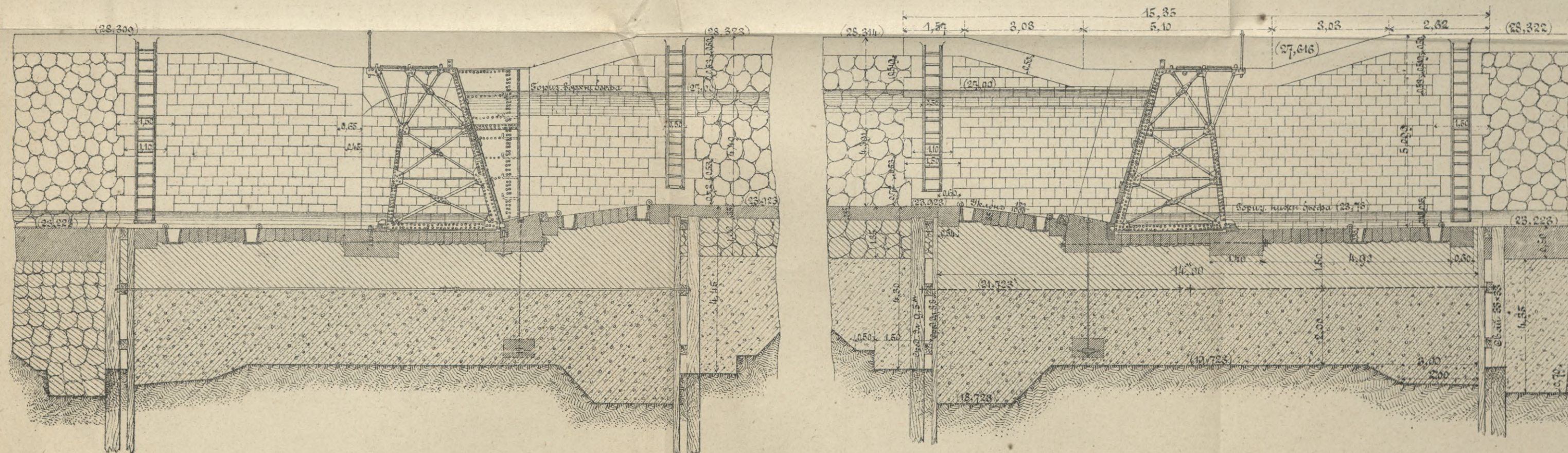
Черт. 4. Поперечный разръзъ по СД.
