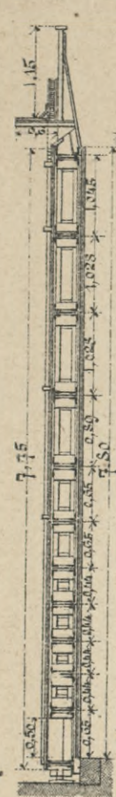
Черт. 2 в. Разрѣзъ по АВ.
