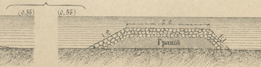
Разрѣзъ по м м.
