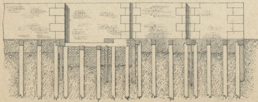
Черт. 1 б. Разрѣзъ по АВ.
