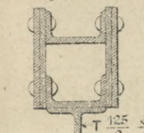
Черт. 6. Разръзъ AA.
