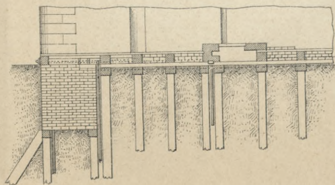
Черт. 1б. Разрѣзъ по АВ.
