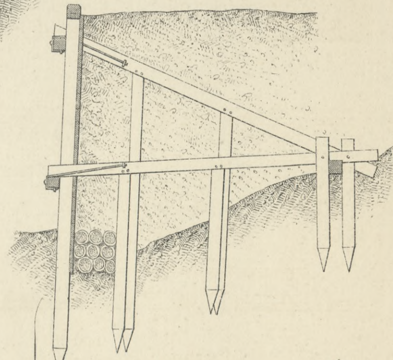
Черт. 5. Разрѣзъ.
