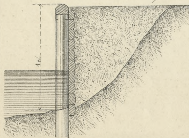
Черт. 3. Разрѣзъ.
