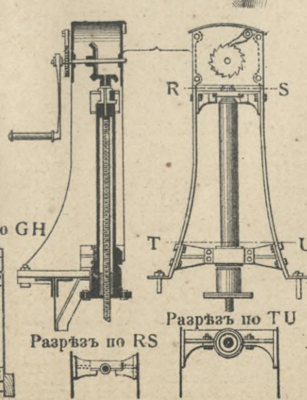
Черт. 4. Домкратъ для подъема щита.
