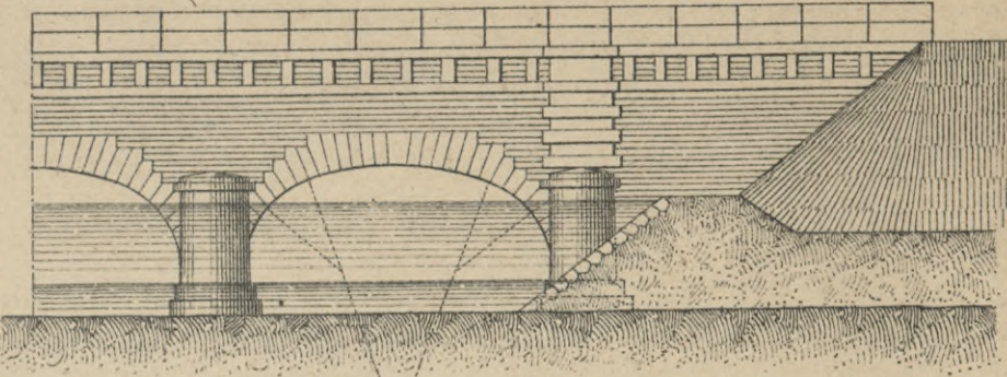
Черт. 4б. Фасадъ.
