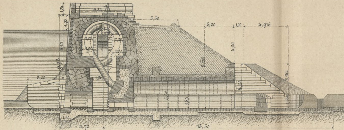
Черт. 1. Разрѣзь по оси
