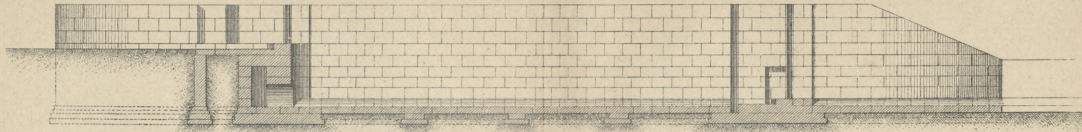
Черт. 1 а. Продольный разръзъ
