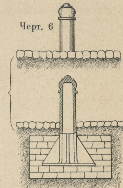
Разрѣзъ.
