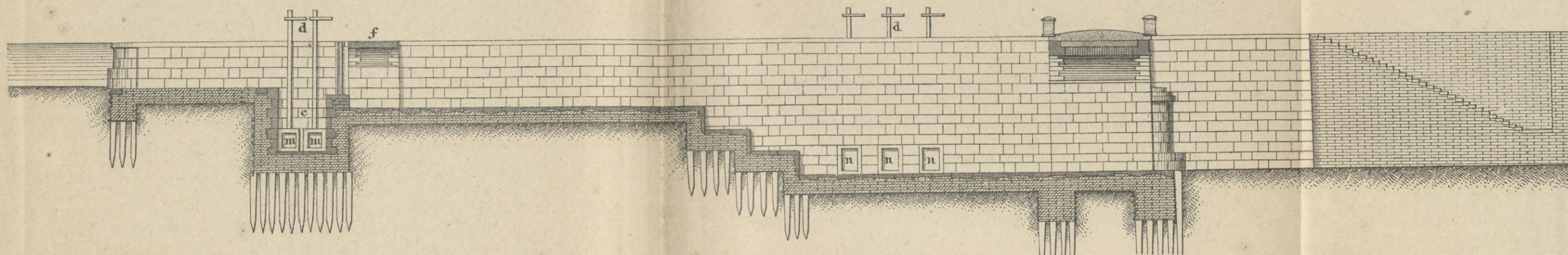
Продольный разрѣзъ по линіи СD.
