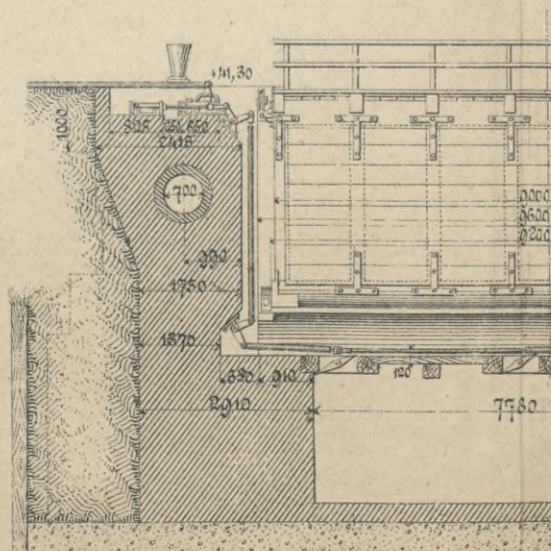
Черт. 2 в. Разрѣзъ по с д.
