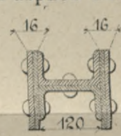
Черт. 11. Нижнее ребро
