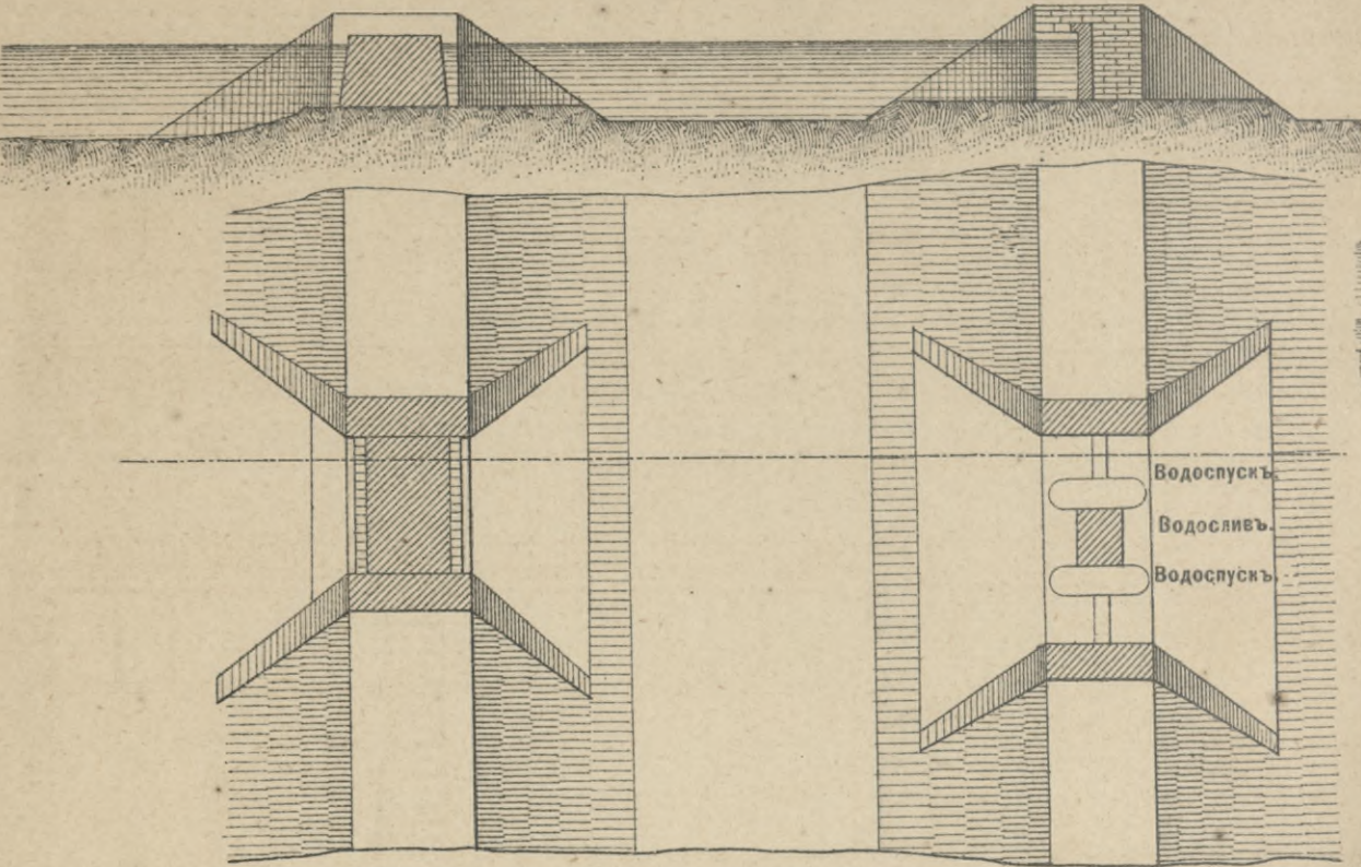
Черт. 1. Разрѣзь по АВ.
