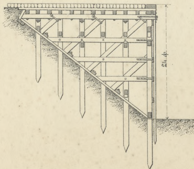
Разрѣзъ.
