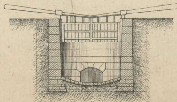
Черт. 1 в. Разръзъ по С D.
