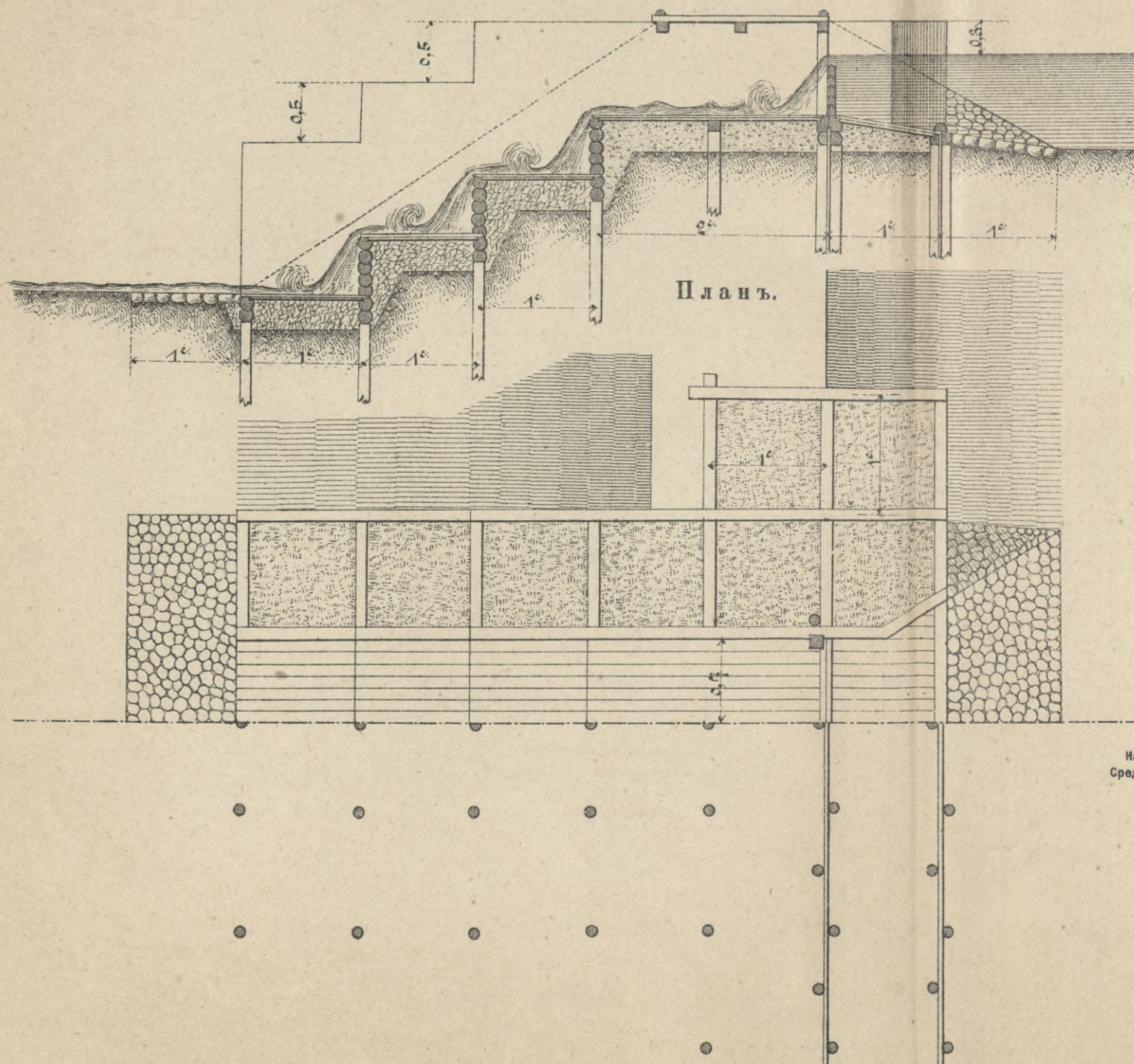
Черт. 1. Разрѣзъ по АВ.
