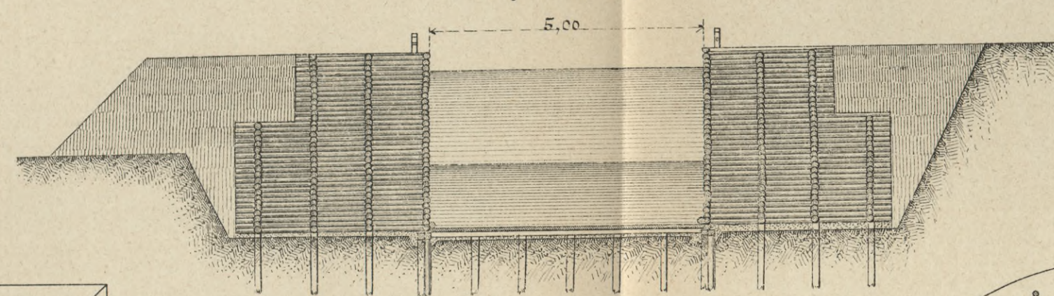
Разрѣзъ по Е F.
