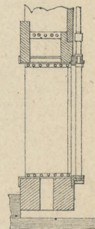
Горизонтальный разрѣзъ.
