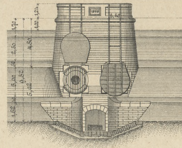
Черт. 3. Фасадъ башни.
