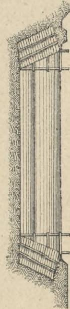
Поперечный разрѣзъ верхней головы шлюза выше лѣваго устоя и по правому.
