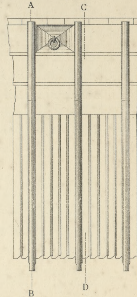
Фасадъ.
