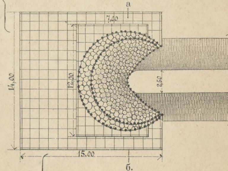
Планъ
