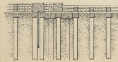
Черт. 2д. Разрѣзъ по EF.
