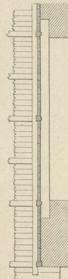
Черт. 2д. Разрѣзъ по EF.
