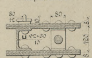
Черт. 10. Разръзъ EE.
