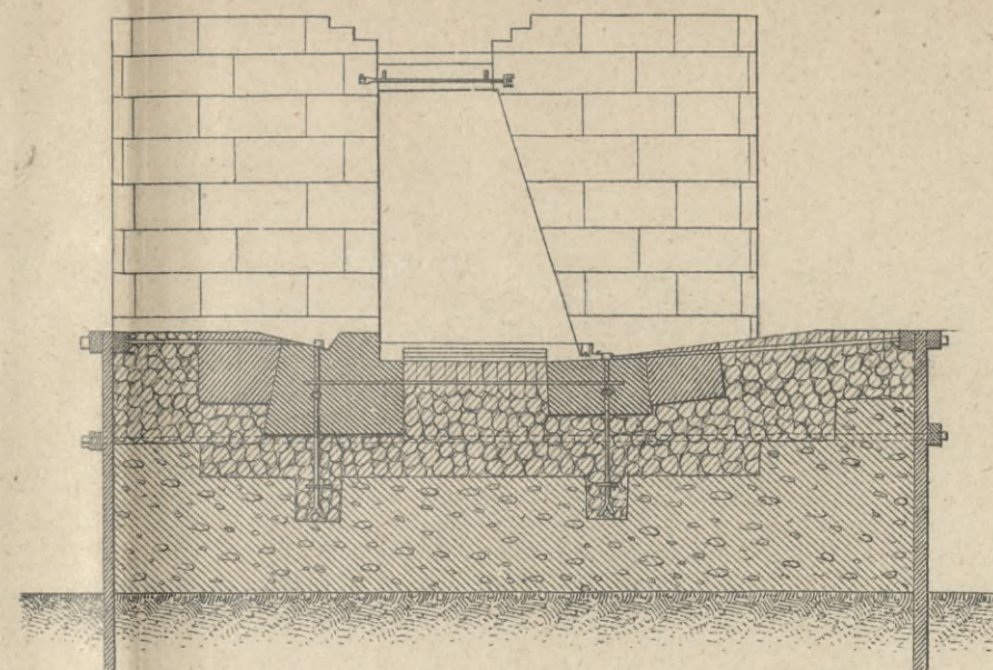
Разрѣзъ по CD.
