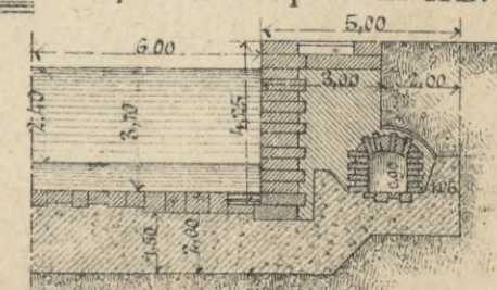
Черт. 6д. Разръзъ по АВ.
