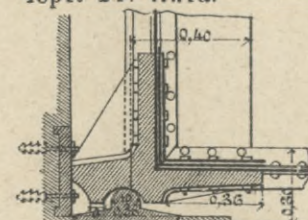
Черт. 2 г. Пята.
