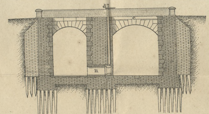
Поперечный разрѣзъ по линіи LM.
