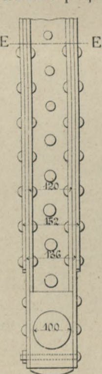
Черт. 11. Нижнее ребро
