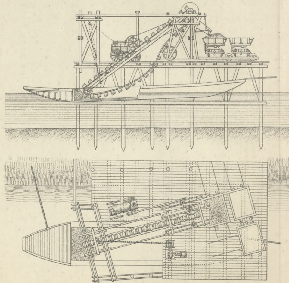
Черт. 2. Фасадъ.
