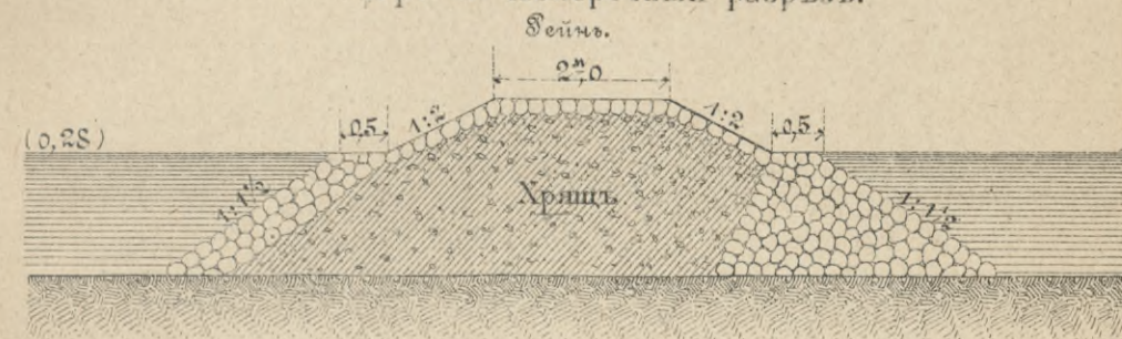
Черт. 5. Поперечный разръзъ.
