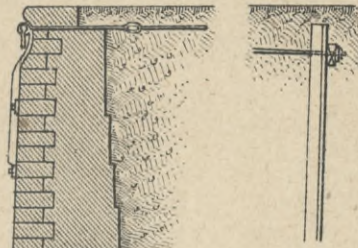
Разрѣзъ.
