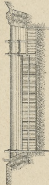
Поперечный разрѣзъ верхней головы шлюза по стѣнкѣ паденія и ниже ея.
