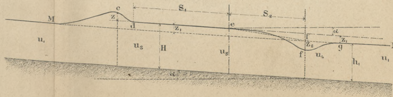
Черт. 8б. Продольная профиль по MN
