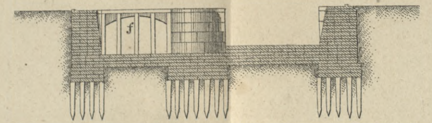
Поперечный разрѣзъ по линіи EF.
