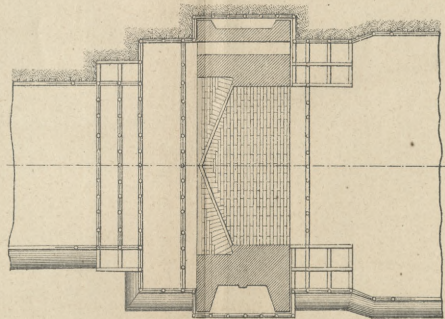
Планъ шлюзной камеры.
