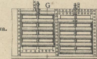
Фасадъ щитовъ.
