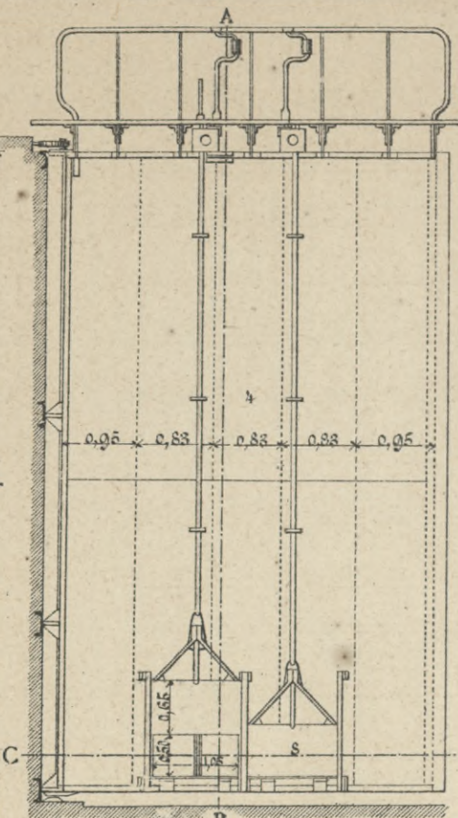
Черт. 2 е. Разрѣзъ по СД.
