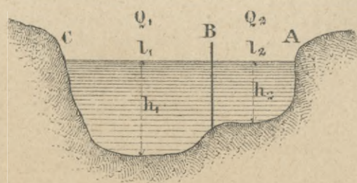
Черт. 8в. Поперечная профиль. по сба.
