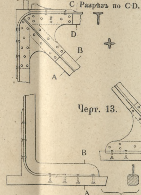
Детали фермы.
