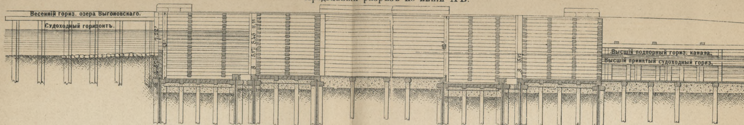
Черт. 1. Продольный разръзъ по линіи АВ.
