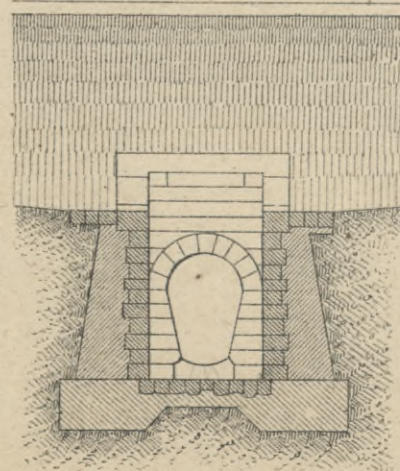
Поперечный разръзъ по колодцу.
