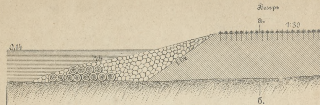
Черт. 1. Продольный разръзъ.
