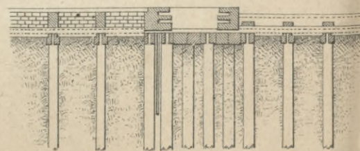
Черт. 2г. Разрѣзъ по CD.
