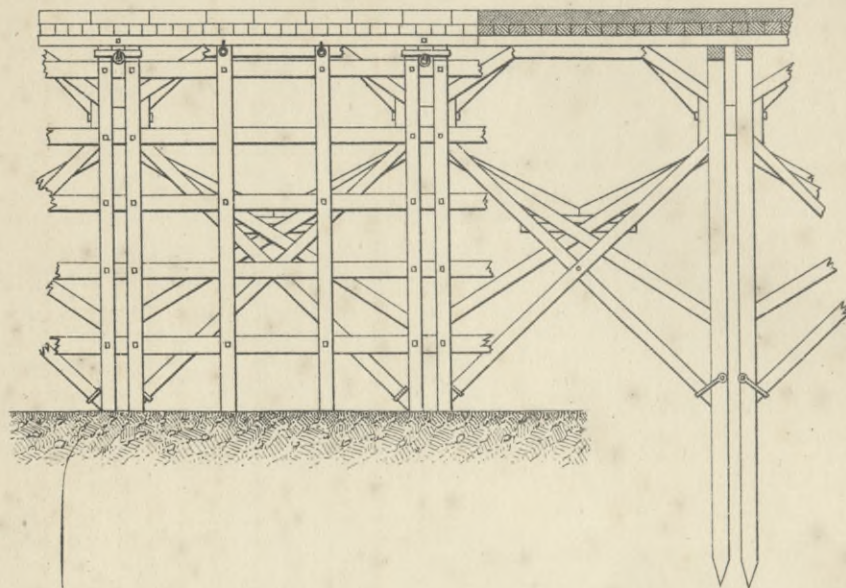
Фасадъ.
