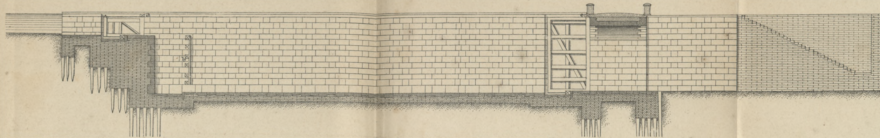
Продольный разрѣзъ по линіи АВ.
