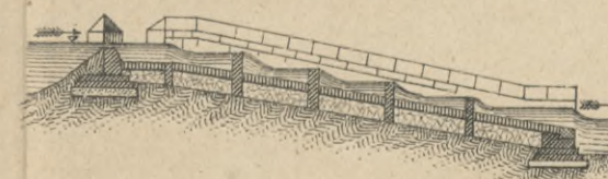
Черт. 3 б. Разрѣзъ по а b c d.
