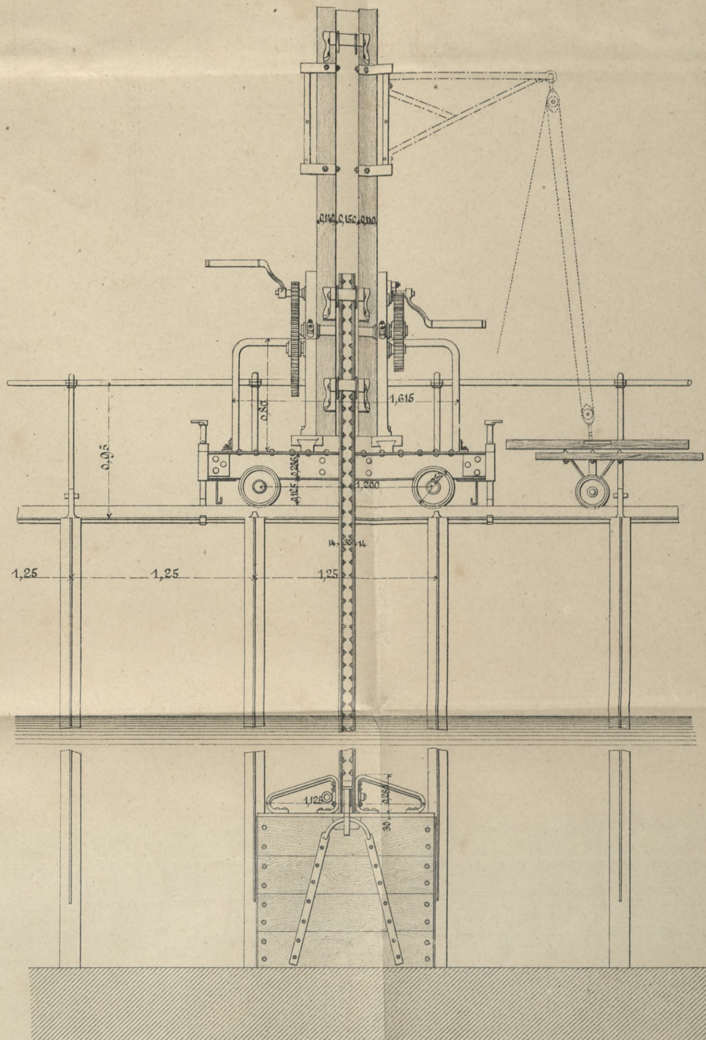
Поворотный кранъ 300 кил.
