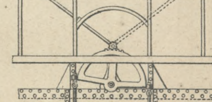
Черт. 5. Балансирный механизмъ для подъема щитовъ.
