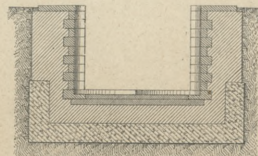
Черт. 3. Разръзъ по А В.
