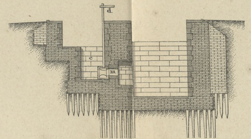
Поперечный разрѣзъ по линіи СН.
