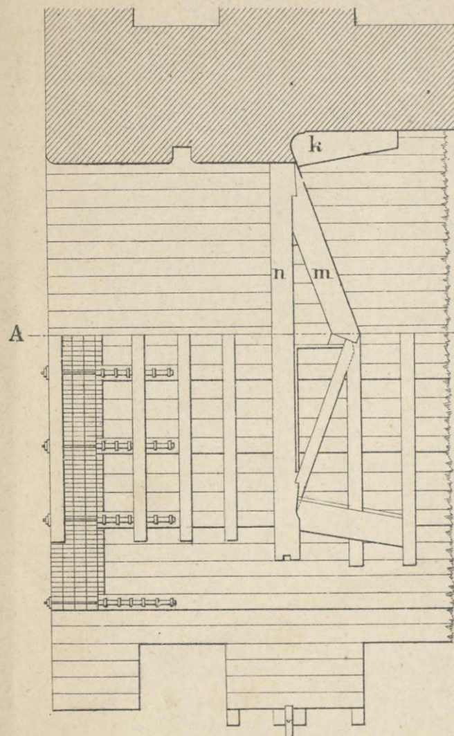
Черт. 1б. Разрѣзъ по АВ.
