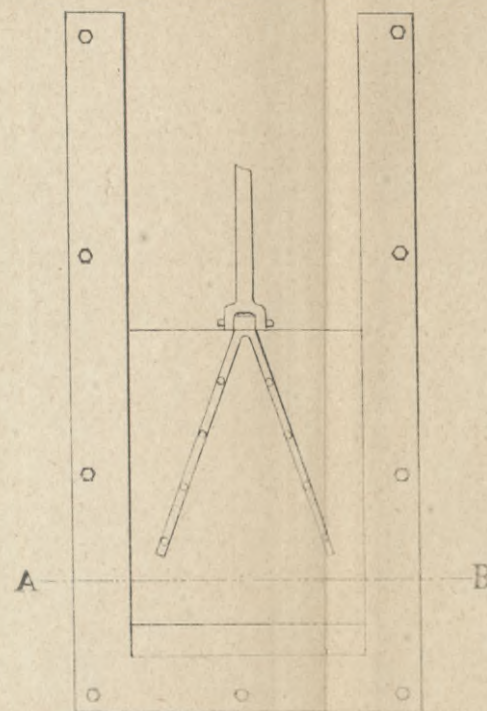
Черт. 2 в. Разрѣзъ по А В.
