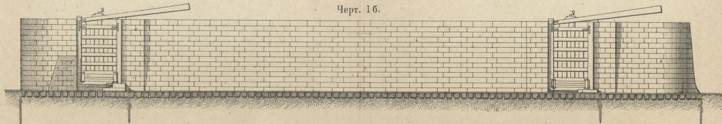
Продольный разръзъ.
