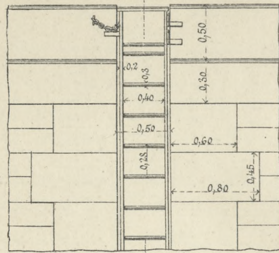
Черт. 2. Фасадъ.
