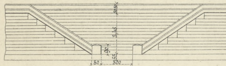
Черт. 2. Фасадъ.
