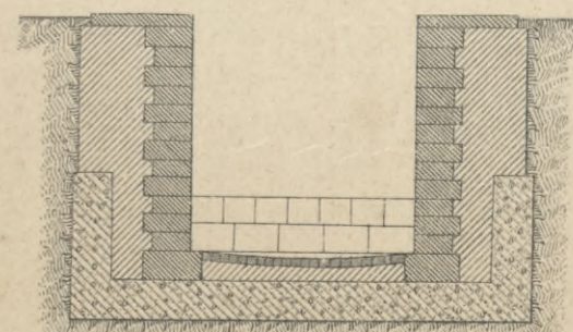
Черт. 4. Разръзъ по С D.
