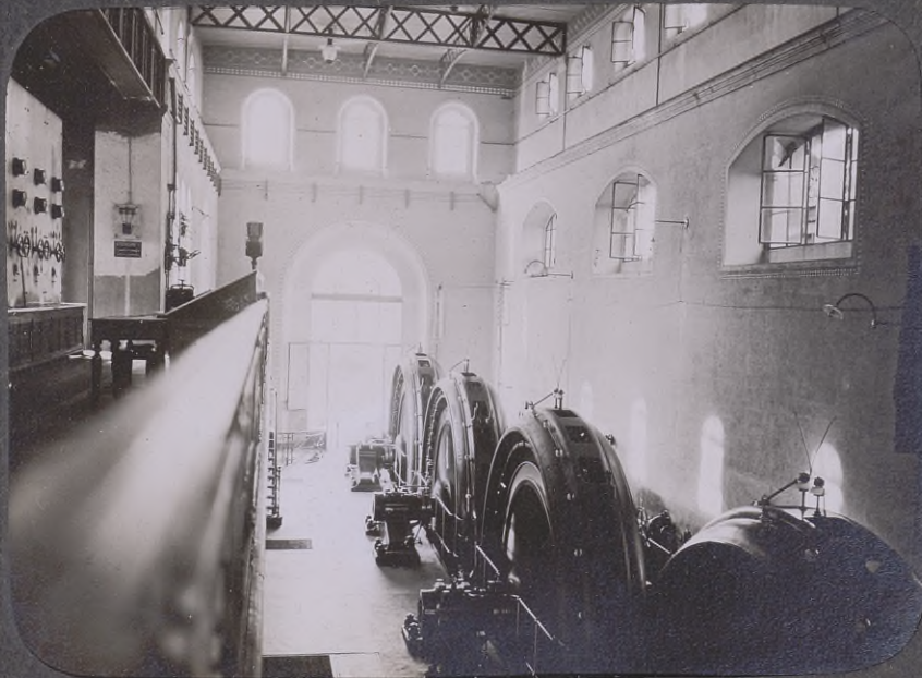
35. Turbigo, Maschinenraum.
