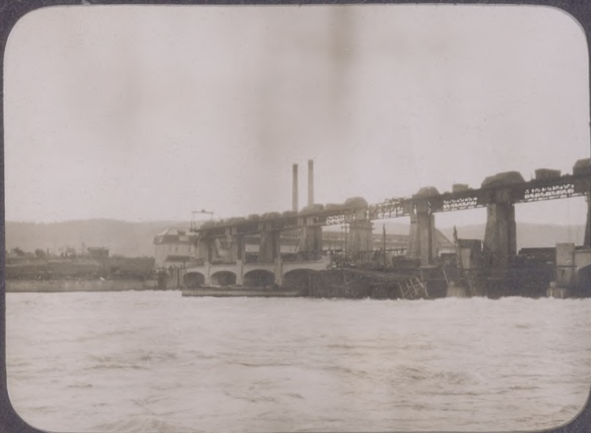
3. Wehr Augst-Wyhlen im Bau.
