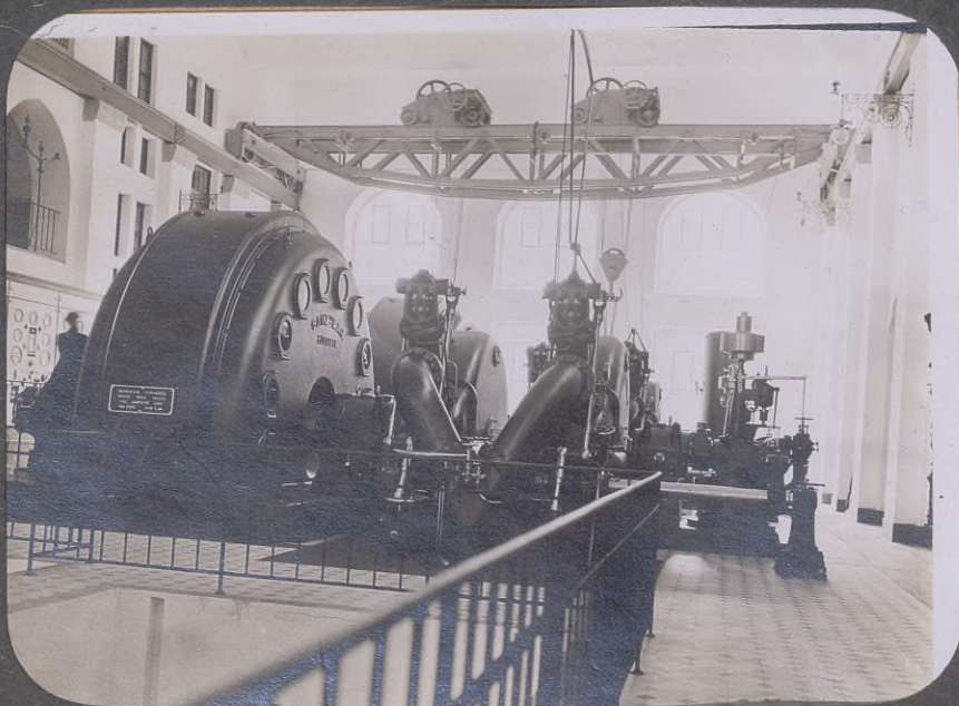
47. Schnalstalwerk, Maschinenraum.
