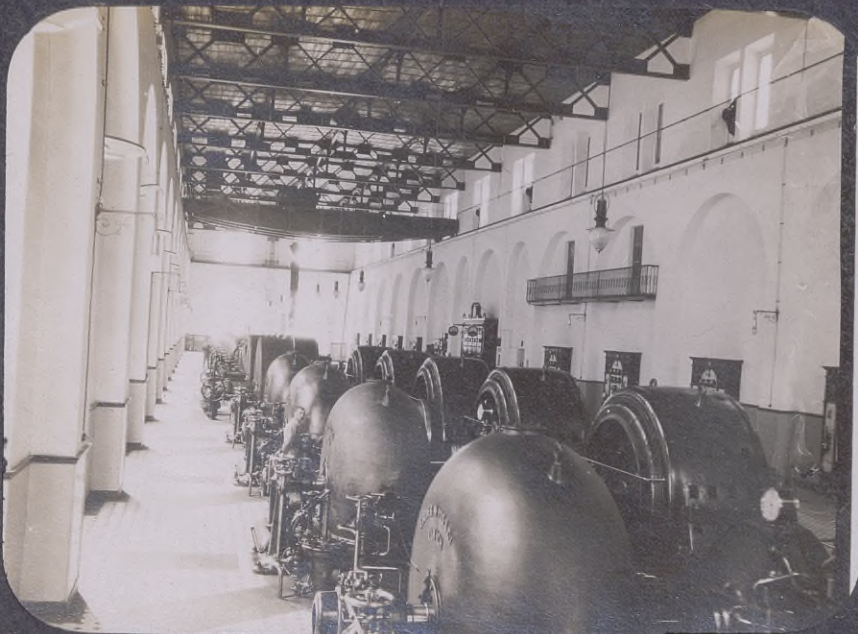
23. Campocologno, Maschinenraum.
