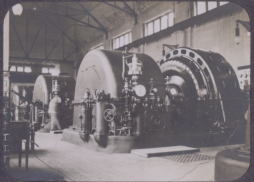
18. Löntschwerk, 6000 P. Turbodynamo.
