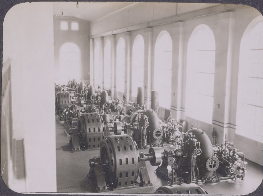
21. Albulawerk, Maschinenraum.
