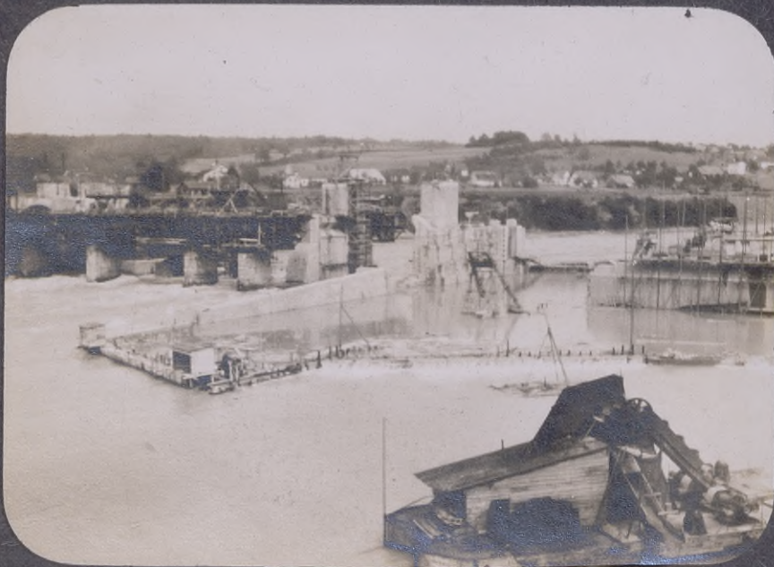
7. Laufenburg, Wehr im Bau.
