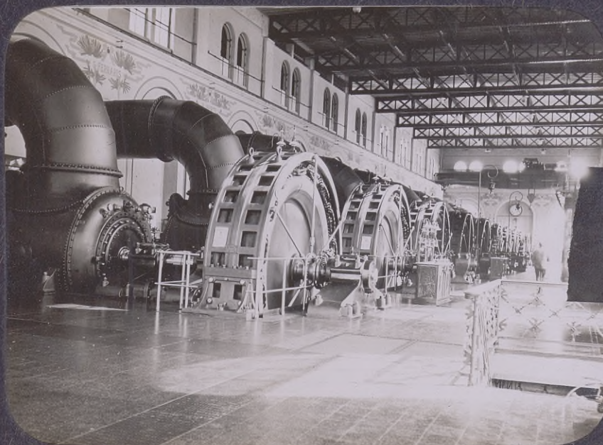
27. Vizzola, Maschinenraum.
