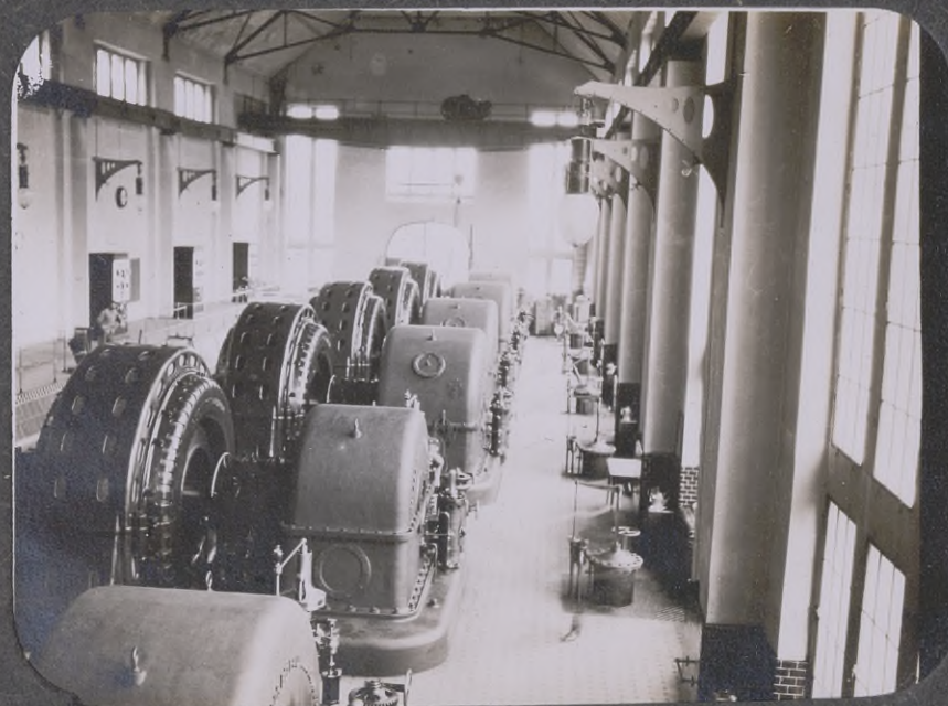
16. Löntschwerk, Maschinenraum.
