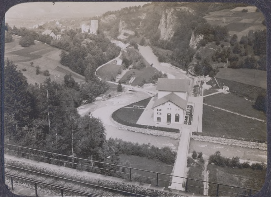
22. Albulawerk, Rohrleitung u. Krafthaus.
