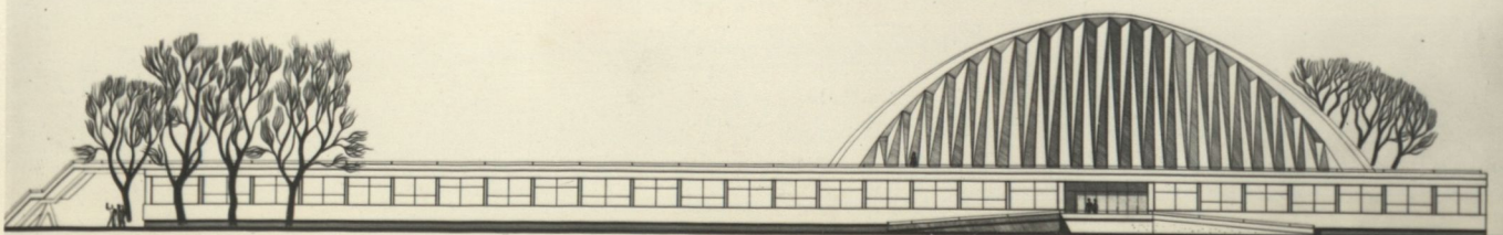
ELEVACJA POŁNOČNA - 1:100
