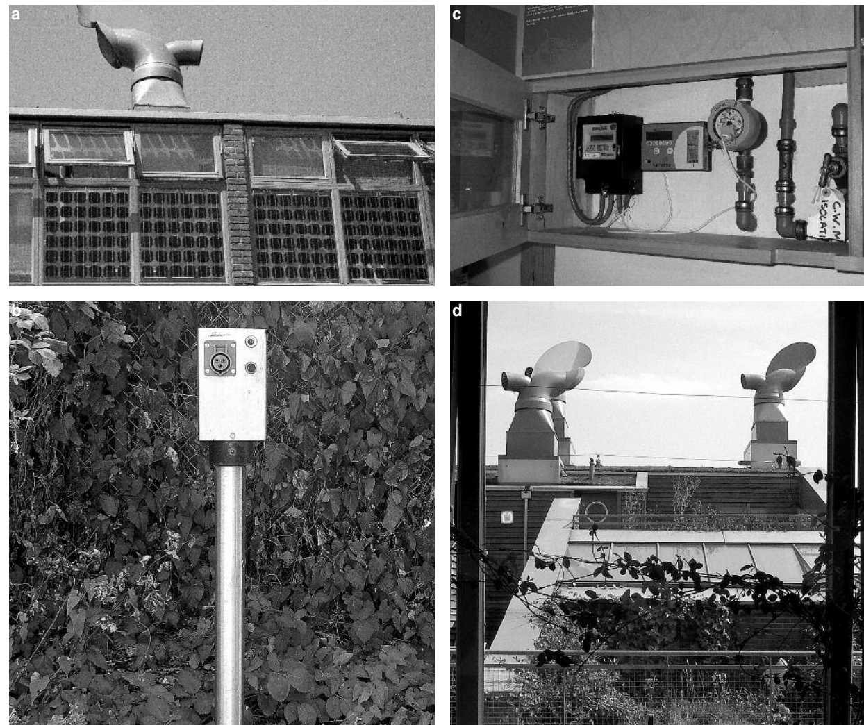
Zespół mieszkaniowy BedZED, Londyn, a – ogniwa fotowoltaiczne, b – miejsce parkingowe z ładowaniem dla samochodu z napędem elektrycznym, c – widoczne dla mieszkańcy wskaźniki zużycia energii i wody, d – zieleń w ogrodzie, na tarasie i na dachu (zdjęcia wykonane przez autorkę w ramach projektu SusPurPol, w czasie wizyty studialnej w Wielkiej Brytanii) Residential complex BedZED, London, a – photovoltaic cells, b – parking place with a charger for a car with electric drive, c – visible indicators of energy and water usage, d – greenery in the garden, on the terrace and on the roof (photos taken by the author within the SusPurPol project, during a study visit to Great Britain)
