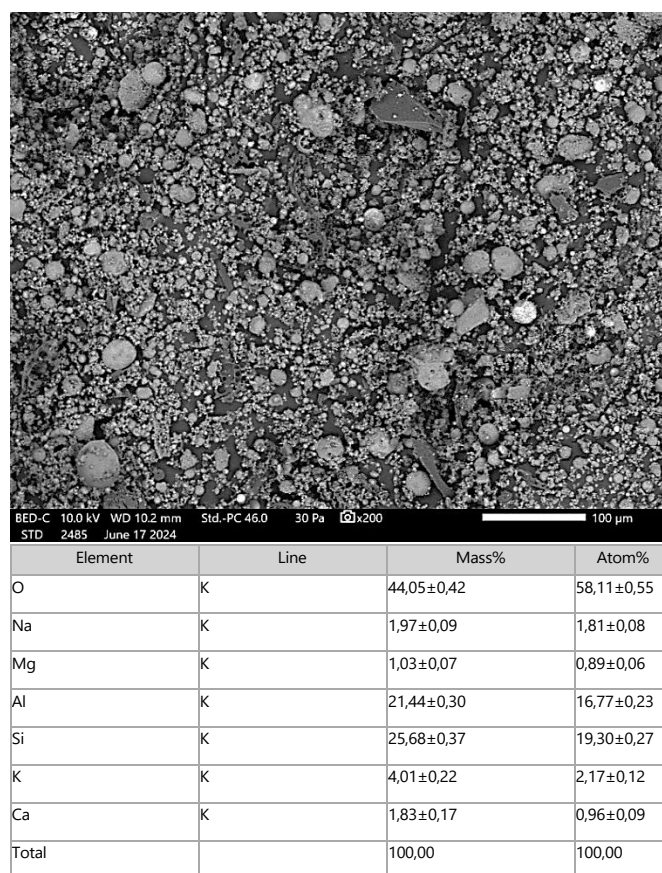
Rysunek 8. Morfologia popiołu lotnego ze spalania węgla kamiennego wraz z analizą składu pierwiastkowego metodą EDS.
