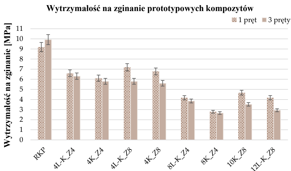
Rysunek 25. Porównanie wytrzymałości na zginanie prototypowych kompozytów z różnym układem zbrojenia.
