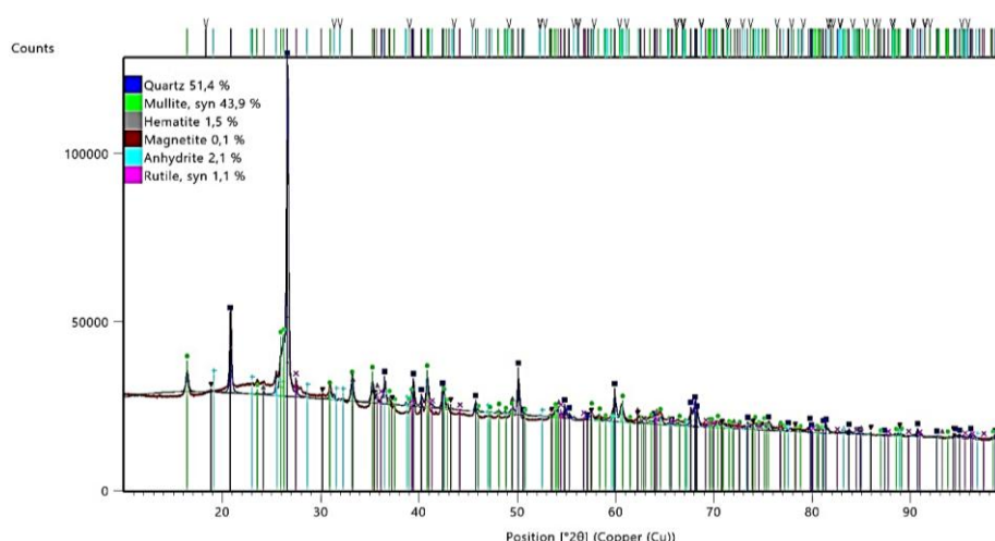
Rysunek 9. Dyfraktogram ilustrujący skład fazowy popiołu lotnego ze spalania węgla kamiennego.
