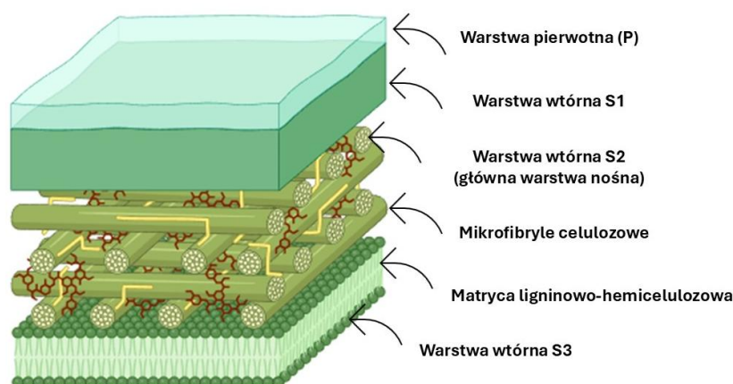
Rysunek 3. Schemat budowy morfologicznej ściany komórkowej włókna roślinnego z zaznaczeniem warstwy pierwotnej (P), warstw wtórnych (S1, S2, S3), mikrofibryli celulozowych oraz matrycy ligninowo-hemicelulozowej (na podstawie [49]).
