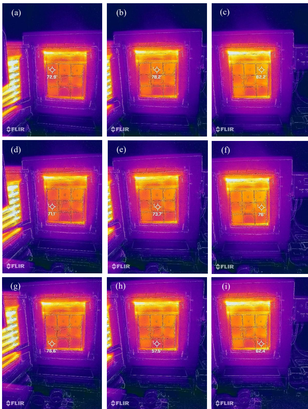
Rysunek 35. Analiza zachowania materiałów w warunkach oddziaływania temperatury 600°C: a) K2MP-4P-R, b) K1M-2P-R, c) K1MP-2P-R, d) K3M-6P-R, e) K3MP-6P-R, f) K2M-4P-R, g) RKG, h) K4M-8P-R, i) K4MP-8P-R.
