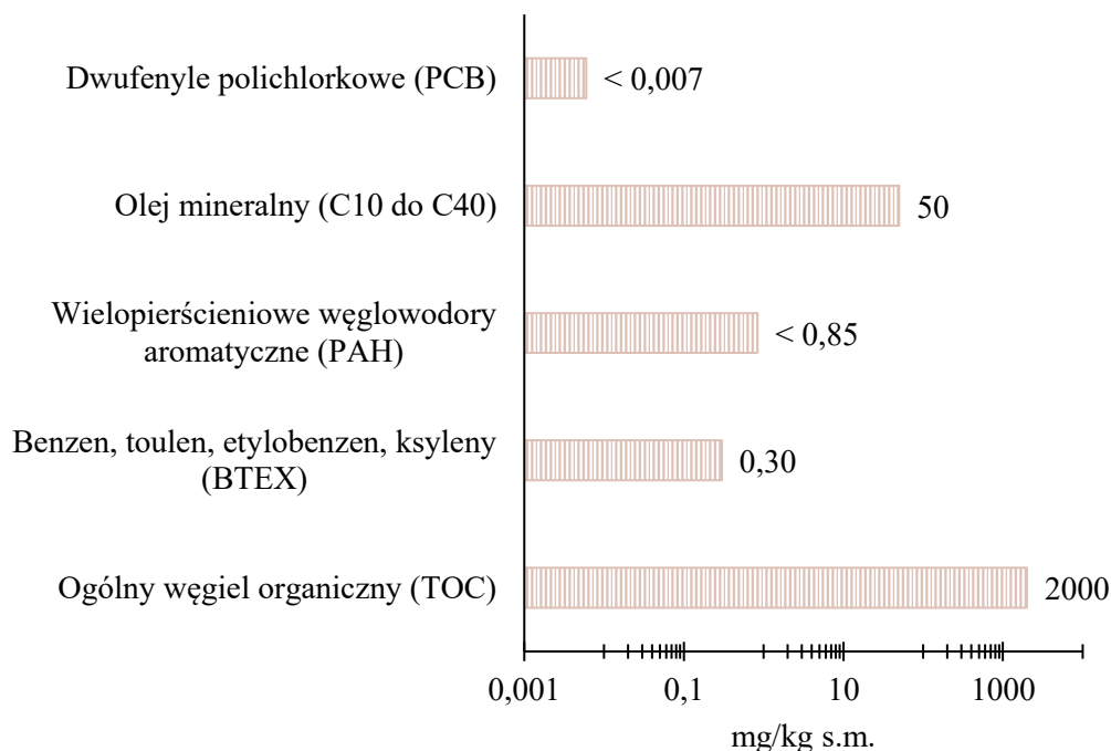
Rysunek 43. Wymywalność związków organicznych w materiale geopolimerowym.
