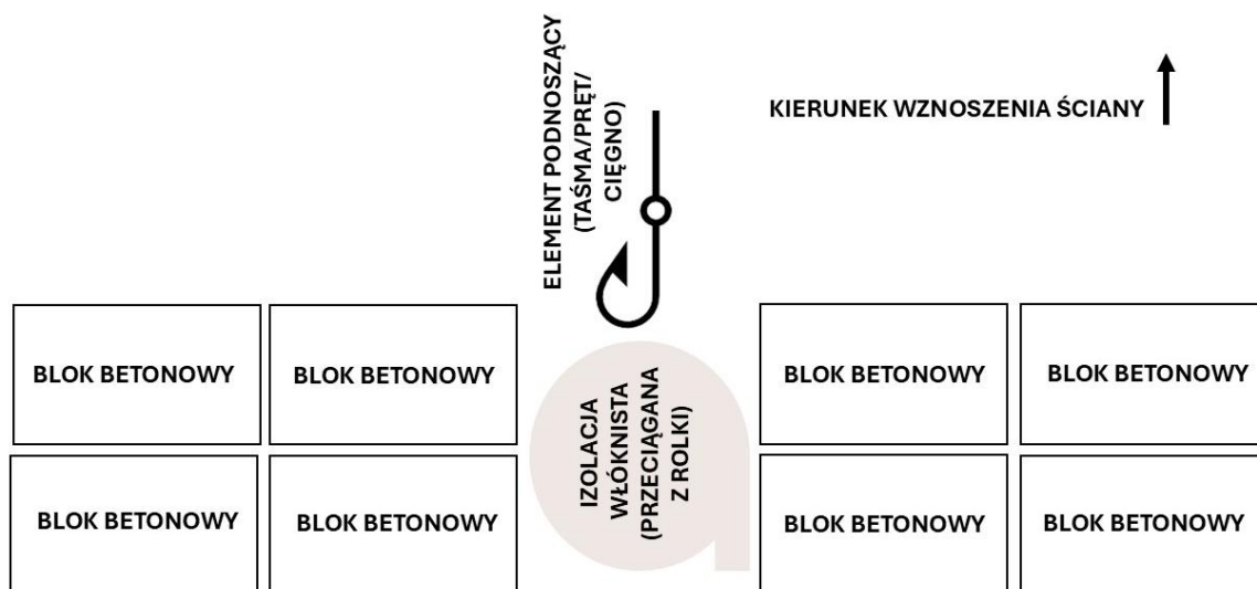
Rysunek 44. Schemat koncepcyjny rozwiązania do zgłoszenia patentowego (rysunek poglądowy).
