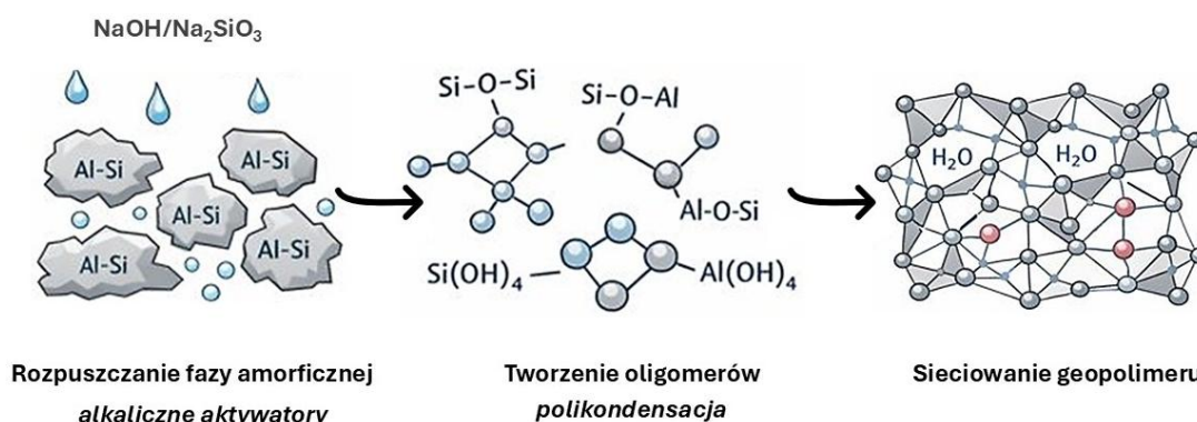
Rysunek 2. Schemat reakcji aktywacji alkalicznej glinokrzemianów - od rozpuszczania fazy amorficznej, przez tworzenie oligomerów, po sieciowanie struktury geopolimerowej (na podstawie [2]).
