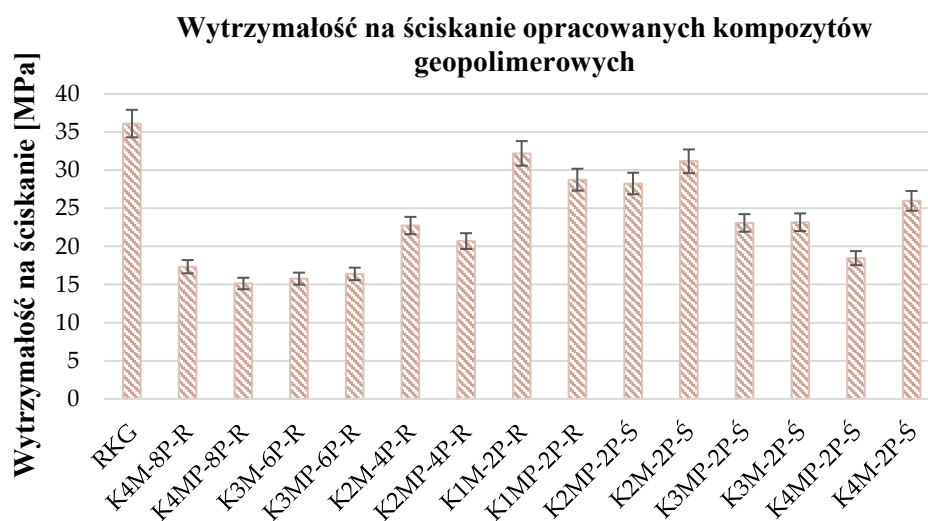
Rysunek 29. Wytrzymałość na ściskanie opracowanych kompozytów geopolimerowych.
