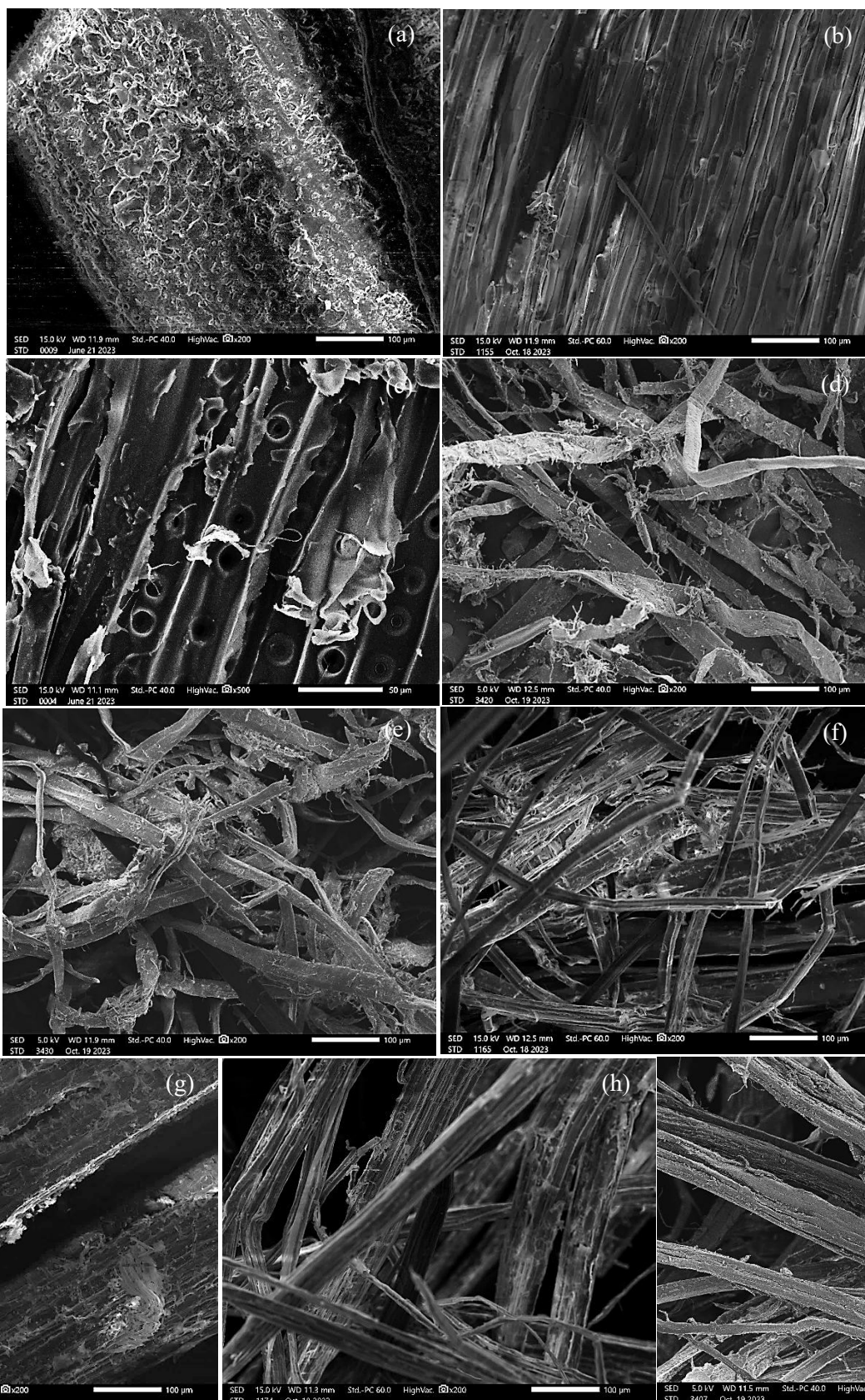
Rysunek 17. Obrazy mikroskopowe włókien ilustrujące różne typy materiałów: a) włókna kokosowe, b) siano, c) wióry drzewne, d) celuloza PRO AGRO, e) celuloza VestaEco CELL, f) włókna lniano-konopne, g) włókna konopne 1, h) włókna konopne 2, i) włókna konopne 3.
