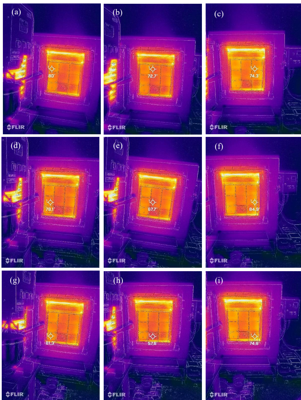
Rysunek 38. Analiza zachowania materiałów w warunkach oddziaływania temperatury 600°C: a) K3M-2P-Ś, b) K4MP-2P-Ś, c) K4M-2P-Ś, d) K2MP-2P-Ś, e) K2M-2P-Ś, f) K3MP-2P-Ś, g) K1MP- 2P-R, h) K4M-8P-R, i) K4MP-8P-R.
