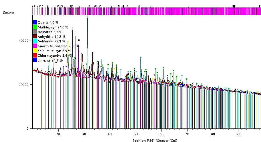
Rysunek 11. Dyfraktogram ilustrujący skład fazowy popiołu lotnego ze spalania węgla brunatnego.
