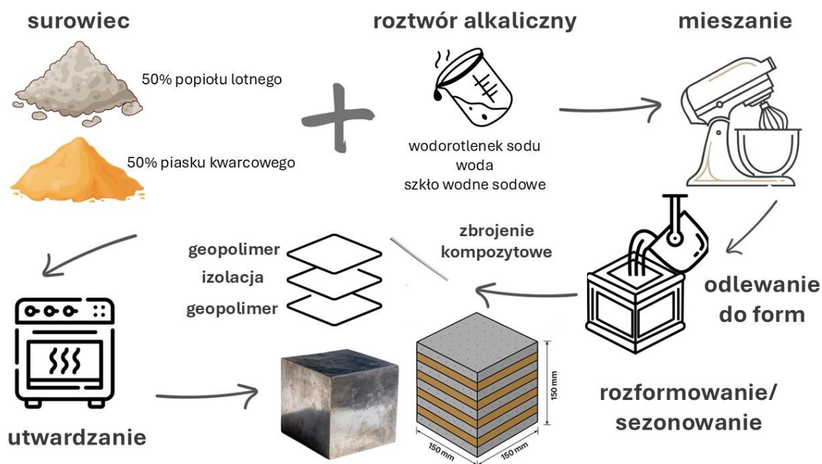
Rysunek 22. Graficzne ujęcie procedury przygotowania kompozytów w warunkach laboratoryjnych.
