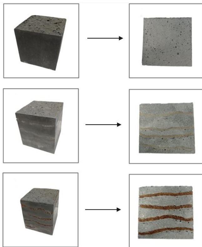
Rysunek 24. Prototypowe materiały kompozytowe - widok ogólny (po lewej) i przekrój poprzeczny (po prawej).
