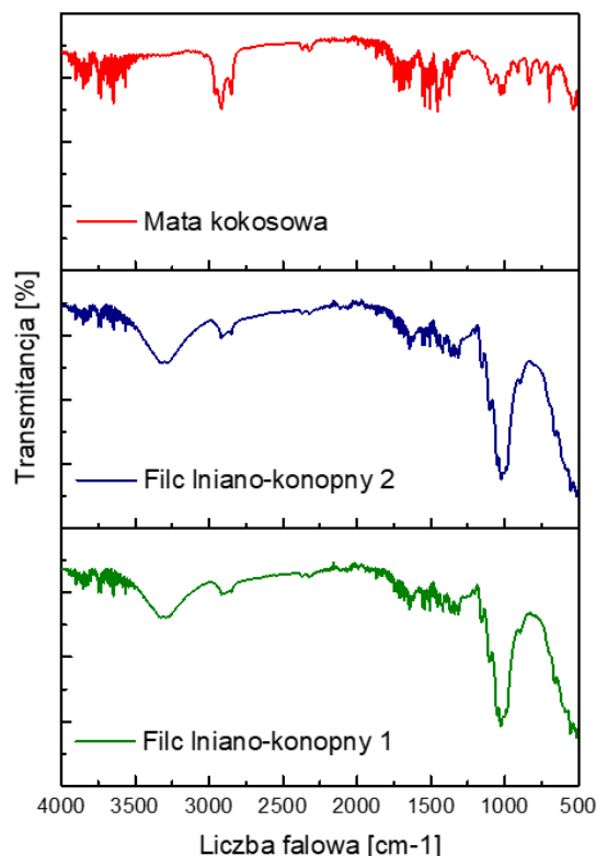
Rysunek 20. Widma FT-IR mat i filców.
