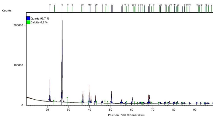
Rysunek 15. Dyfraktogram ilustrujący skład fazowy piasku kwarcowego.
