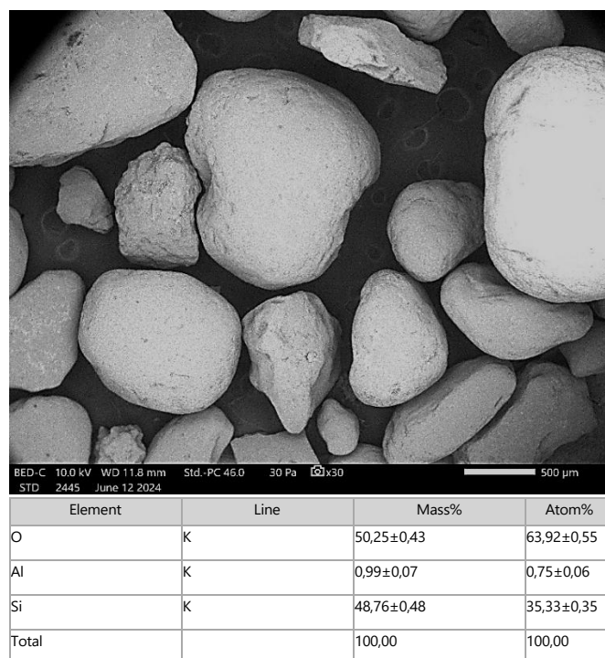
Rysunek 14. Morfologia piasku kwarcowego wraz z analizą składu pierwiastkowego metodą EDS.
