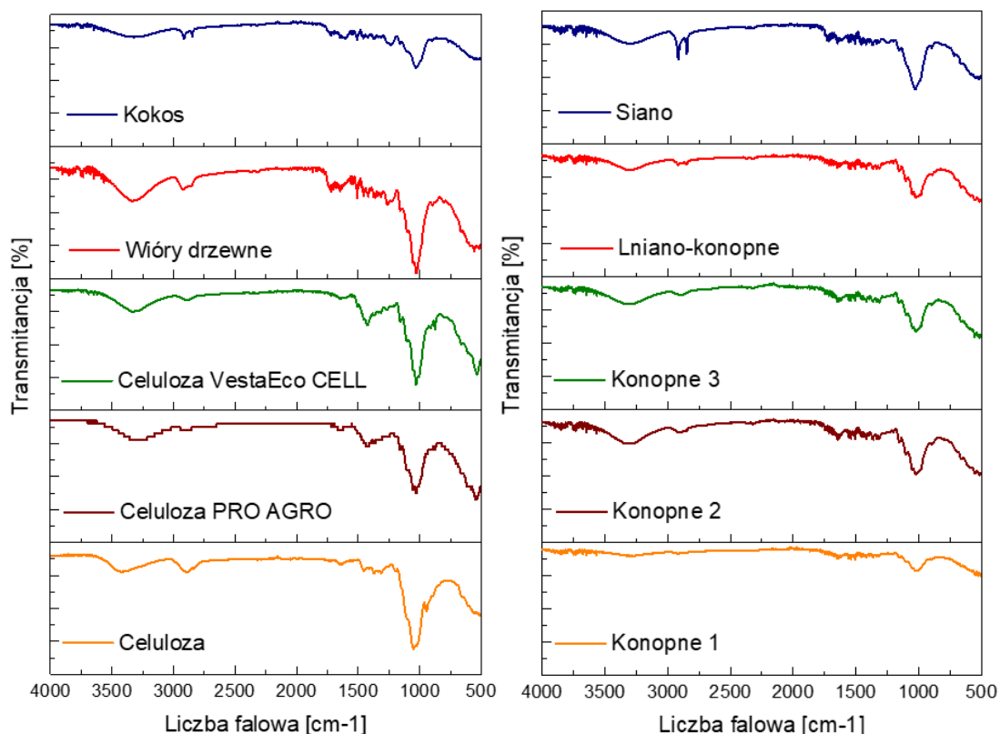
Rysunek 16. Widma FT-IR badanych włókien naturalnych.
