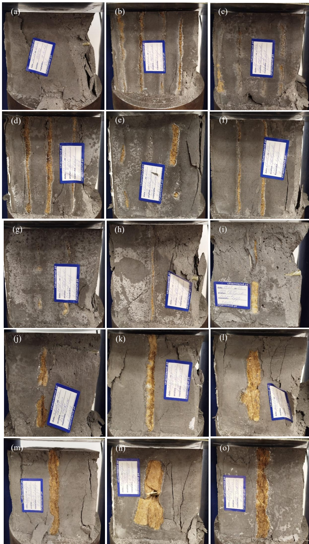
Rysunek 30. Makrofotografie kompozytów geopolimerowych po ściskaniu: a) RKG, b) K4M-8P-R, c) K4MP-8P-R, d) K3M-6P-R, e) K3MP-6P-R, f) K2M-4P-R, g) K2MP-4P-R, h) K1M-2P-R, i) K1MP-2P-R, j) K2MP-2P-Ś, k) K2M-2P-Ś, l) K3MP-2P-Ś, m) K3M-2P-Ś, n) K4MP-2P-Ś, o) K4M-2P-Ś.
