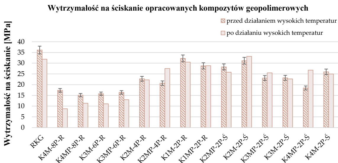
Rysunek 40. Porównanie wytrzymałości na ściskanie przed i po oddziaływaniu wysokich temperatur.
