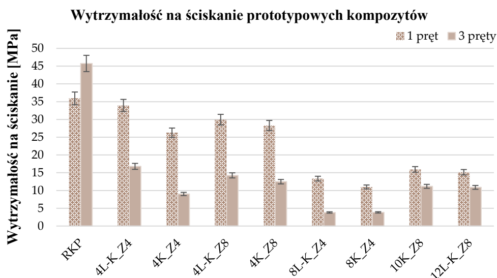
Rysunek 26. Porównanie wytrzymałości na ściskanie prototypowych kompozytów z różnym układem zbrojenia.
