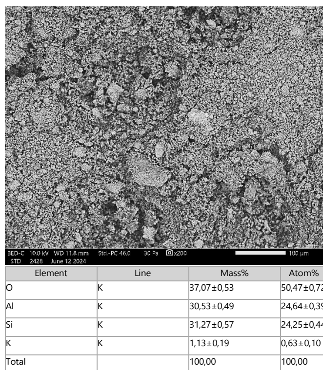
Rysunek 12. Morfologia metakaolinu wraz z analizą składu pierwiastkowego metodą EDS.
