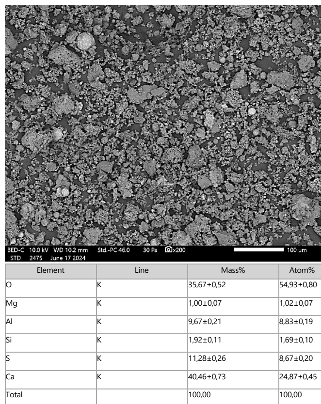
Rysunek 10. Morfologia popiołu lotnego ze spalania węgla brunatnego wraz z analizą składu pierwiastkowego metodą EDS.
