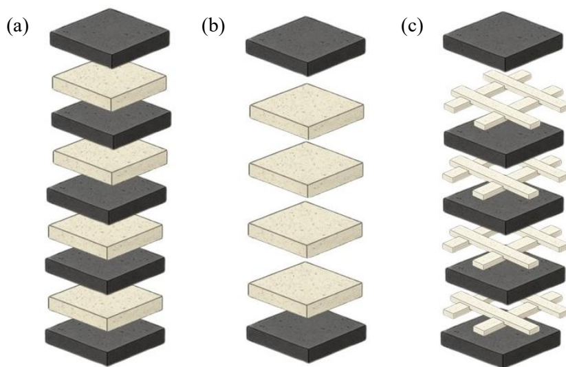
Rysunek 27. Schemat układu warstw w opracowanych kompozytach warstwowych: a) układ naprzemienny geopolimer-izolacja, b) układ z warstwą izolacyjną skoncentrowaną w środkowej części próbki, c) układ naprzemienny z warstwami izolacyjnymi ułożonymi krzyżowo.
