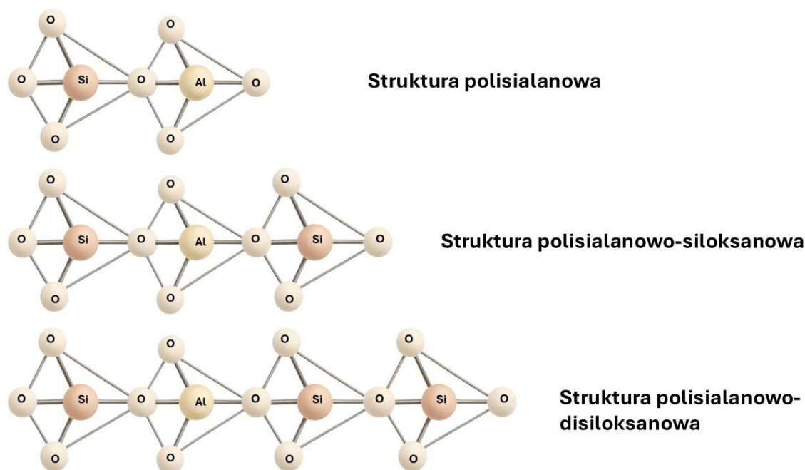
Rysunek 1. Schematyczne przedstawienie jednostek tetraedrycznych [\text{SiO}_4] i [\text{AlO}_4] oraz sposobu ich łączenia w sieć glinokrzemianową w zależności od stosunku Si/Al (na podstawie [14]).
