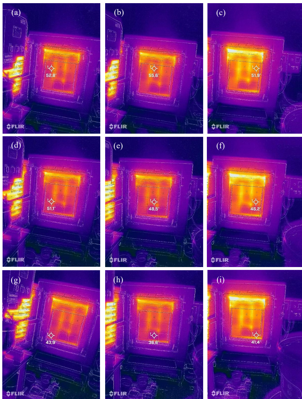
Rysunek 34. Analiza zachowania materiałów w warunkach oddziaływania temperatury 400°C: a) K2MP-4P-R, b) K1M-2P-R, c) K1MP-2P-R, d) K3M-6P-R, e) K3MP-6P-R, f) K2M-4P-R, g) RKG, h) K4M-8P-R, i) K4MP-8P-R.
