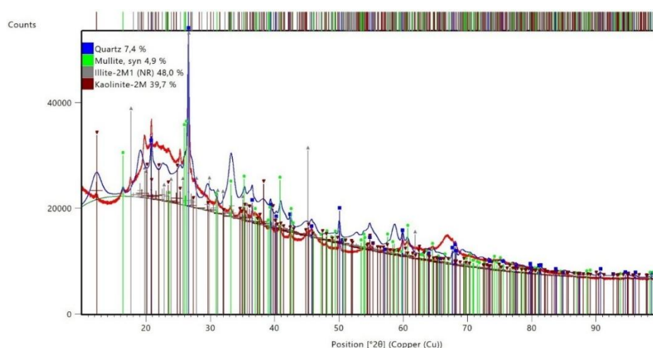
Rysunek 13. Dyfraktogram ilustrujący skład fazowy metakaolinu.
