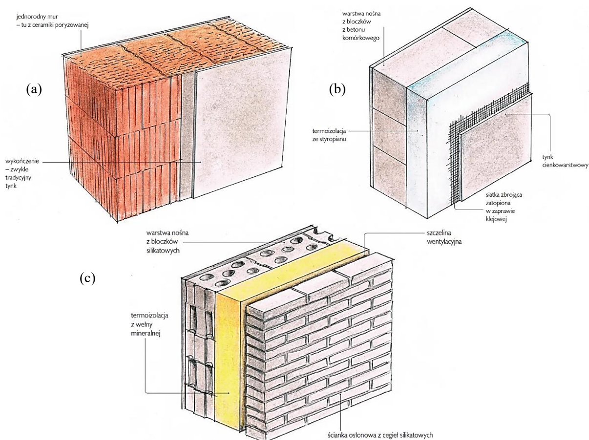
Rysunek 4. Schematy konstrukcyjne zewnętrznych ścian budynku: (a) ściana jednowarstwowa, (b) ściana dwuwarstwowa, (c) ściana trójwarstwowa [65].
