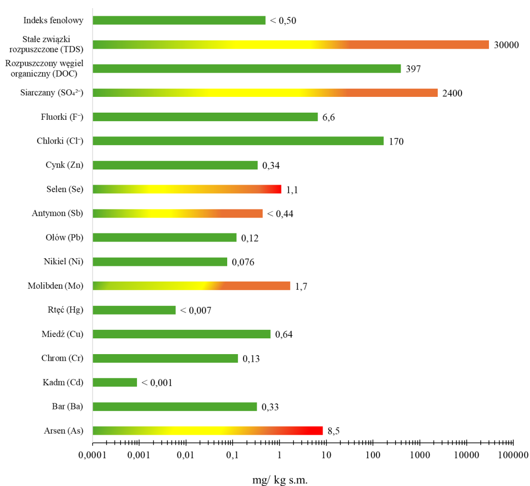
Rysunek 42. Wymywalność metali ciężkich i zanieczyszczeń w materiale geopolimerowym.
