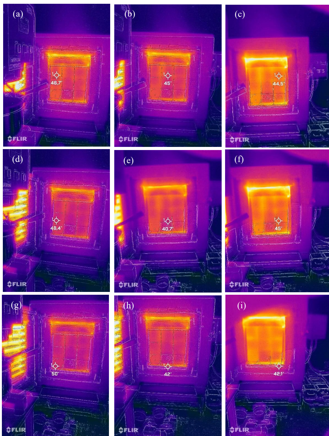
Rysunek 37. Analiza zachowania materiałów w warunkach oddziaływania temperatury 400°C: a) K3M-2P-Ś, b) K4MP-2P-Ś, c) K4M-2P-Ś, d) K2MP-2P-Ś, e) K2M-2P-Ś, f) K3MP-2P-Ś, g) K1MP- 2P-R, h) K4M-8P-R, i) K4MP-8P-R.
