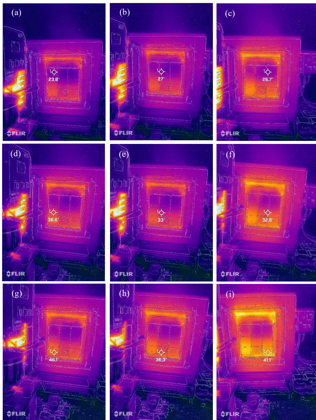
Rysunek 36. Analiza zachowania materiałów w warunkach oddziaływania temperatury 100°C: a) K3M-2P-Ś, b) K4MP-2P-Ś, c) K4M-2P-Ś, d) K2MP-2P-Ś, e) K2M-2P-Ś, f) K3MP-2P-Ś, g) K1MP- 2P-R, h) K4M-8P-R, i) K4MP-8P-R.
