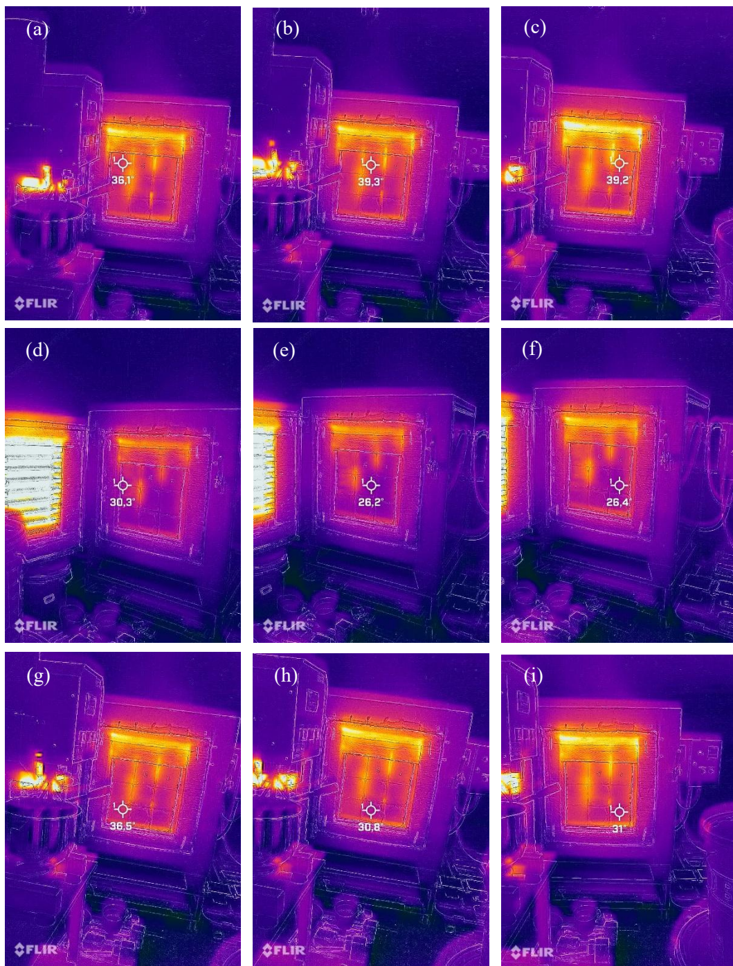
Rysunek 33. Analiza zachowania materiałów w warunkach oddziaływania temperatury 100°C: a) K2MP-4P-R, b) K1M-2P-R, c) K1MP-2P-R, d) K3M-6P-R, e) K3MP-6P-R, f) K2M-4P-R, g) RKG, h) K4M-8P-R, i) K4MP-8P-R.
