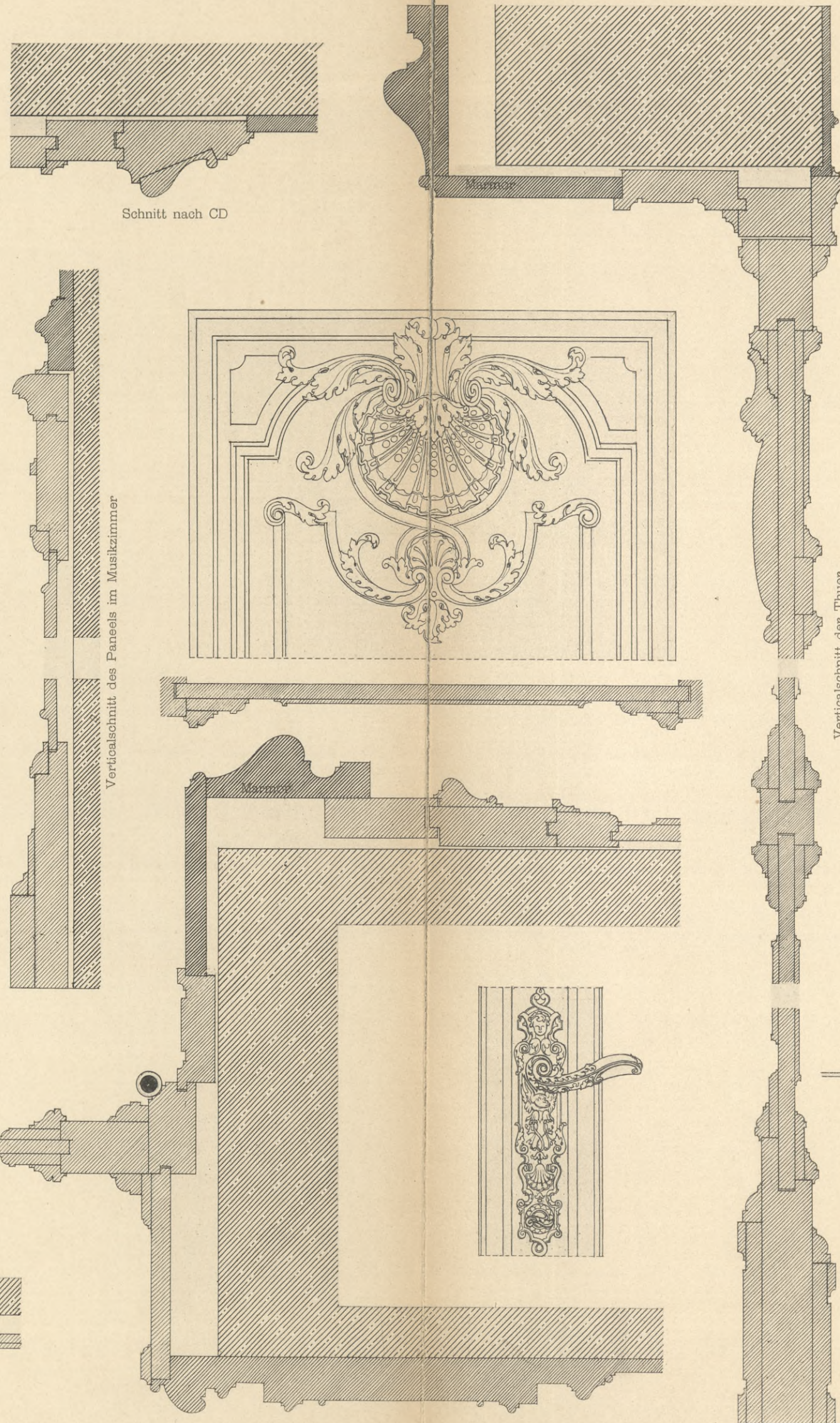
Horizontalschnitt der Thuer
