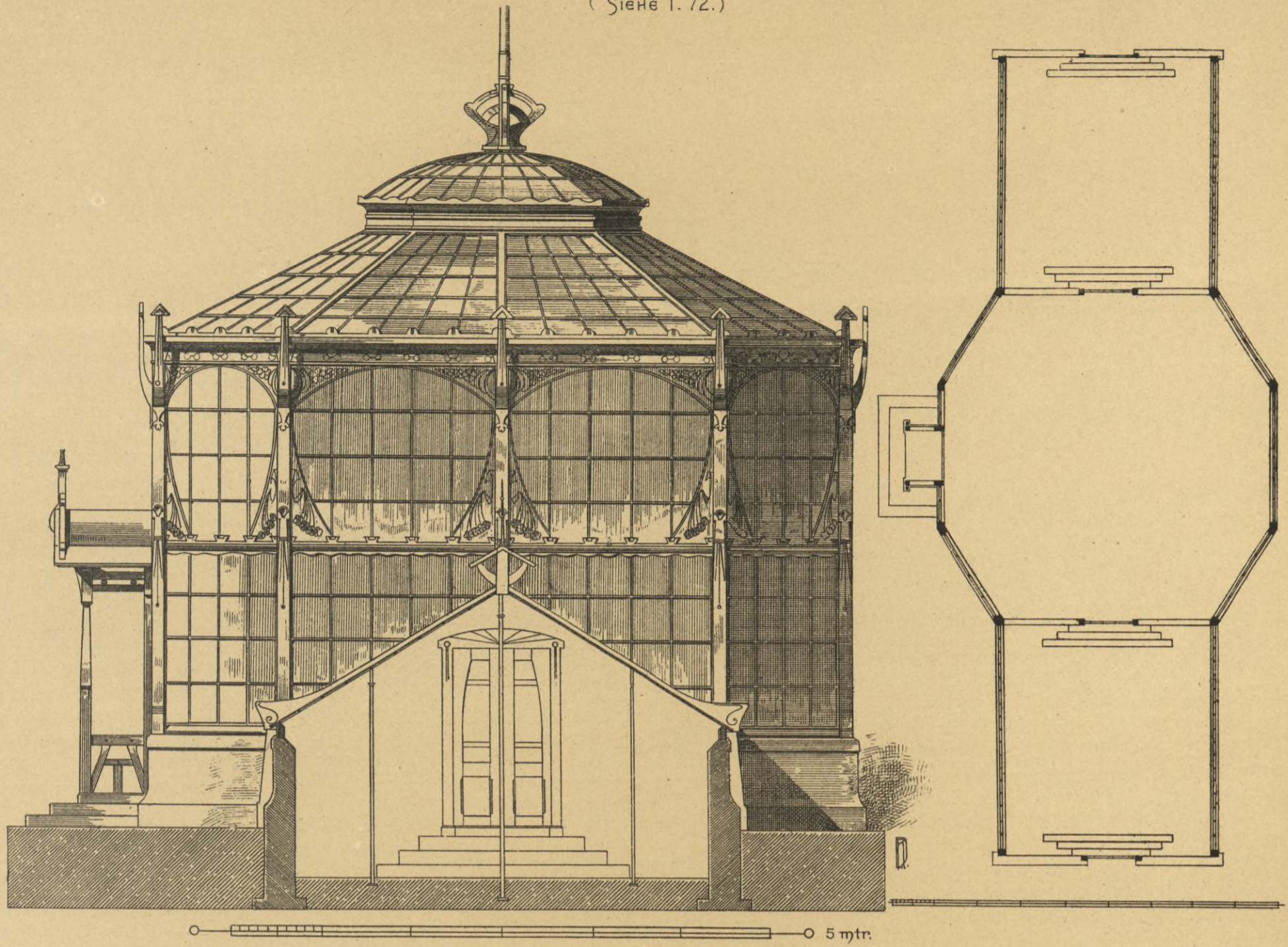
PALMEN- & GEWÄCHSHAUS. SEITENANSICHT.
