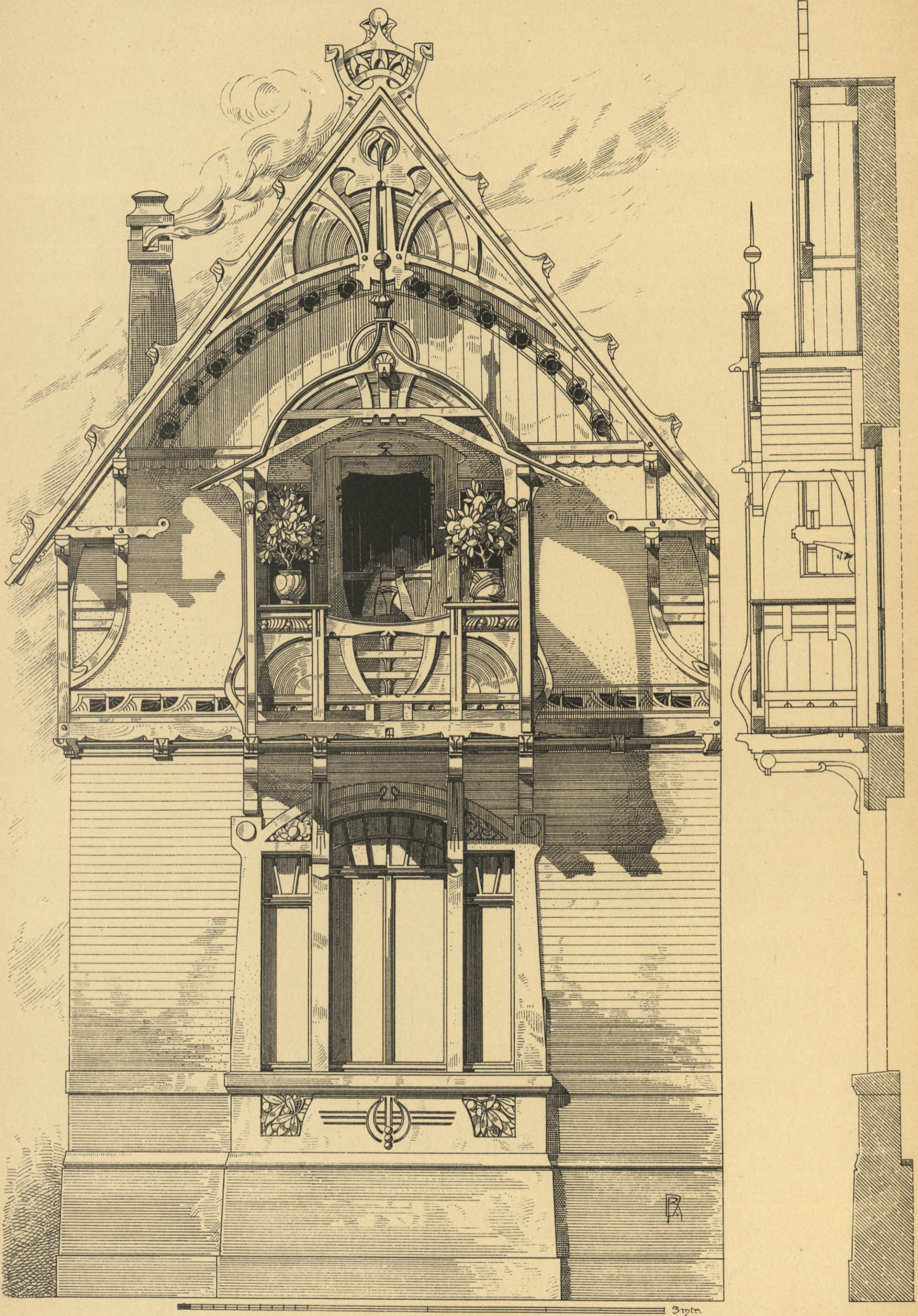
GIEBEL MIT BALKON.
