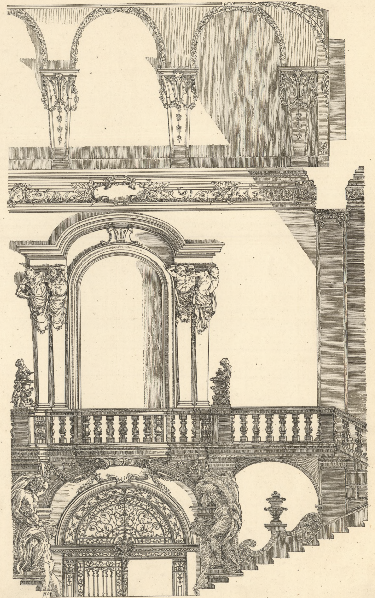
SCHNITT A-B GEGEN DEN EINGANG GESEHEN.
